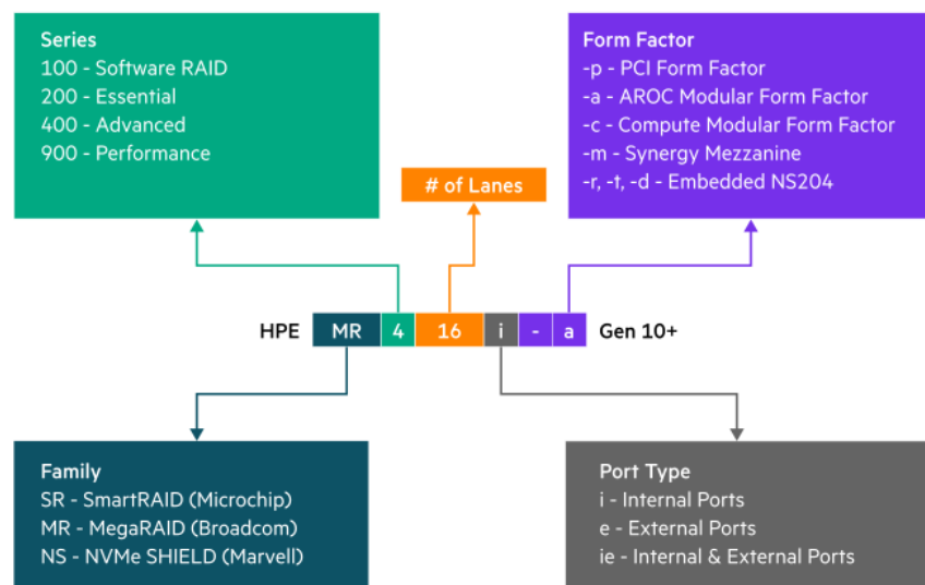
図 1. HPE MR Gen10 Plusコントローラーの命名フレームワーク
