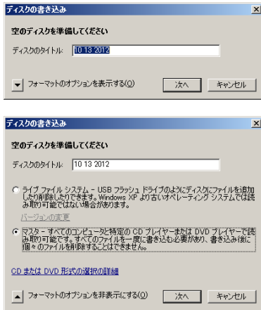
Win2008 の表示
