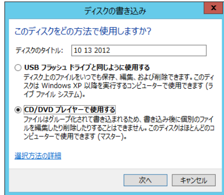
Win2012 の表示
