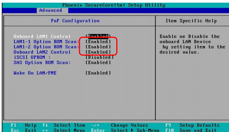
図 4-10 BIOS 設定画面([PnP Configuration]の確認)
