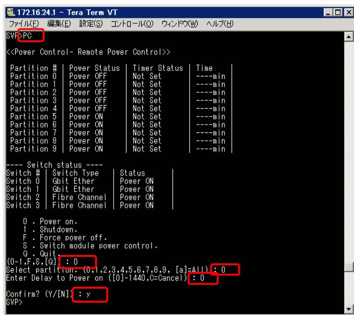
図 4-5 ブレード電源 ON
