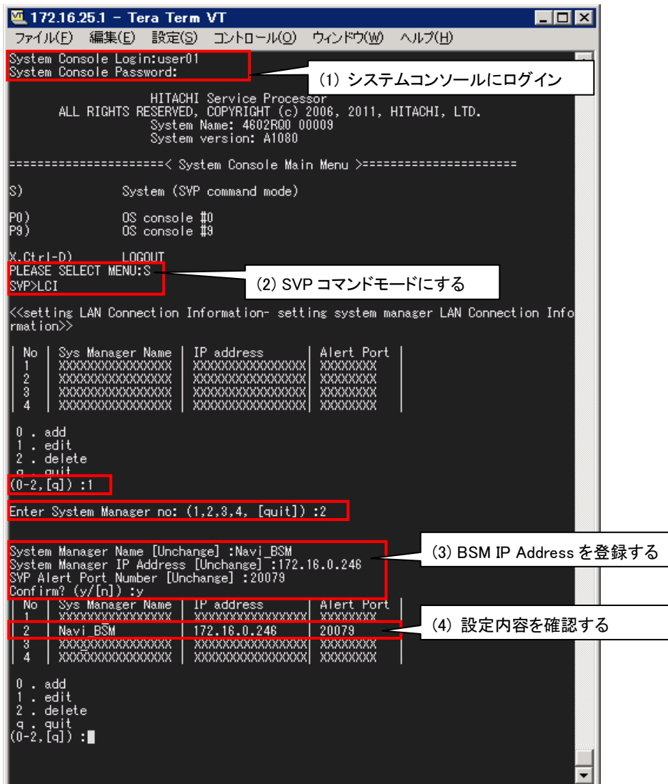
図 4-2 システムコンソール(BSM IP Address の設定)
