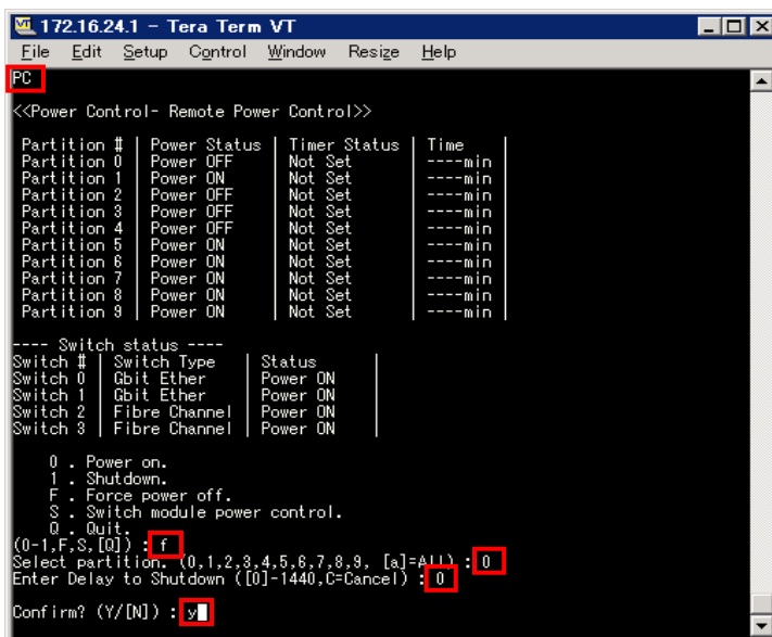
図 4-14 ブレード電源 OFF
