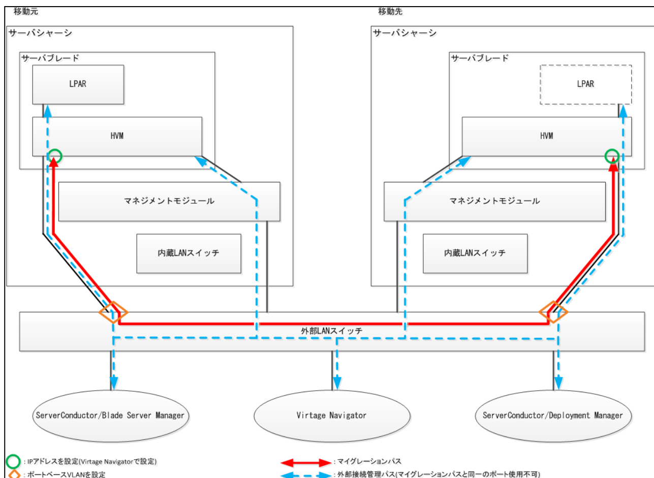
図 2-9 ネットワークの推奨構成
