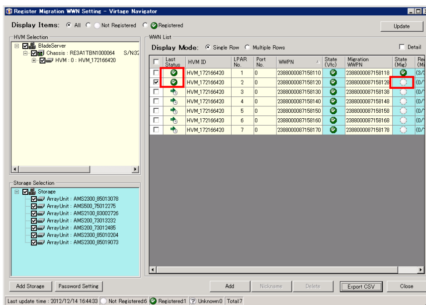
図 3-148 Register Migration WWN Setting ウィンドウ (マイグレーション WWPN 削除結果の確認)
