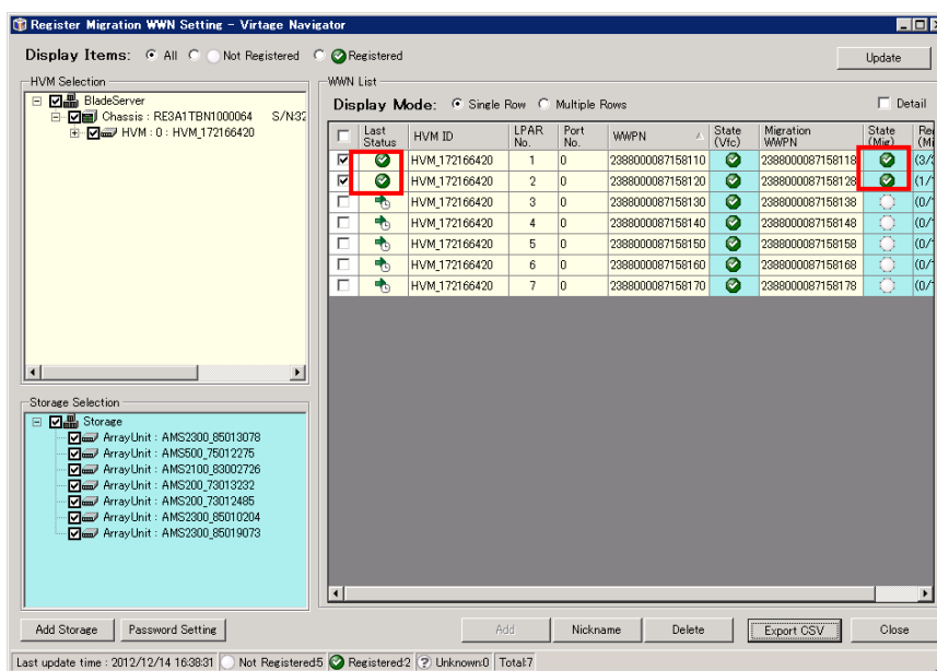
図 3-143 Register Migration WPN Setting ウィンドウ (マイグレーション WPN 登録結果の確認)
