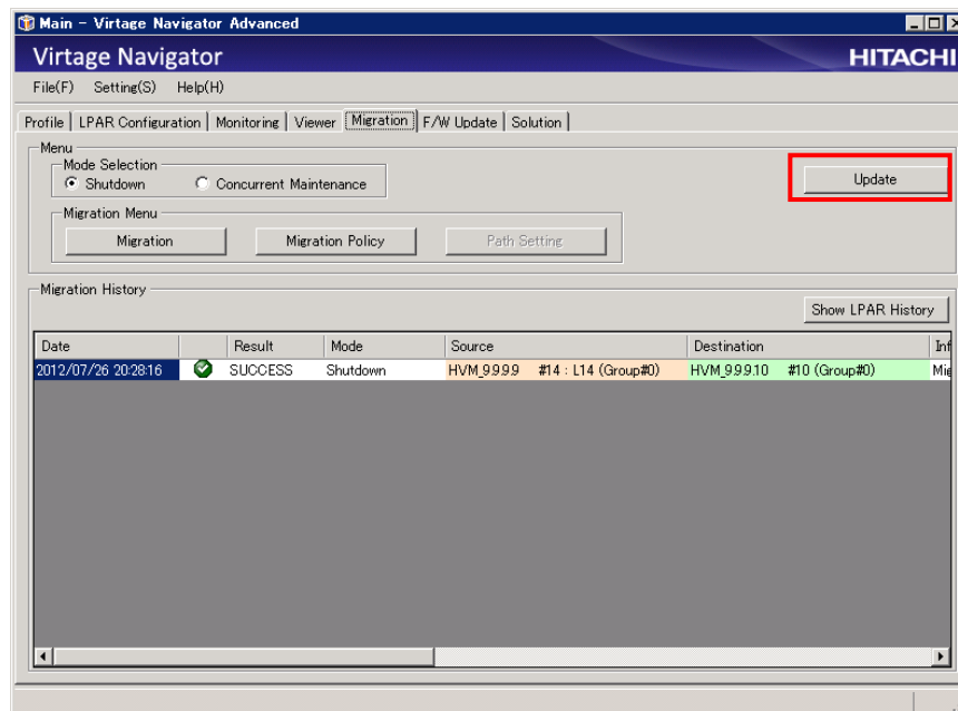
図 3-17 Main ウィンドウ (Update 操作)
