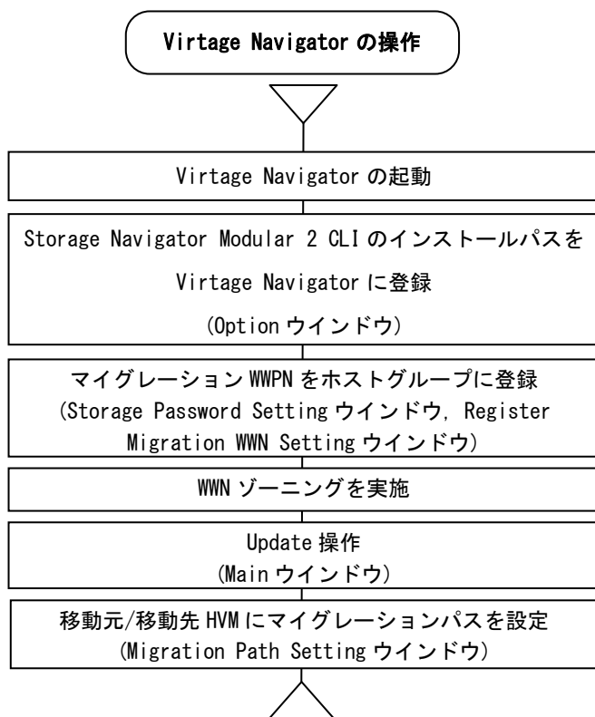
図 3-23 コンカレントメンテナンスモードの LPAR マイグレーションの設定フロー
