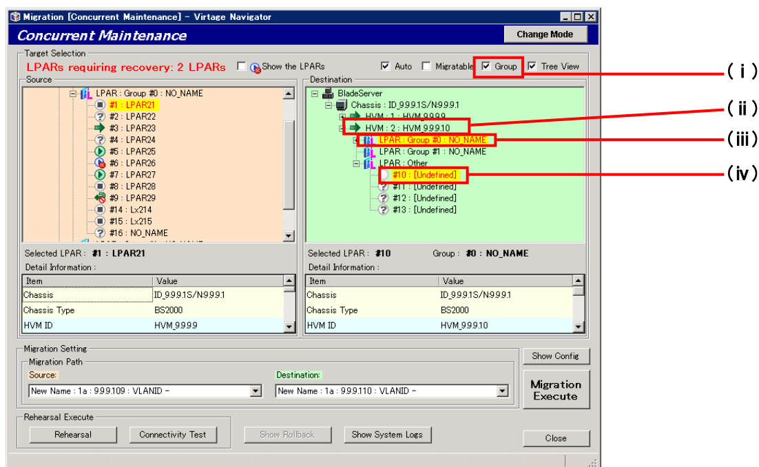
図 3-46 Migration[Concurrent Maintenance] ウィンドウ (プロセッサグループ指定)
