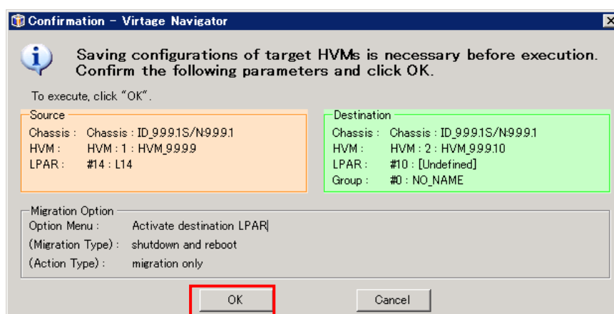
図 3-11 Confirmation ウインドウ(シャットダウンモードの LPAR マイグレーション実施)
