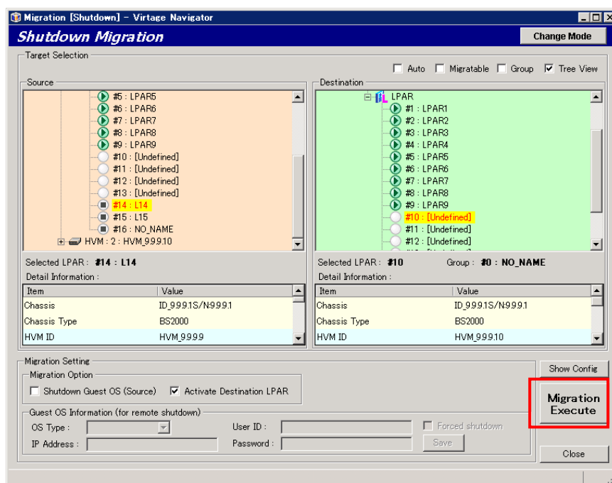
図 3-10 Migration[Shutdown]ウインドウ(シャットダウンモードの LPAR マイグレーションの実施)
