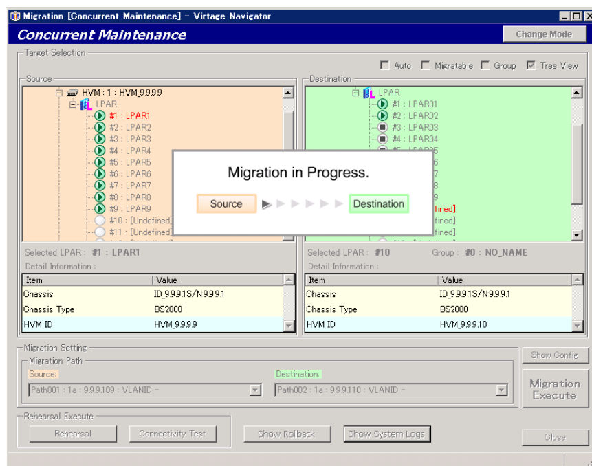
図 3-53 Migration[Concurrent Maintenance] ウィンドウ(コンカレントメンテナンスモードの LPAR マイグレーション実施中)
