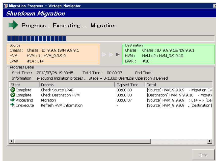
図 3-13 Migration Progress ウィンドウ(シャットダウンモードの LPAR マイグレーション進行状況表示)
