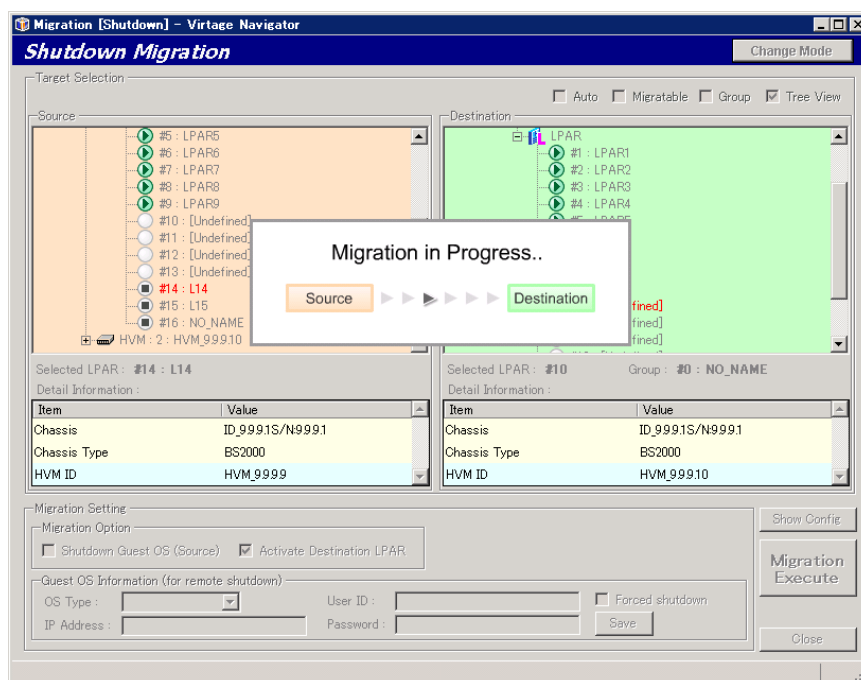
図 3-12 Migration[Shutdown] ウィンドウ(シャットダウンモードの LPAR マイグレーション実施中)
