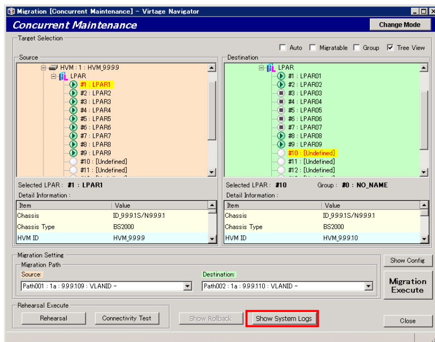
図 3-47 Migration[Concurrent Maintenance] ウィンドウ (Show System Logs クリック)
