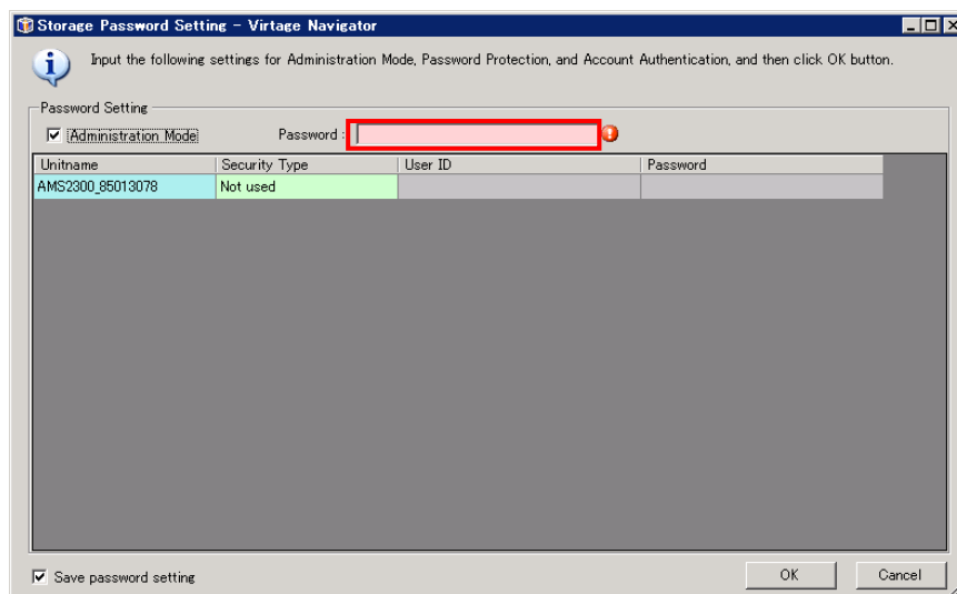
図 3-132 Storage Password Setting ウィンドウ (Administration Mode チェック)
