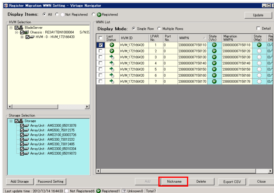
図 3-150 Register Migration WWN Setting ウィンドウ (Nickname クリック)
