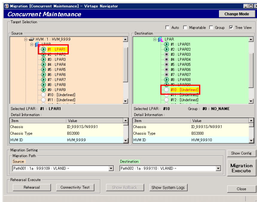
図 3-43 Migration[Concurrent Maintenance]ウインドウ(移動元/移動先 LPAR の選択)
