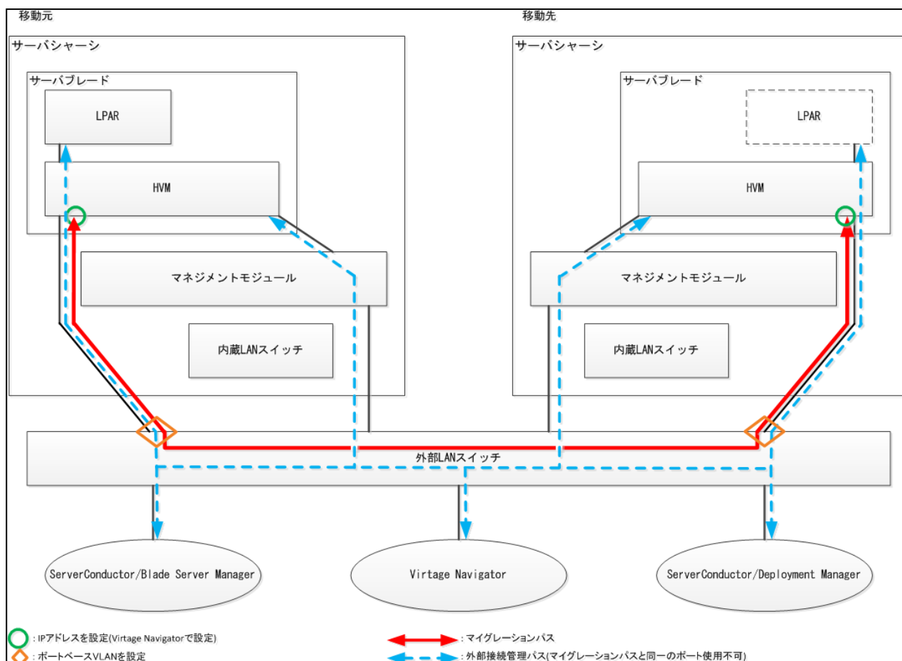
図 2-9 ネットワークの推奨構成 (PCI カードをマイグレーションパス専用を設定した場合)
