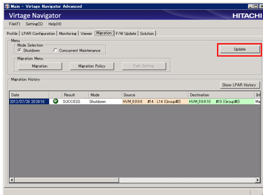
図 3-61 Main ウィンドウ (Update 操作)
