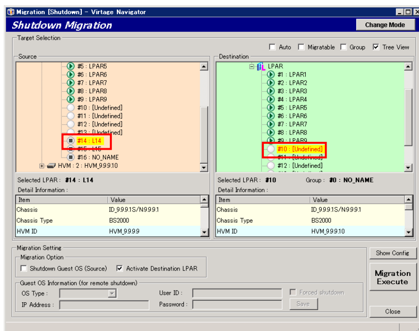
図 3-6 Migration[Shutdown] ウィンドウ (移動元/移動先 LPAR の選択)
