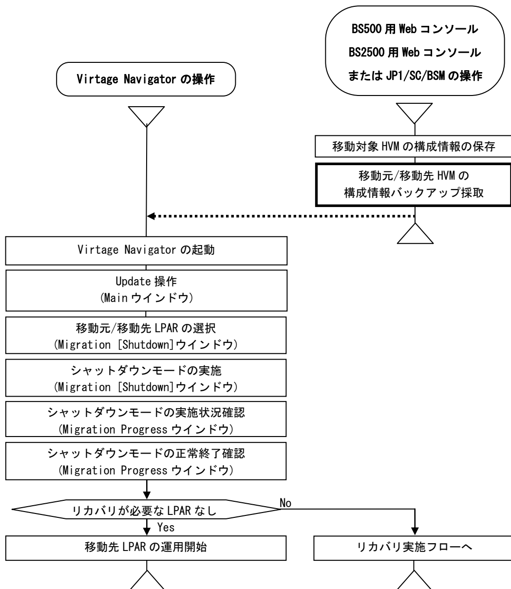
図 3-1 シャットダウンモードの LPAR マイグレーションの基本的な実施フロー
