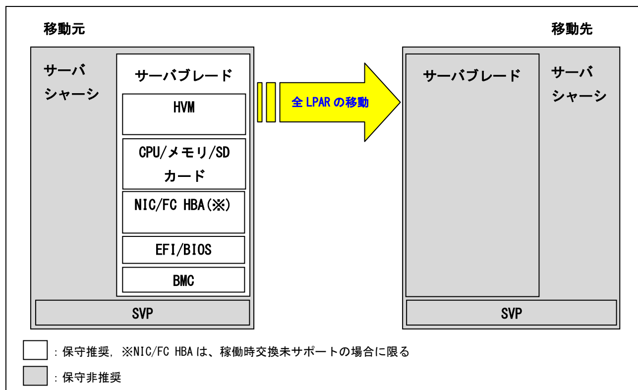
図 1-1 コンカレントメンテナンスモードの LPAR マイグレーションを利用した保守の種類
