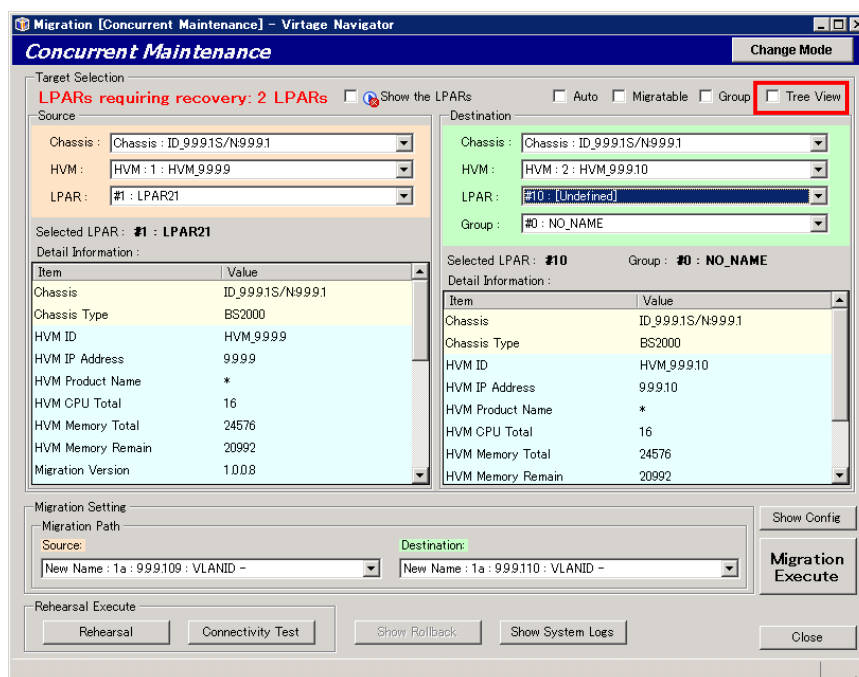
図 3-44 Migration[Concurrent Maintenance]ウインドウ(コンボボックスでの LPAR 選択)
