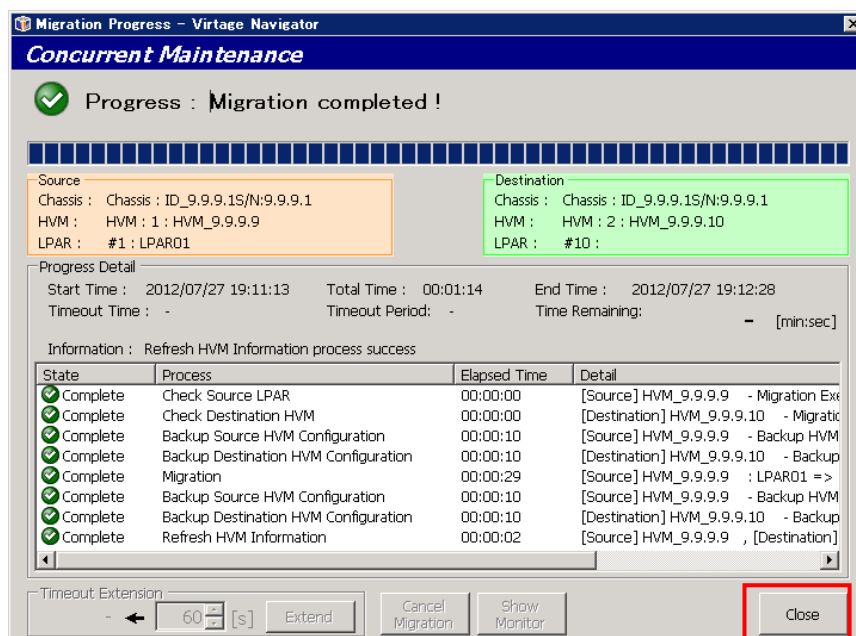
図 3-55 Migration Progress ウィンドウ (コンカレントメンテナンスモードの LPAR マイグレーション完了時)
