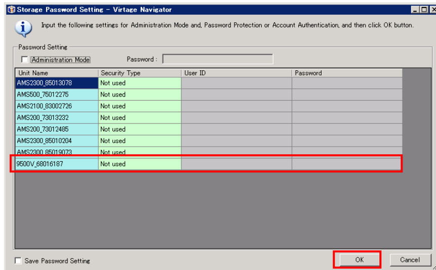
図 3-172 Configuration Registration ウィンドウ (Password Setting クリック)
