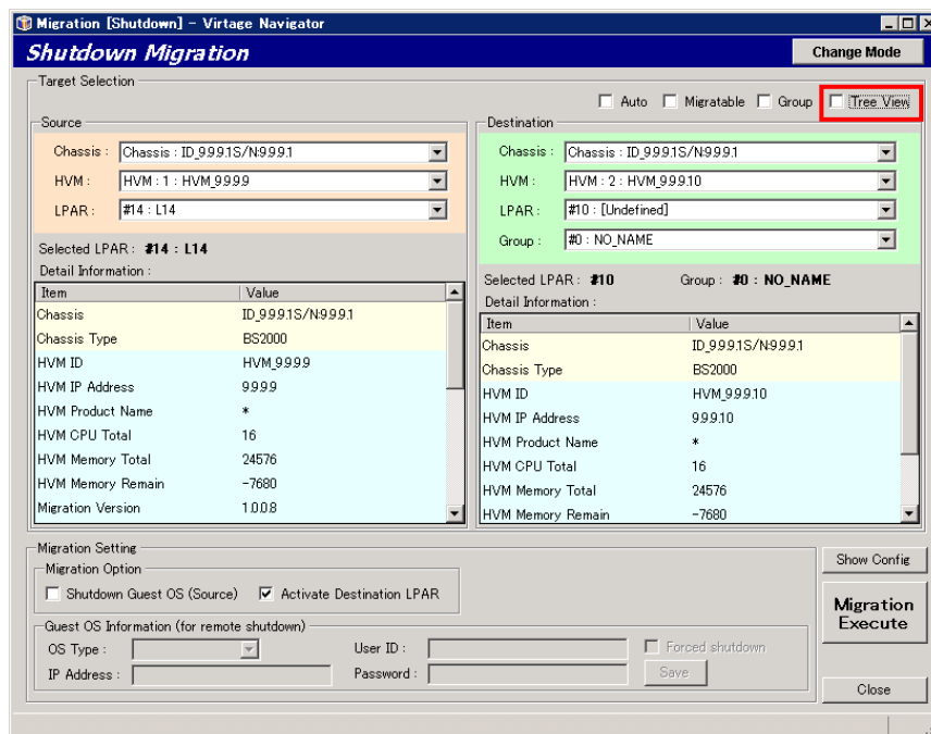
図 3-7 Migration[Shutdown] ウインドウ (コンボボックスでの LPAR 選択)
