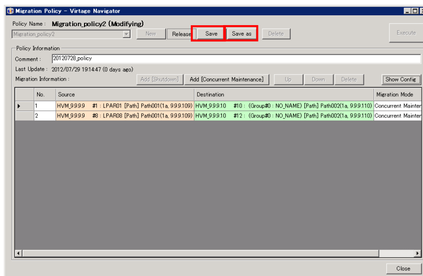
図 3-100 Migration Policy ウィンドウ (Migration Policy 保存)
