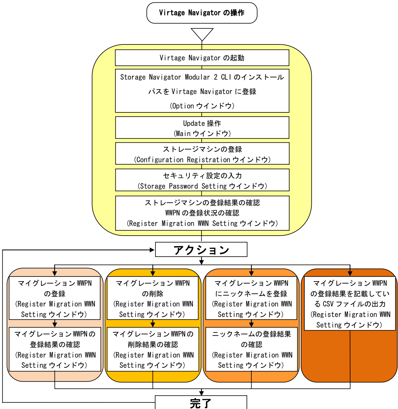
図 3-116 マイグレーション WPN 登録、削除フロー
