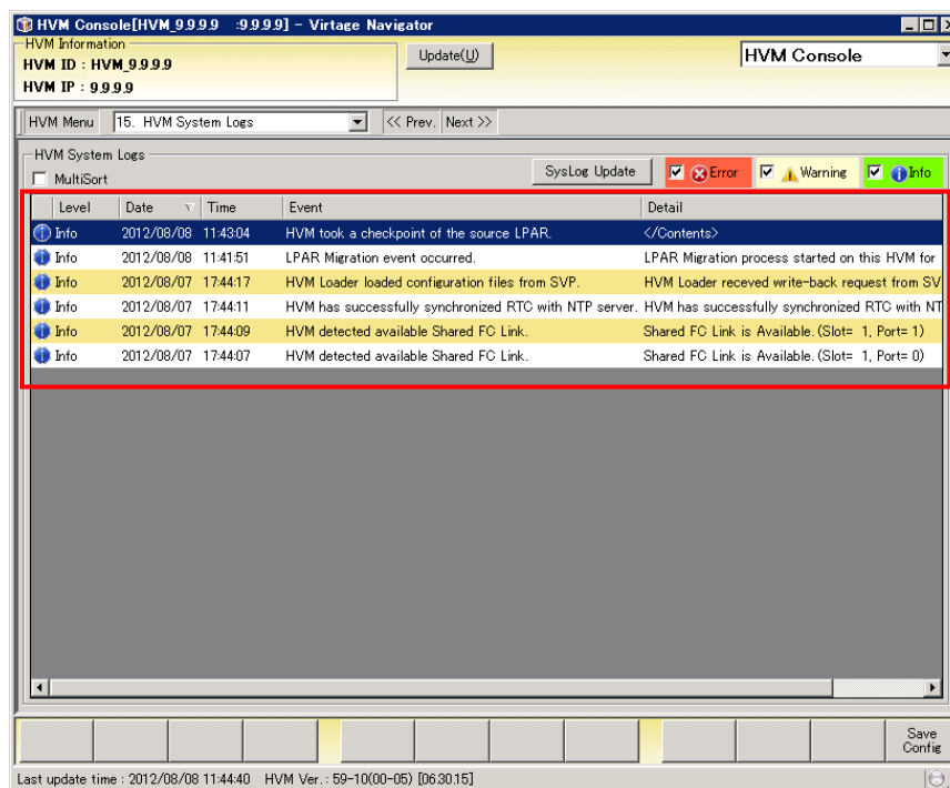
図 3-57 HVM Console ウィンドウ (移動元 HVM でエラーログがないことの確認)
