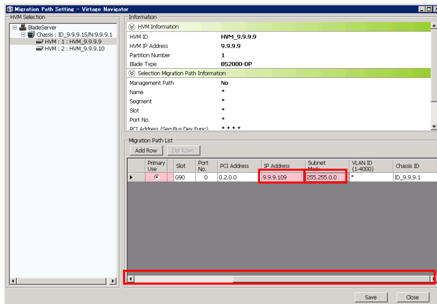
図 3-33 Main ウィンドウ (IP アドレスと Subnet Mask の設定)
