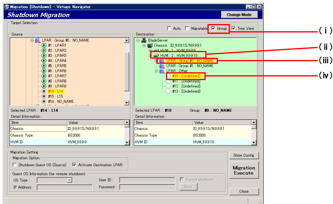
図 3-9 Migration[Shutdown] ウィンドウ (プロセッサグループ指定)
