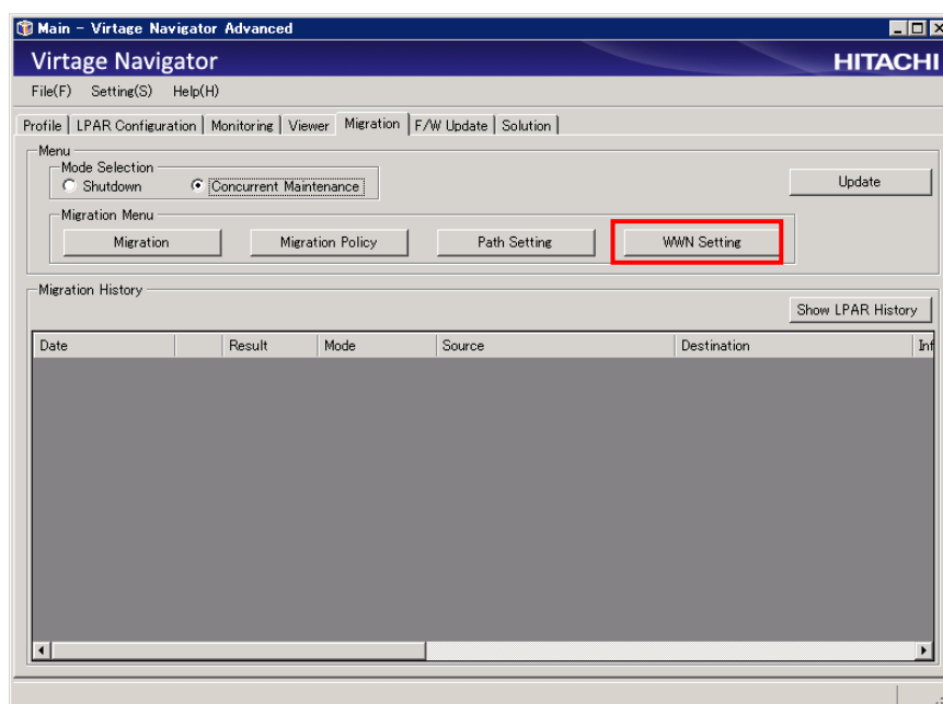
図 3-125 Main ウィンドウ (WWN Setting クリック)
