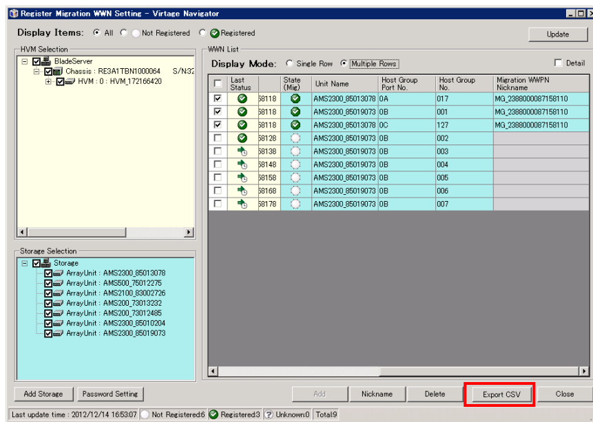
図 3-157 Register Migration WPN Setting ウィンドウ (Export CSV クリック)
