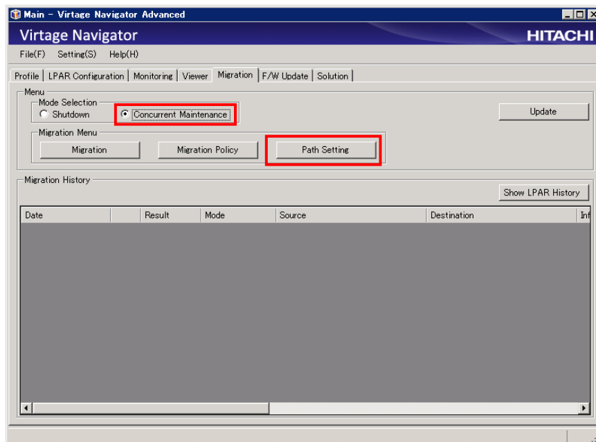
図 3-30 Main ウィンドウ (Path Setting クリック)
