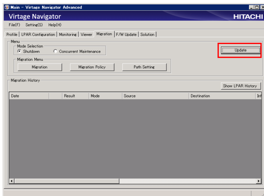
図 3-40 Main ウィンドウ (Update クリック)
