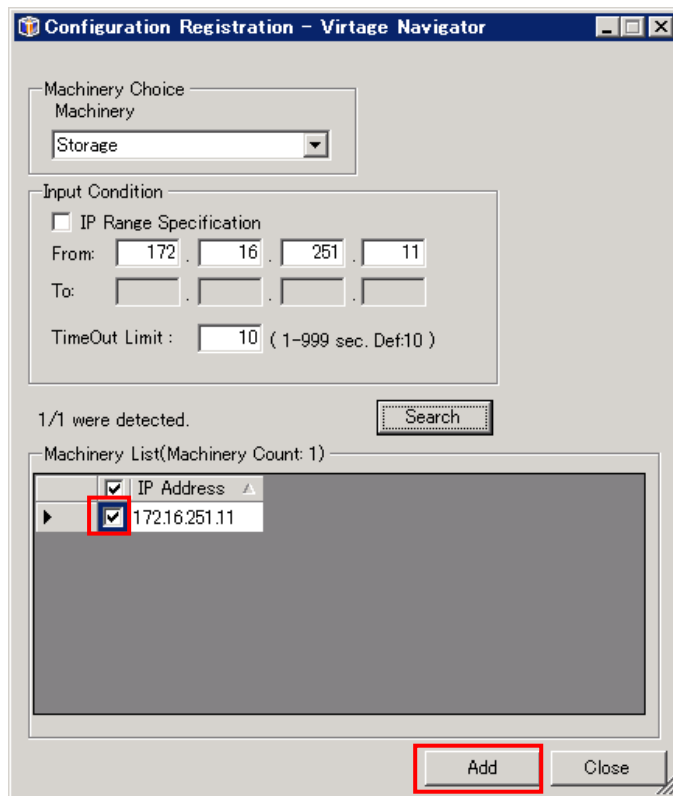
図 3-128 Configuration Registration ウィンドウ (Add クリック)
