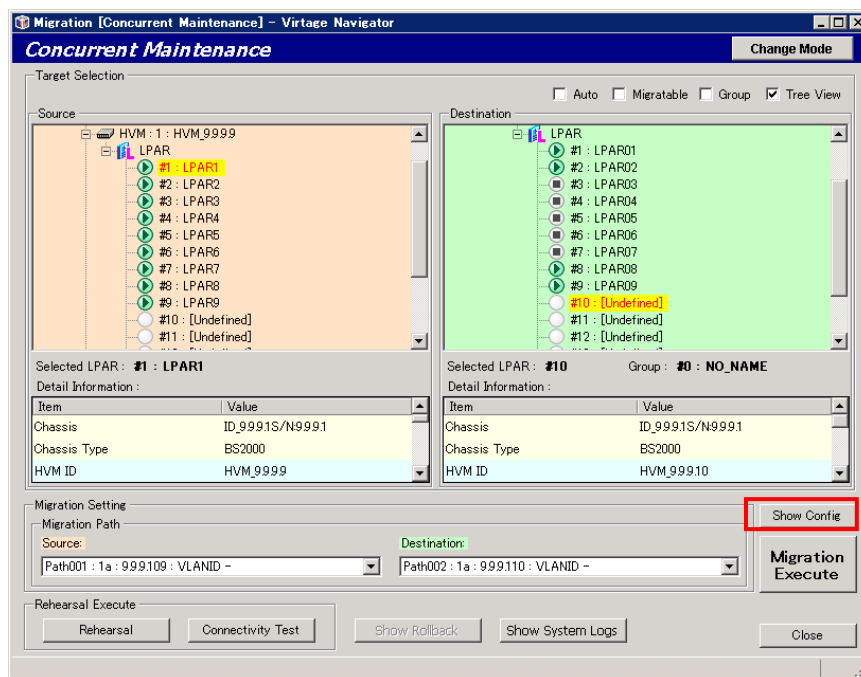
図 3-49 Migration [Concurrent Maintenance] ウィンドウ (Show Config クリック)
