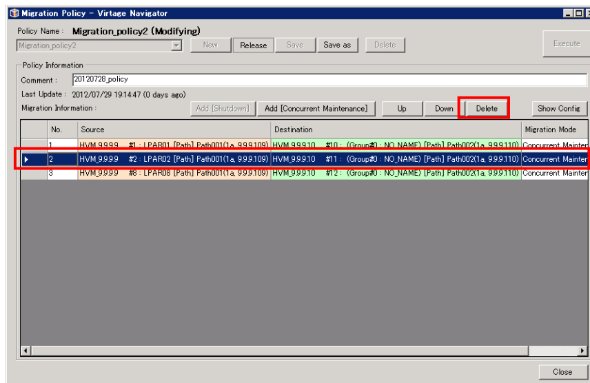
図 3-99 Migration Policy ウィンドウ (Migration Policy エントリの削除)
