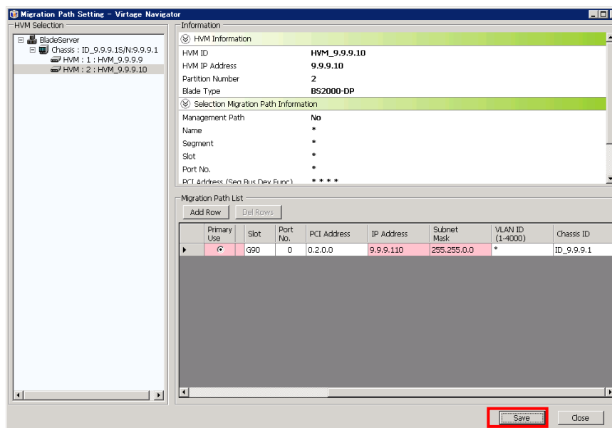
図 3-34 Main ウィンドウ (Save クリック)
