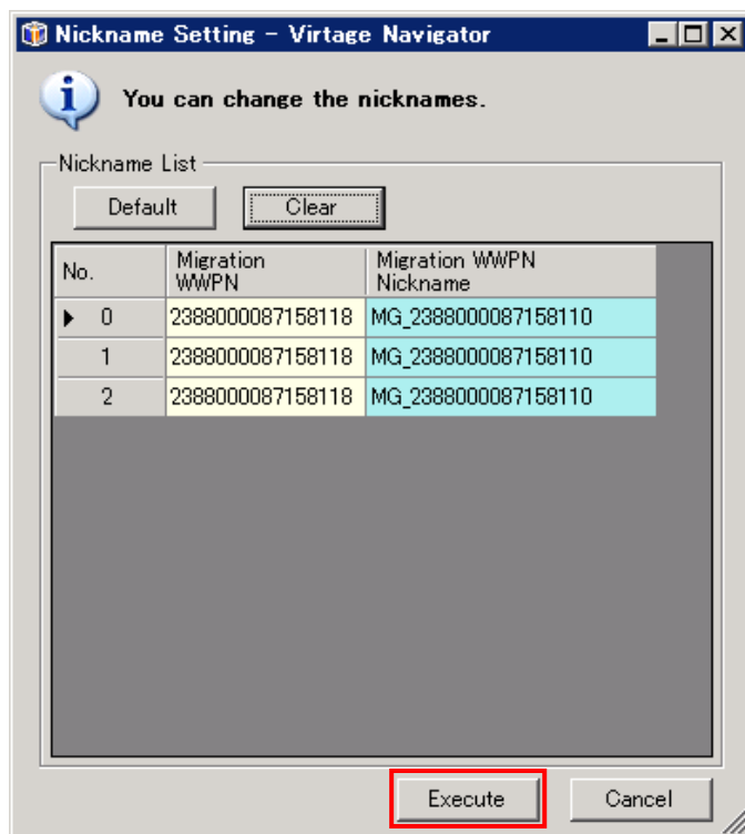
図 3-152 Nickname Setting ウィンドウ(Execute クリック)
