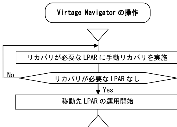
図 3-59 リカバリ実施フロー
