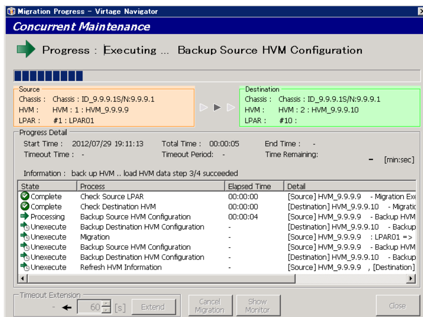
図 3-54 Migration Progress ウィンドウ(コンカレントメンテナンスモード進行状況表示)
