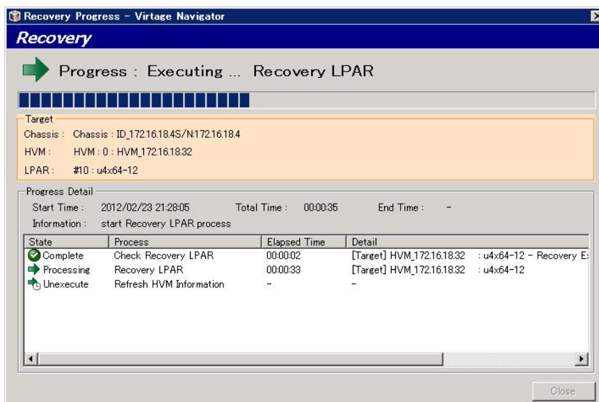
図 3-65 Recovery の Progress ウィンドウ (実施中)
