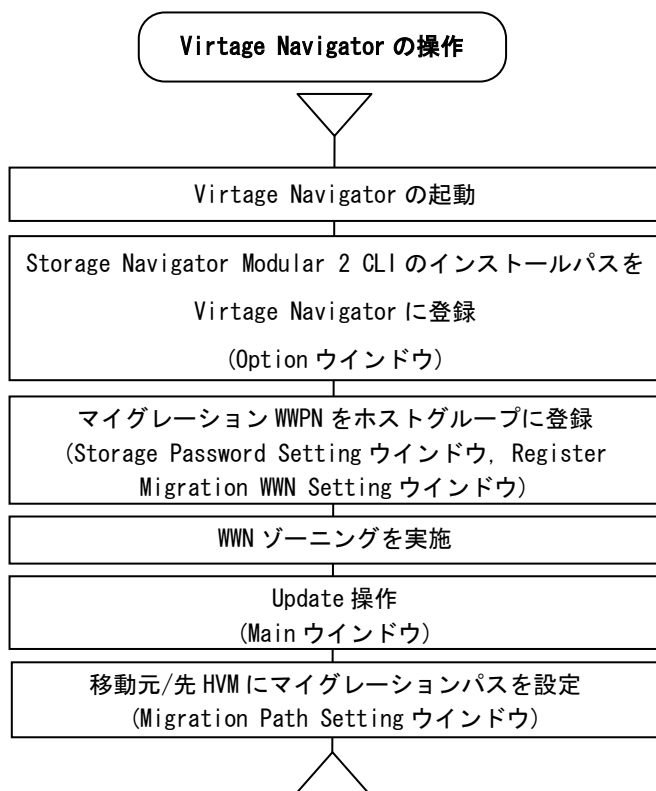
図 3-23 コンカレントメンテナンスモードの設定フロー
