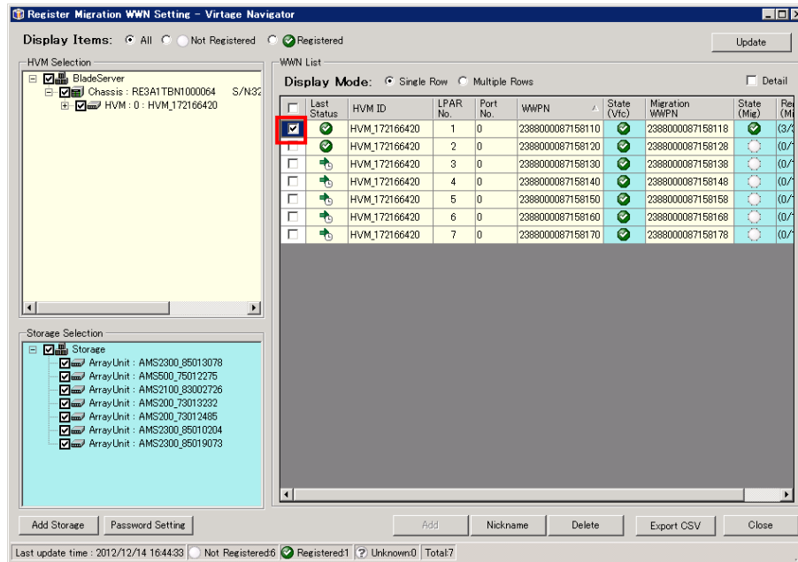
図 3-149 Register Migration WPN Setting ウィンドウ (マイグレーション WPN の選択)
