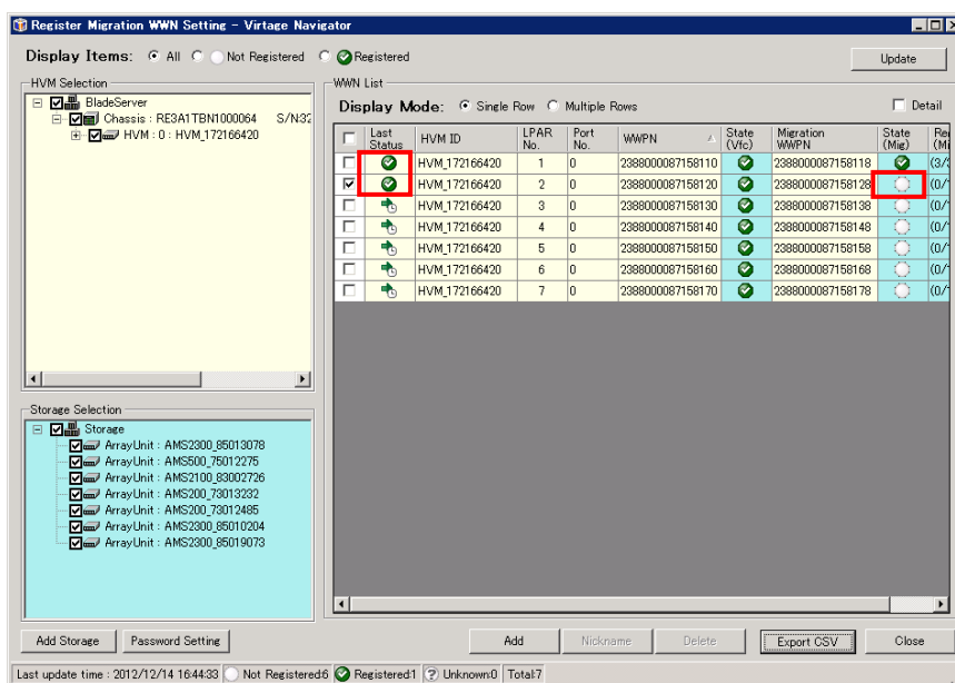
図 3-148 Register Migration WWN Setting ウィンドウ (マイグレーション WWP 削除結果の確認)
