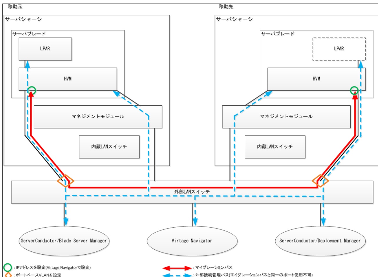
図 2-9 ネットワークの推奨構成
