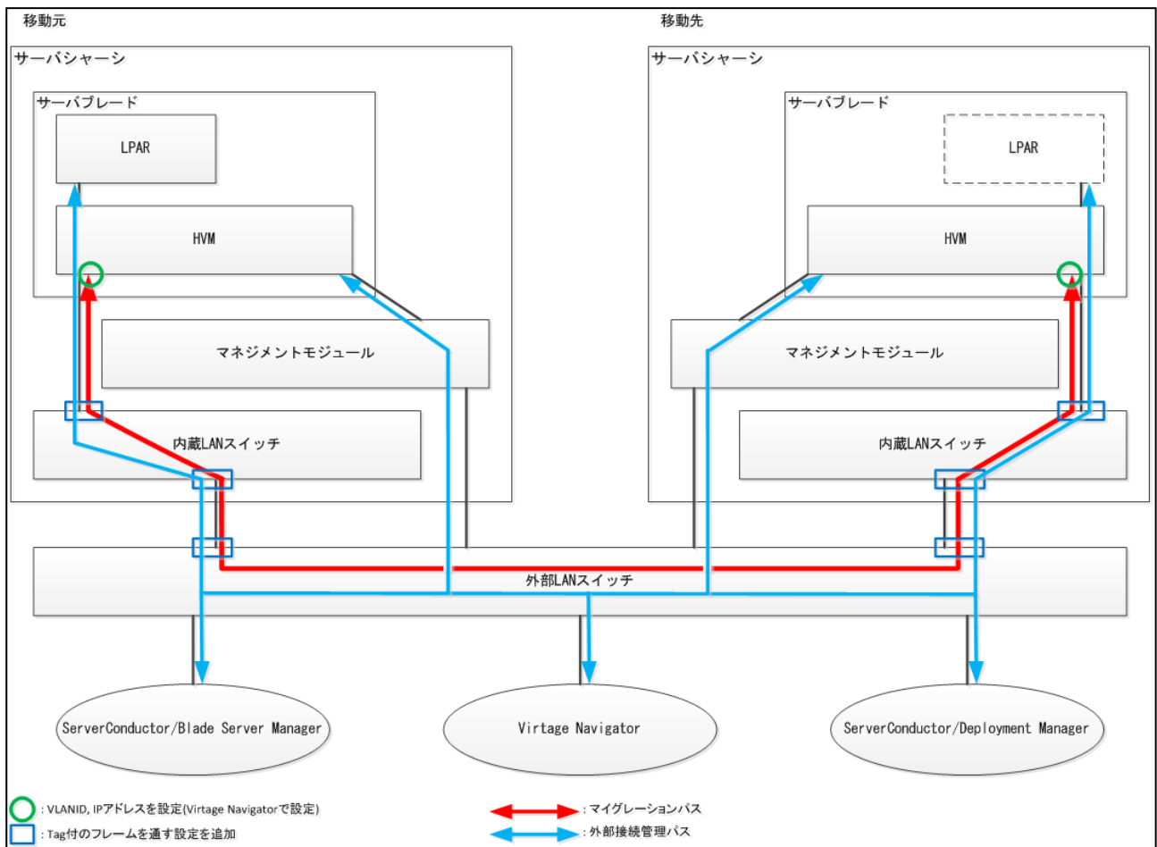
図 2-6 ネットワークの推奨構成
