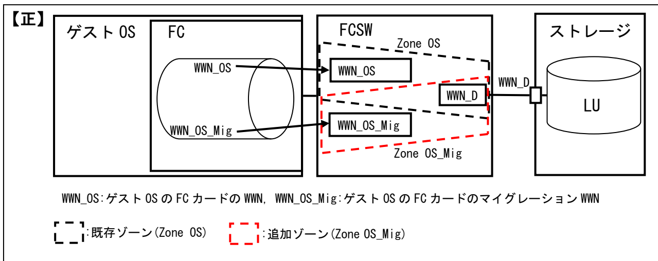
図 3-24 マイグレーション WWN を含むゾーニング構成 (正しい例)
