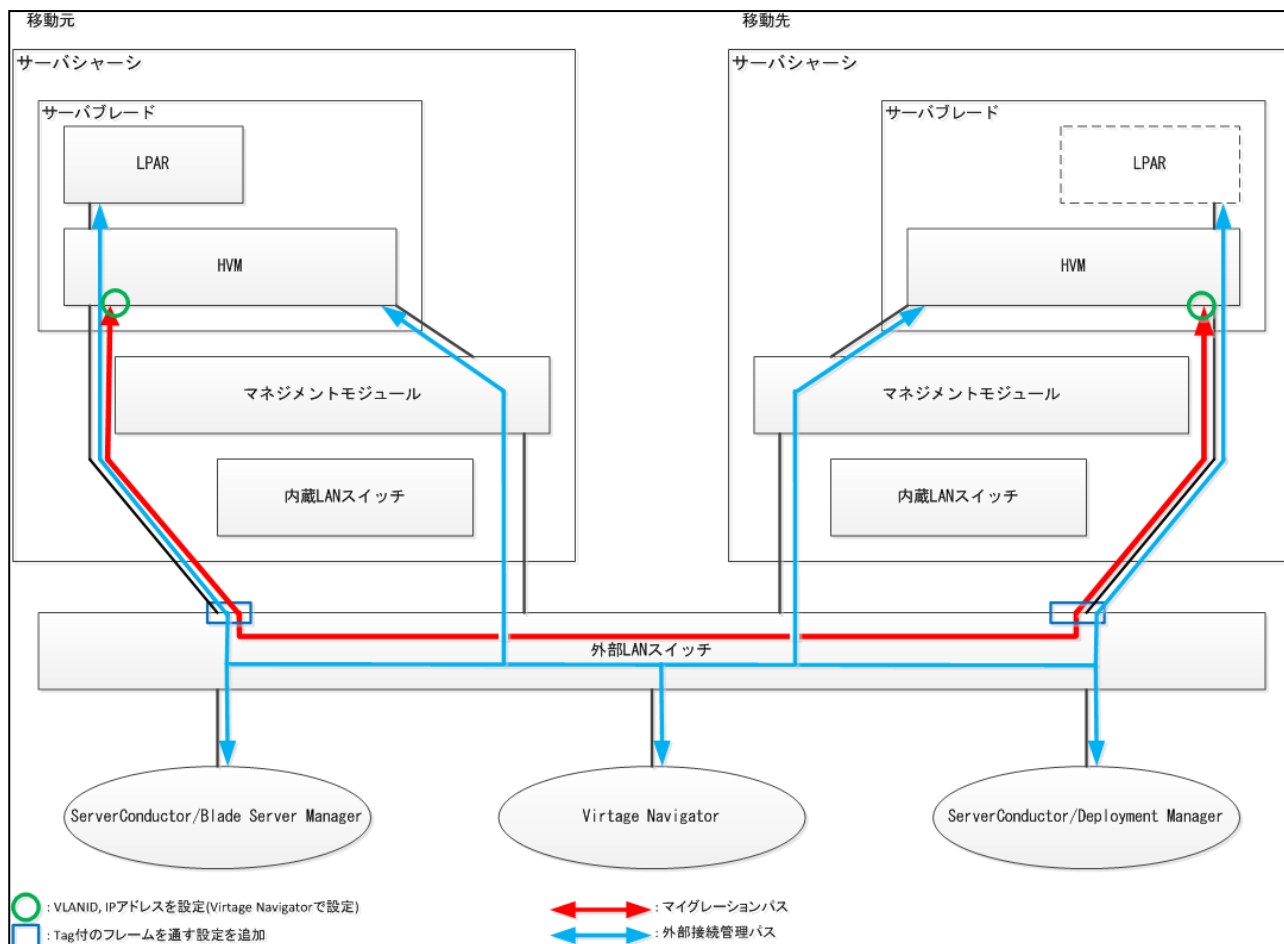
図 2-8 ネットワークの推奨構成 (PCI カードにマイグレーションパスを追加で設定した場合)
