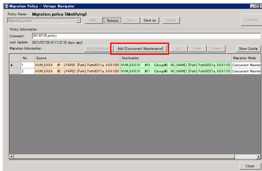
図 3-93 Migration Policy ウィンドウ (Migration Policy エントリの追加)
