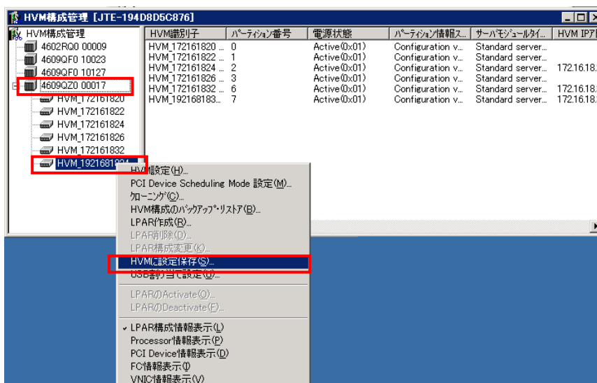
図 3-109 HVM 構成管理ウィンドウ (シャーシの選択)
