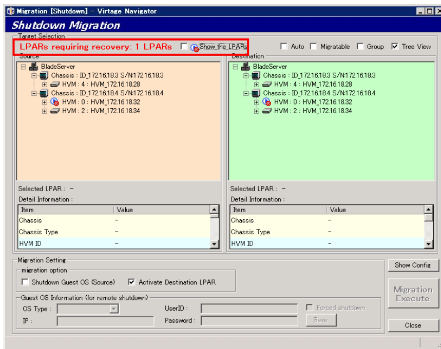
図 3-18 Migration[Concurrent Maintenance]ウィンドウ(手動リカバリ要 LPAR あり)
