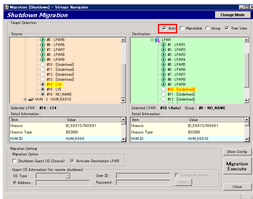
図 3-8 Migration[Shutdown]ウインドウ (移動先 LPAR の自動選択)
