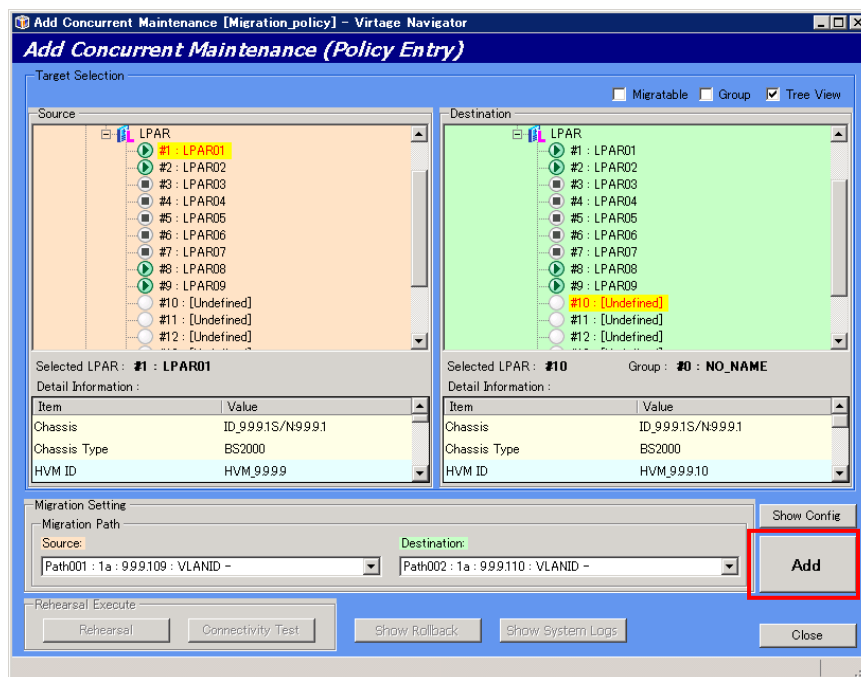
図 3-79 Add Concurrent Maintenance ウィンドウ (LPAR 選択操作)
