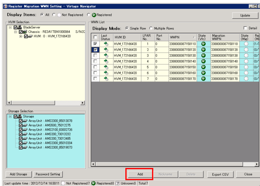
図 3-140 Register Migration WPN Setting ウィンドウ(Add クリック)
