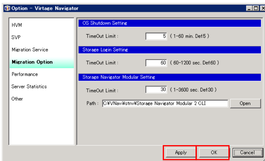
図 3-121 Option ウィンドウ (Storage Navigator Modular 2 CLI フォルダの選択)
