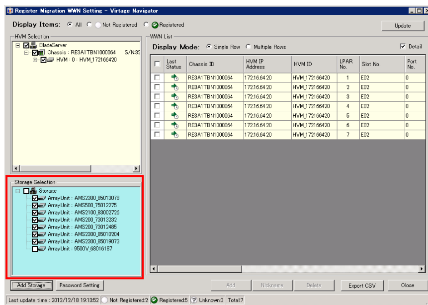
図 3-170 Configuration Registration ウィンドウ (OK クリック)
