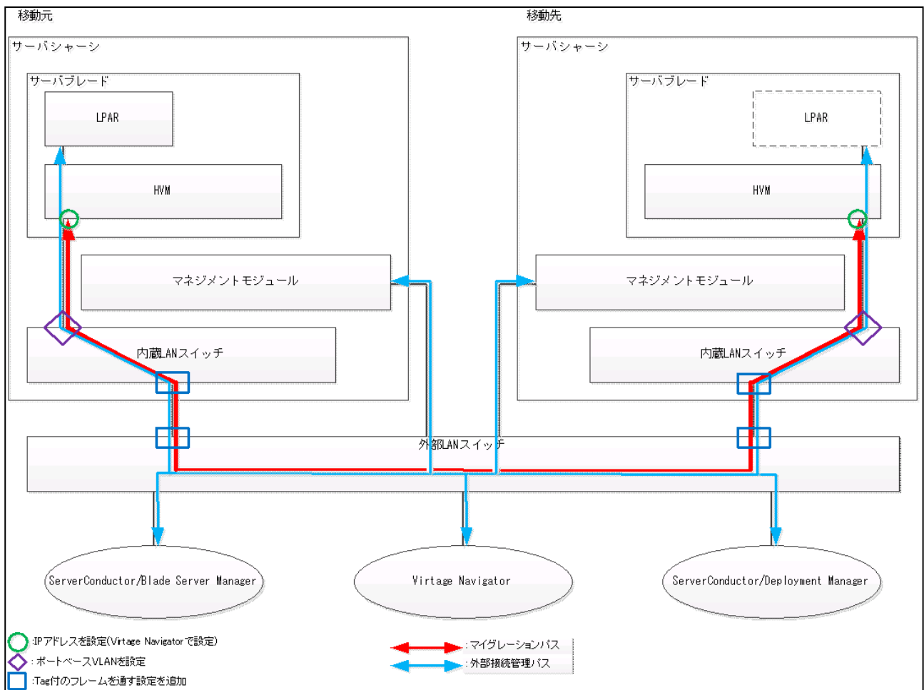
図 2-9 ネットワークの推奨構成
