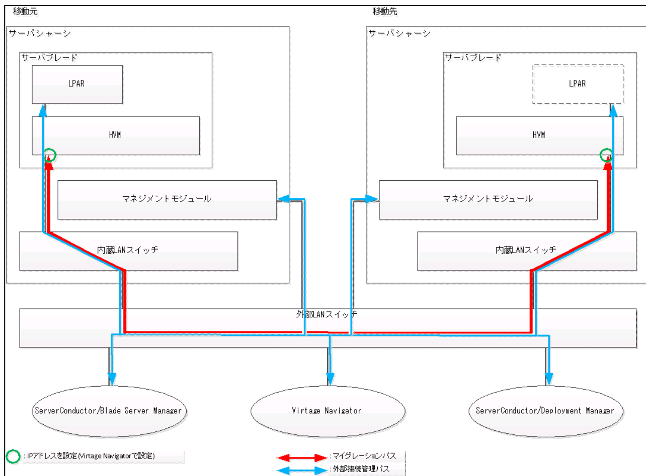
図 2-8 ネットワークの推奨構成
