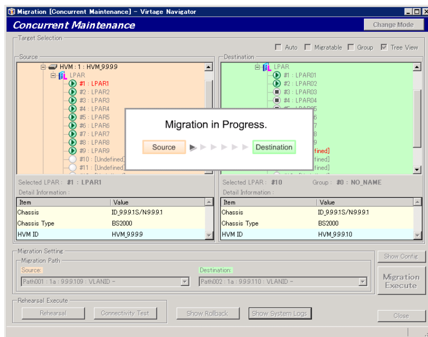
図 3-54 Migration[Concurrent Maintenance] ウィンドウ (コンカレントメンテナンスモード実施中)
