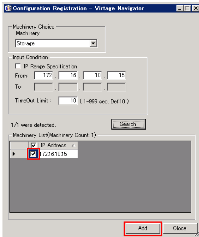
図 3-169 Configuration Registration ウィンドウ (Add クリック)
