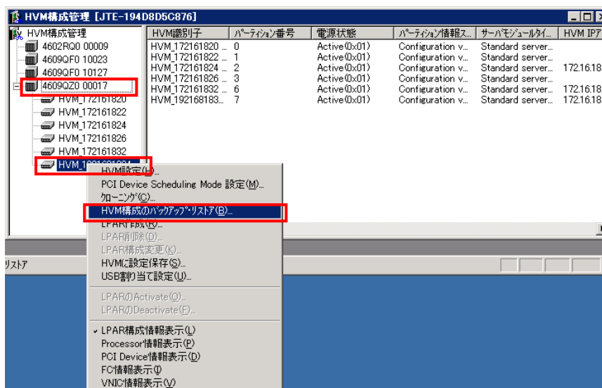
図 3-114 HVM 構成管理ウィンドウ ([HVM 構成のバックアップ・リストア (B)]の選択)
