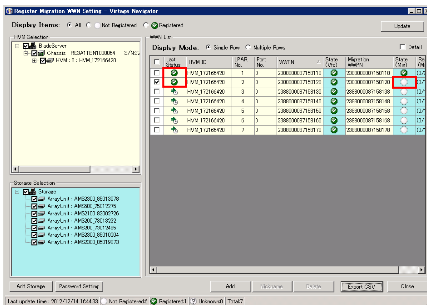
図 3-149 Register Migration WWN Setting ウィンドウ (マイグレーション WWPN 削除結果の確認)
