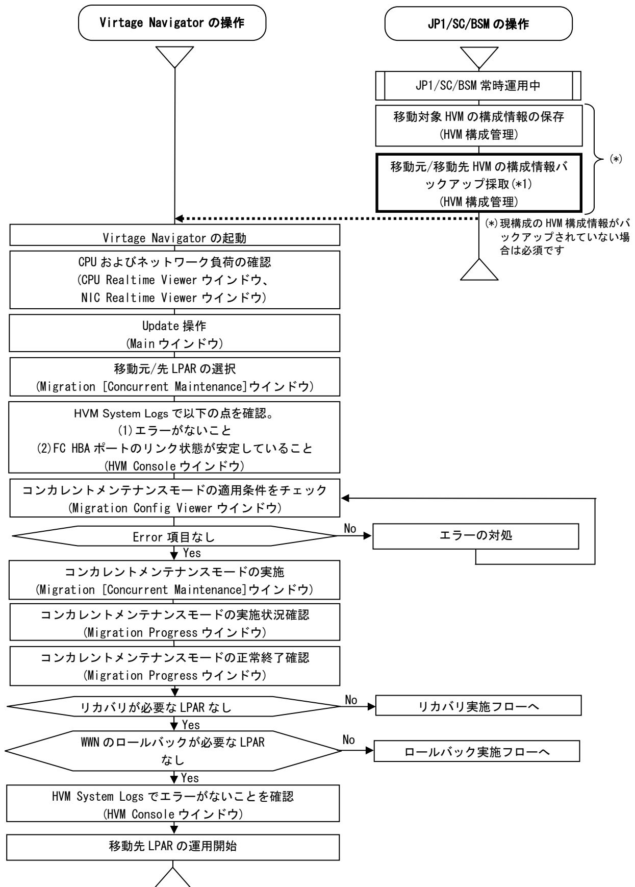
図 3-39 コンカレントメンテナンスモードの基本的な実施フロー
