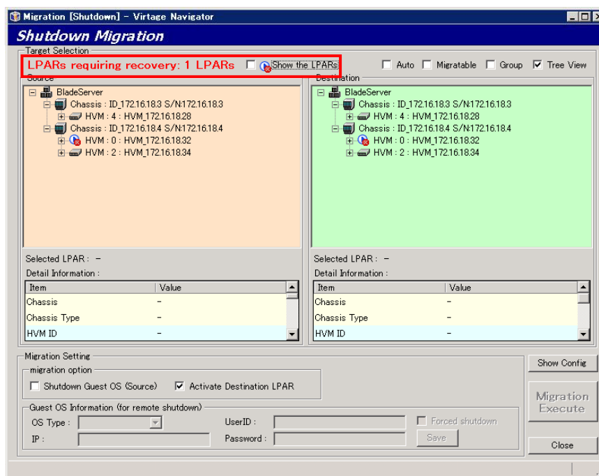
図 3-63 Migration[Concurrent Maintenance]ウィンドウ(手動リカバリ要 LPAR あり)
