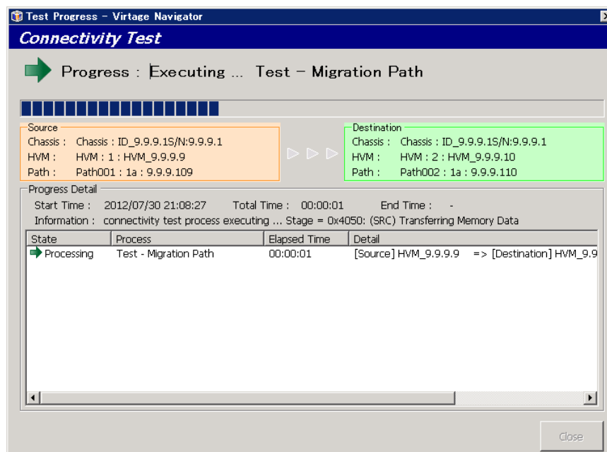
図 4-16 Migration Progress ウィンドウ(マイグレーションパス通信確認の進行状況表示)
