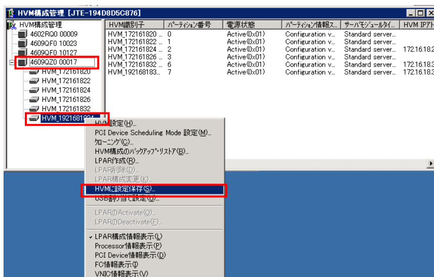
図 3-110 HVM 構成管理ウィンドウ(シャーシの選択)
