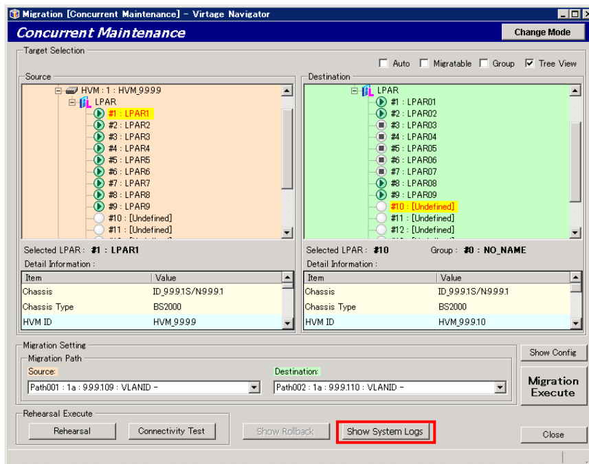
図 3-48 Migration[Concurrent Maintenance]ウインドウ (Show System Logs クリック)
