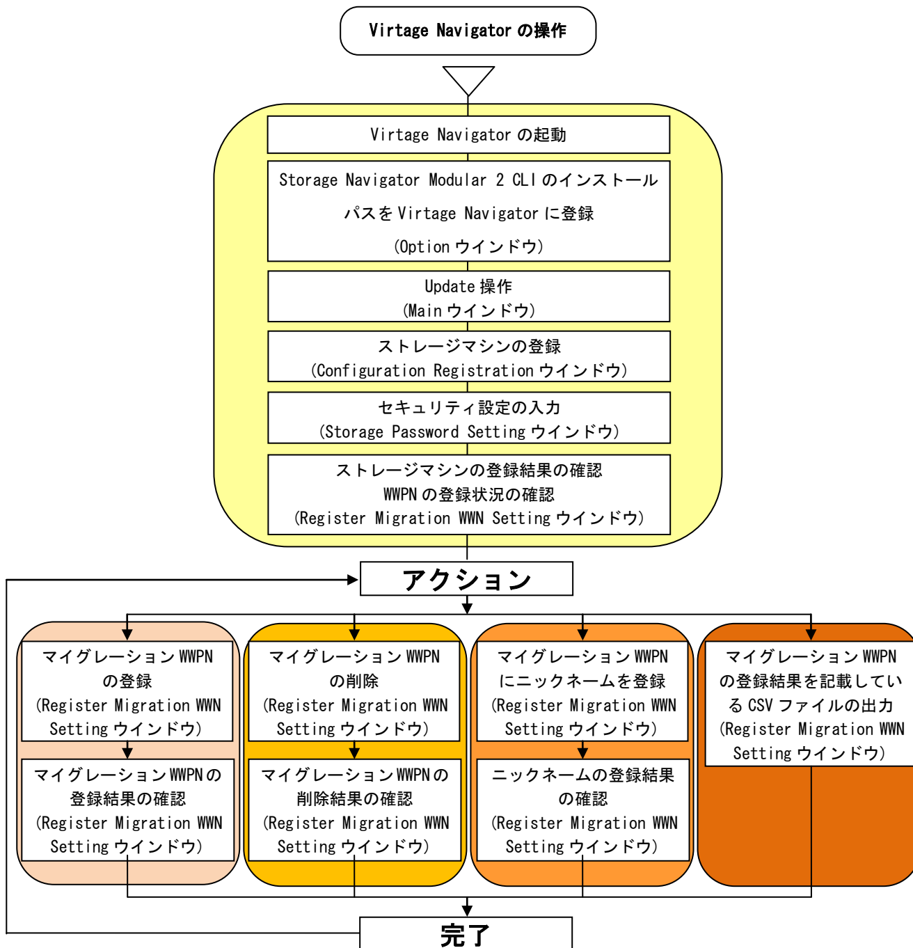
図 3-117 マイグレーション WPN 登録、削除フロー
