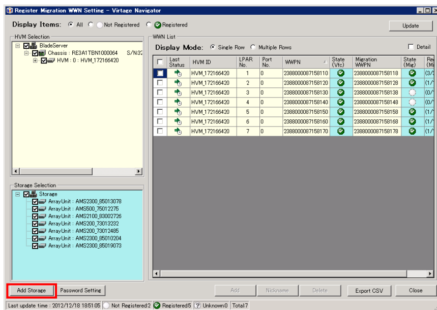
図 3-166 Register Migration WWN Setting ウィンドウ (OK クリック)
