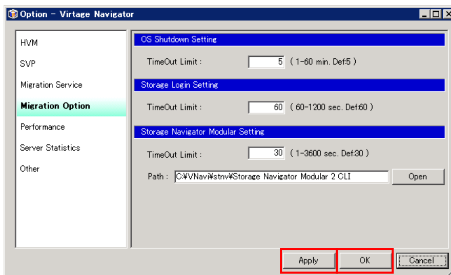
図 3-122 Option ウィンドウ (Storage Navigator Modular 2 CLI フォルダの選択)
