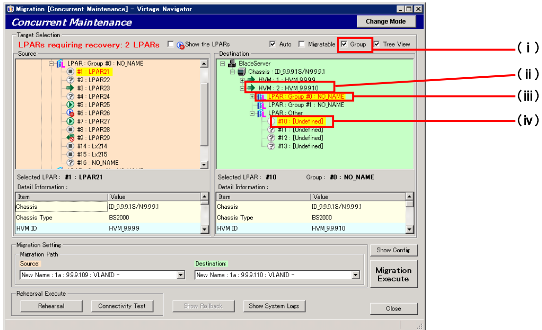
図 3-47 Migration[Concurrent Maintenance]ウインドウ(プロセッサグループ指定)
