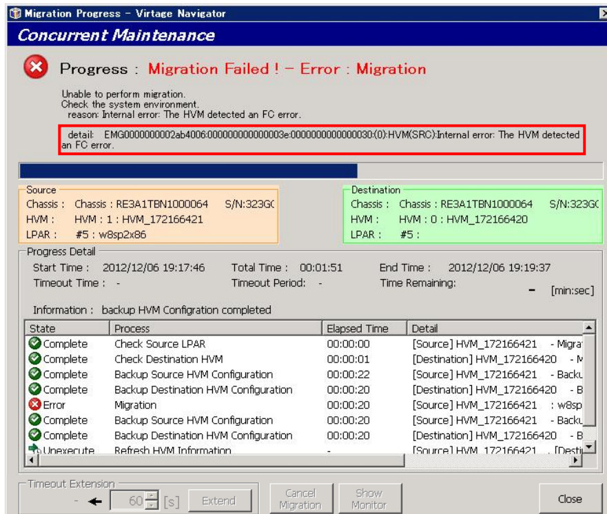
図 6-23 Migration Progress ウィンドウ (“EMG000000003004006:000000000000003e:0000000000000030:(0)” のエラー)
