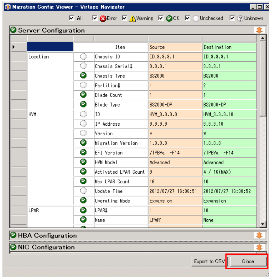
図 3-51 Migration[Concurrent Maintenance]ウィンドウ(適用条件の確認)
