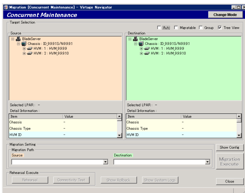
図 3-43 Migration[Concurrent Maintenance]ウィンドウ
