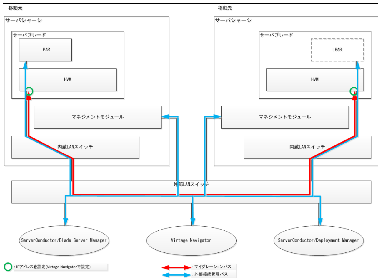
図 2-7 ネットワークの推奨構成 (BS500 の場合)
