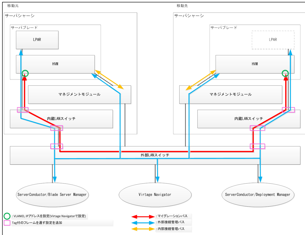
図 2-6 ネットワークの推奨構成 (BS2000 の場合)
