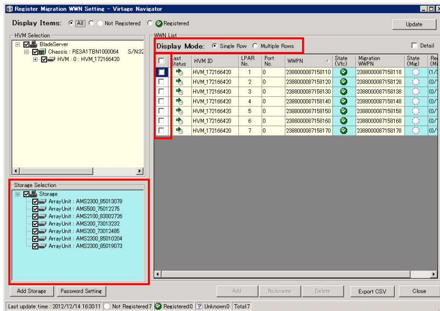
図 3-140 Register Migration WPN Setting ウィンドウ (マイグレーション WPN の選択)
