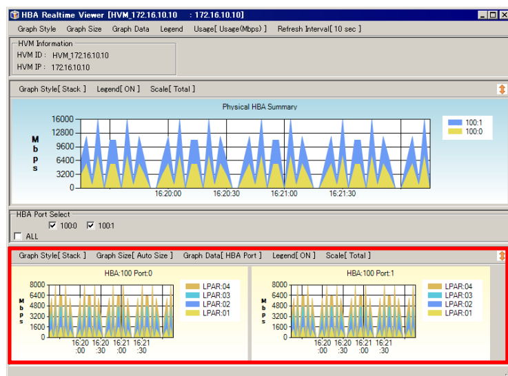
図 2-33 HBA Realtime Viewer[HVM ID : HVM IP]ウインドウ (HBA:xxx Port:n)
