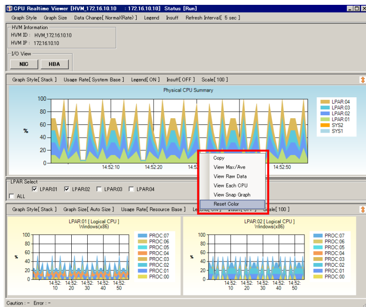
図 4-108 CPU/NIC/HBA Realtime Viewer[HVM_ID : HVM_IP] ウィンドウ
