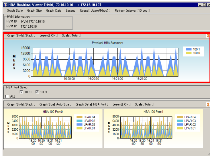
図 2-32 HBA Realtime Viewer[HVM ID : HVM IP]ウインドウ (Physical HBA Summary)
