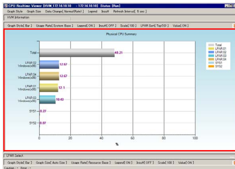
図 4-40 CPU Realtime Viewer[HVM_ID : HVM_IP]ウインドウ (Top10 表示)
