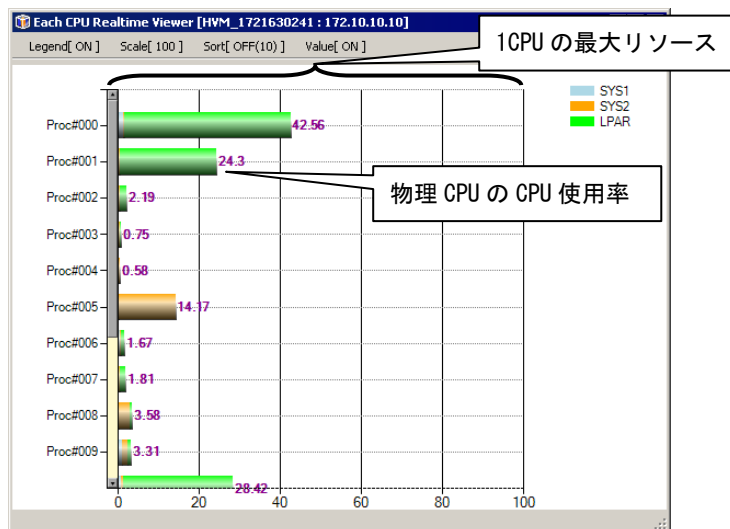
図 2-12 CPU Realtime Viewer[HVM ID : HVM IP]ウインドウ (Each CPU)
