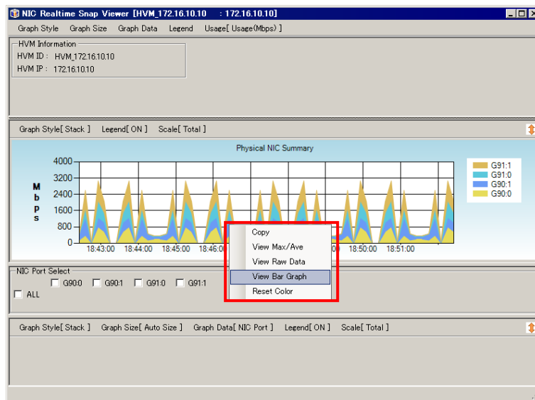
図 4-97 NIC/HBA Realtime Snap Viewer[HVM_ID : HVM_IP] ウィンドウ (View Bar Graph 選択)
