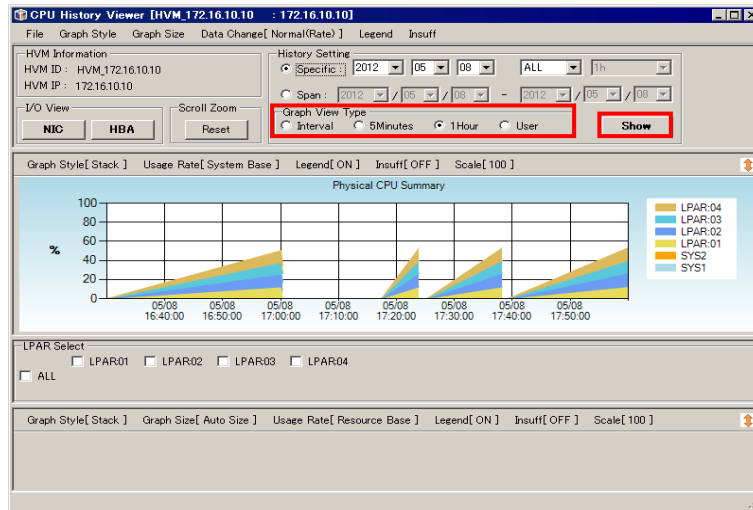
図 4-71 CPU/NIC/HBA History Viewer ウィンドウ (Show ボタンクリック)
