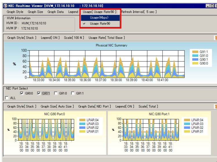
図 4-50 NIC/HBA Realtime Viewer[HVM ID : HVM IP]ウインドウ ([Usage]-[Usage (Mbps)]選択)
