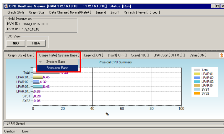
図 4-20 CPU Realtime Viewer[HVM_ID : HVM_IP]ウインドウ ([Usage Rate]-[Resource Base]選択)
