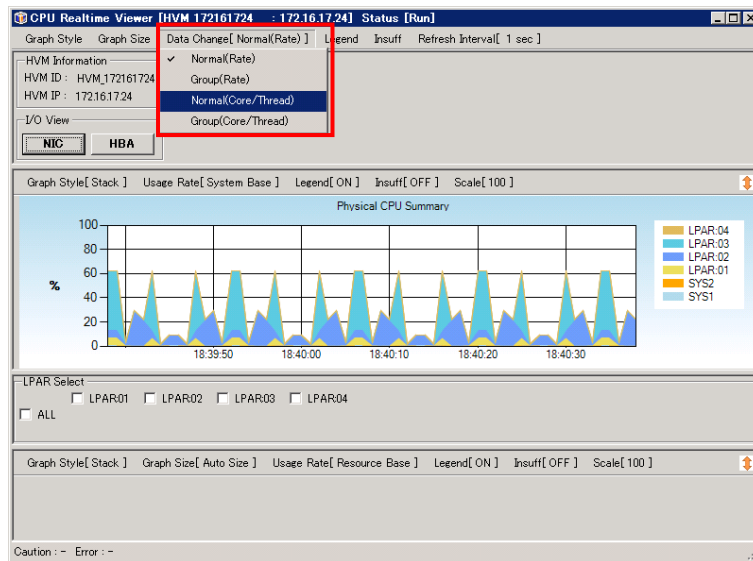
図 4-14 CPU Realtime Viewer [HVM_ID : HVM_IP] ウィンドウ ([Data Change]-[Normal (Core/Thread)] 選択)
