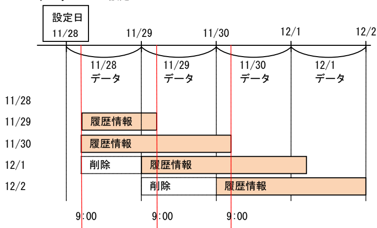
図 4-113 Auto Clear History Log (履歴情報自動削除機能概要)
