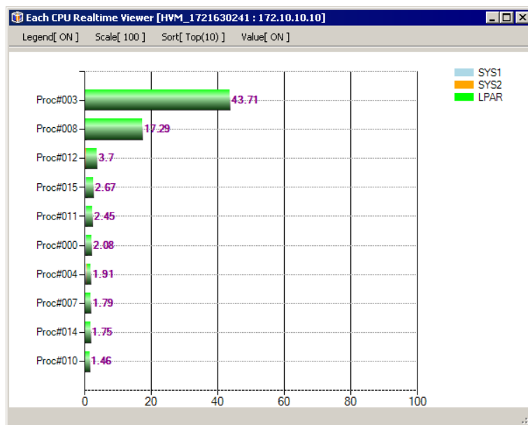
図 4-88 Each CPU Realtime Viewer ウィンドウ (Top10)
