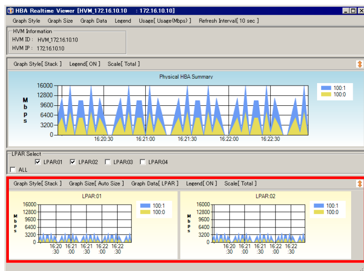
図 2-34 HBA Realtime Viewer[HVM ID : HVM IP]ウインドウ (LPAR:nn)
