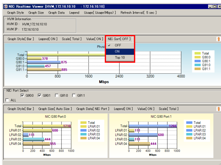
図 4-63 NIC/HBA Realtime Viewer[HVM ID : HVM IP]ウインドウ ([NIC/HBA Sort]-[ON]選択)
