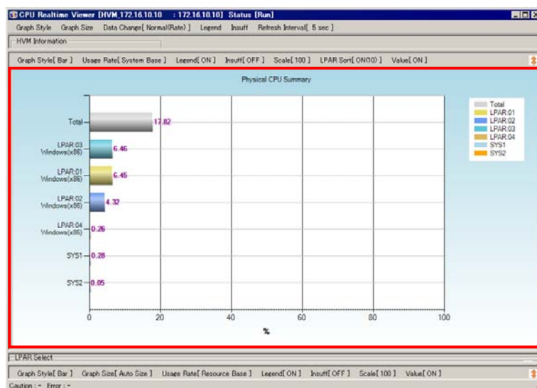
図 4-36 CPU Realtime Viewer[HVM_ID : HVM_IP]ウインドウ (ソート ON 表示)
