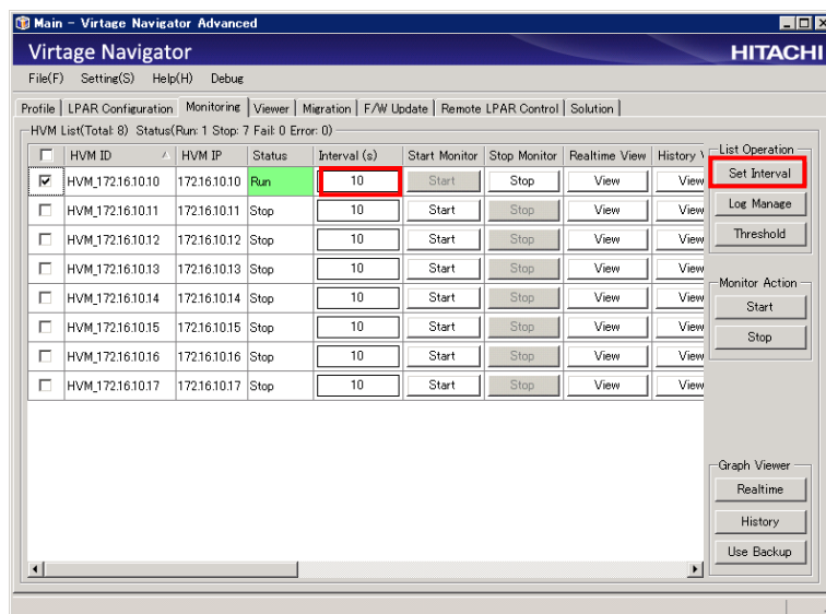
図 4-3 Main ウィンドウ (Interval 設定)
