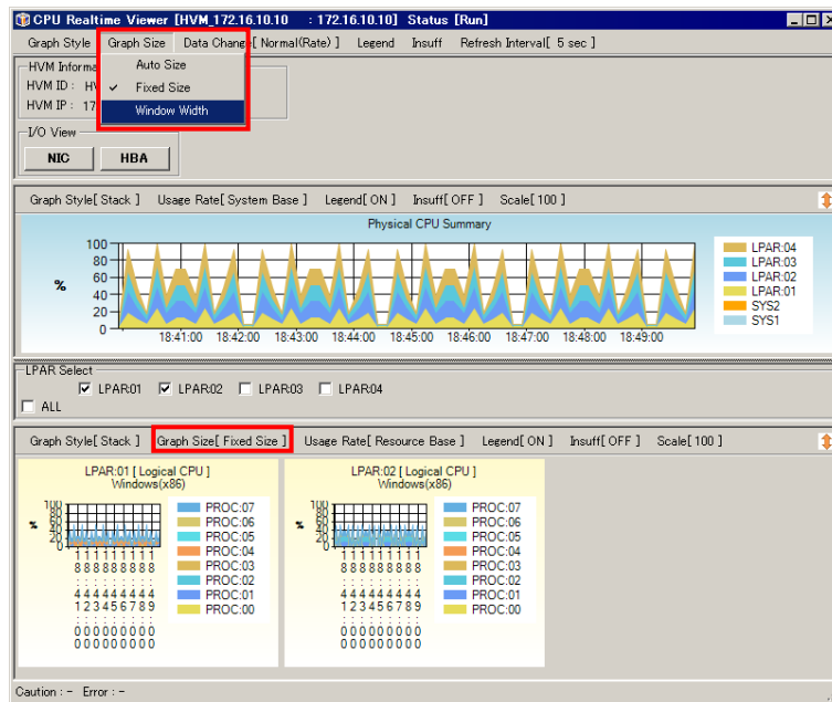
図 4-76 CPU/NIC/HBA Realtime Viewer [HVM_ID : HVM_IP] ウィンドウ ([Graph Size]-[Window Width] 選択)
