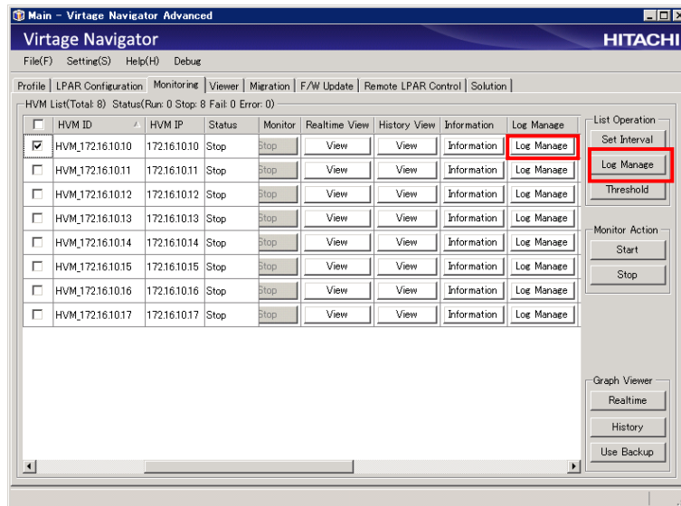
図 4-109 Main ウィンドウ (履歴情報自動集計ユーザ時間設定)
