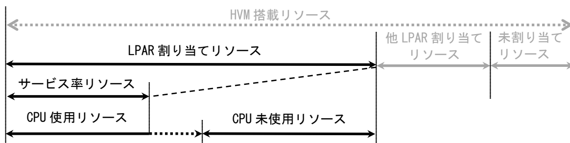
図 2-19 Data Change:Normal (Rate)、Usage Rate: Service Rate Base の場合の性能データ
