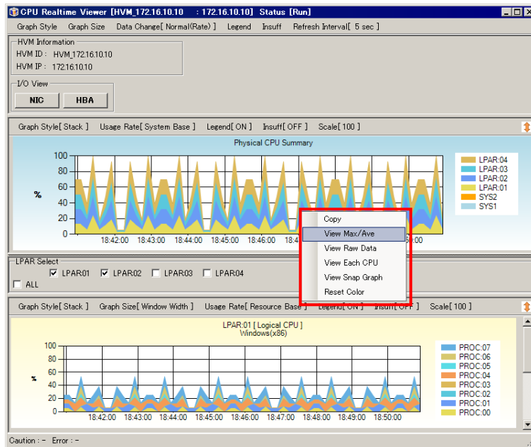
図 4-79 CPU/NIC/HBA Realtime Viewer ウィンドウ (View Max/Ave 選択)
