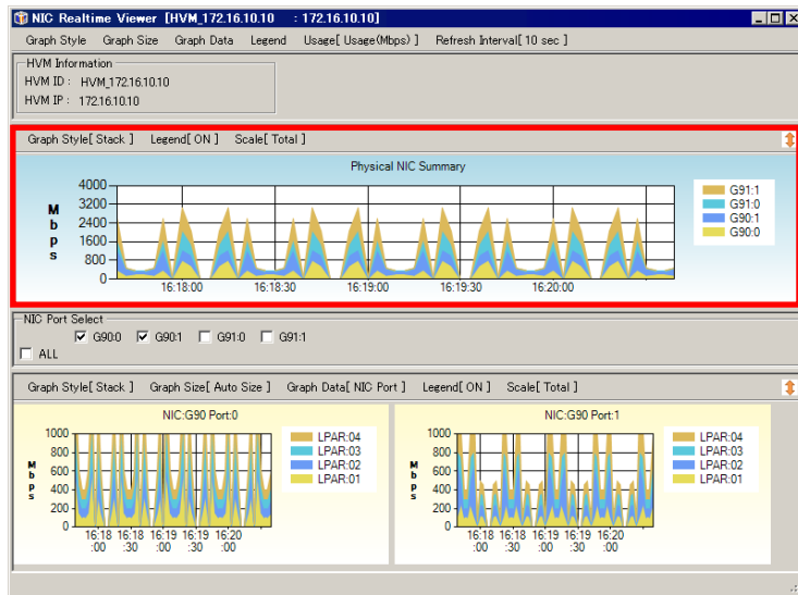
図 2-28 NIC Realtime Viewer[HVM ID : HVM IP]ウインドウ (Physical NIC Summary)
