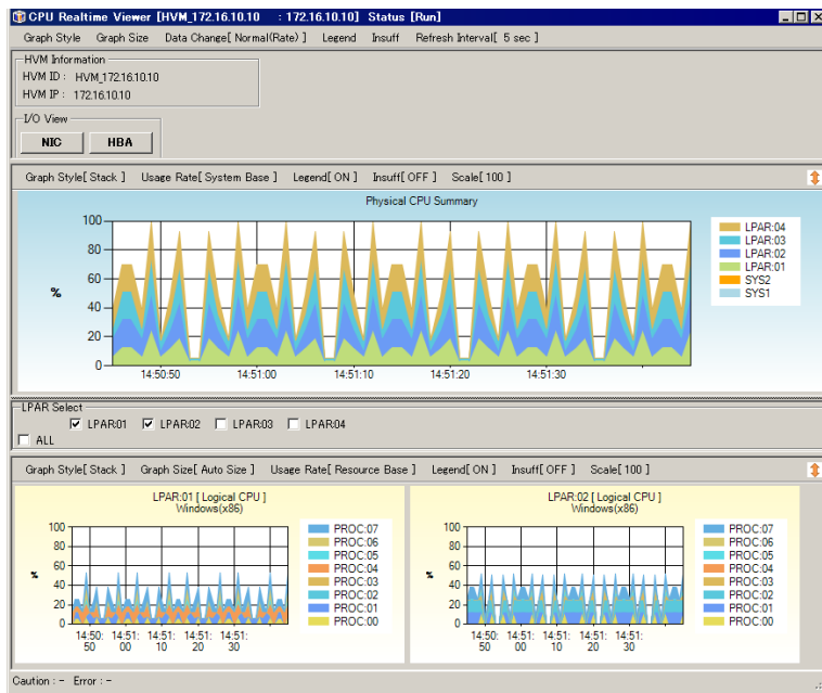
図 4-107 CPU/NIC/HBA Realtime Viewer[HVM ID : HVM IP] ウィンドウ
