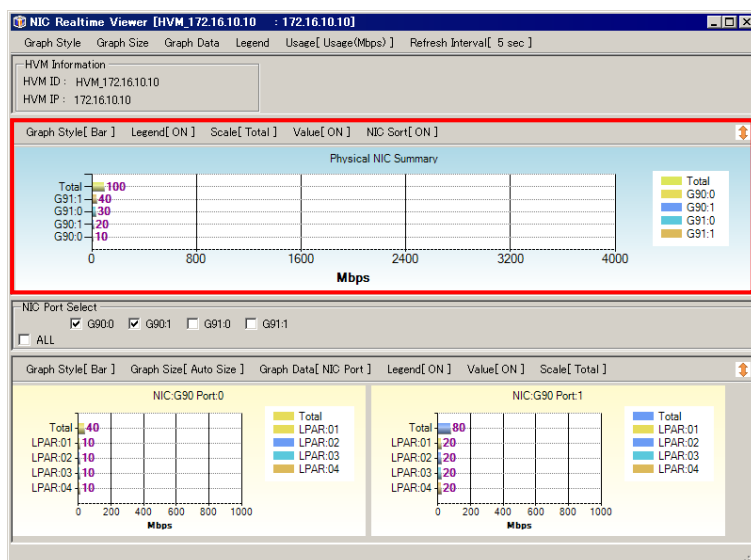
図 4-64 NIC/HBA Realtime Viewer[HVM ID : HVM IP]ウインドウ (ソート ON 表示)
