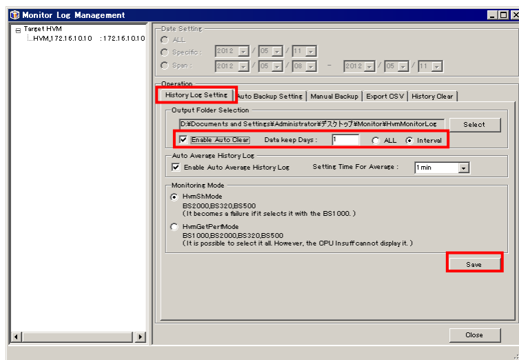
図 4-112 Monitor Log Management ウィンドウ (履歴情報自動削除設定)
