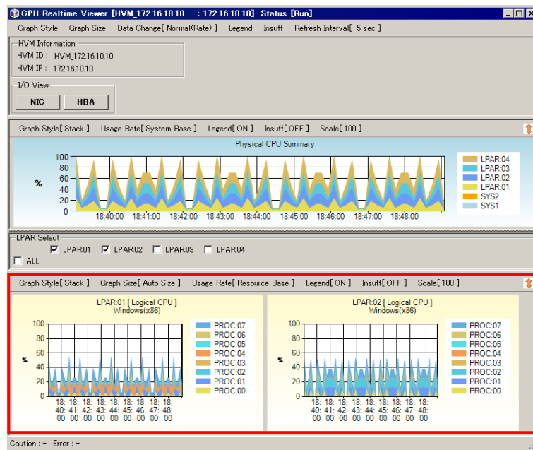
図 4-73 CPU/NIC/HBA Realtime Viewer [HVM_ID : HVM_IP] ウィンドウ ([Auto Size]表示)
