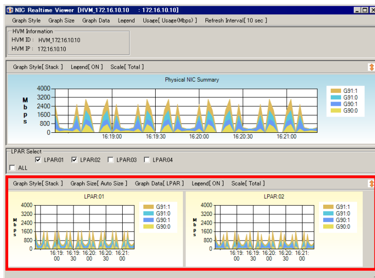
図 2-30 NIC Realtime Viewer[HVM ID : HVM IP]ウインドウ (LPAR:nn)
