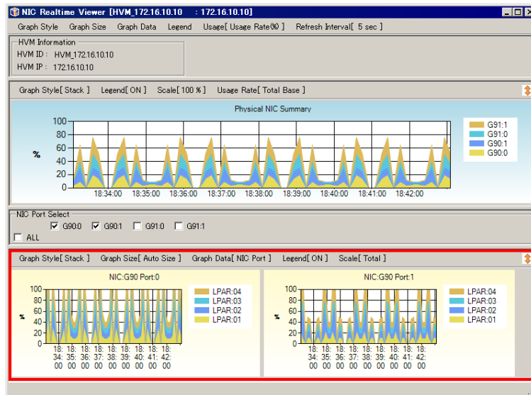
図 4-54 NIC/HBA Realtime Viewer[HVM ID : HVM IP]ウィンドウ (NIC/HBA のポートごとの使用率表示)
