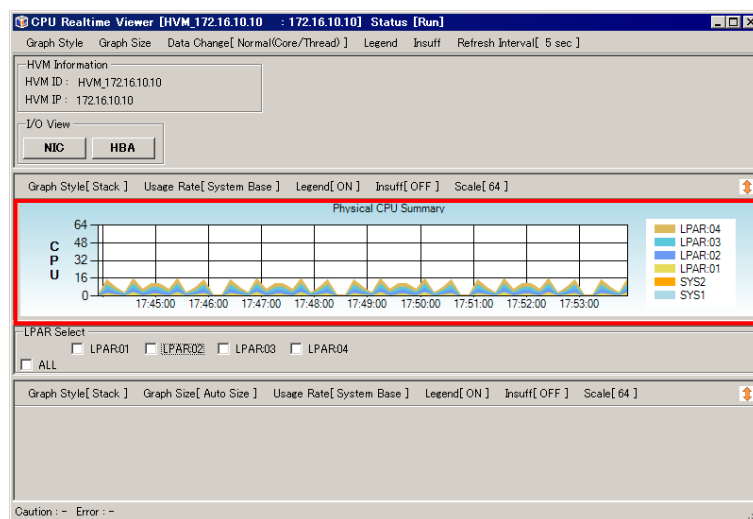
図 4-15 CPU Realtime Viewer [HVM_ID : HVM_IP] ウィンドウ (LPAR ごとのコア数またはスレッド数での CPU 使用量表示)
