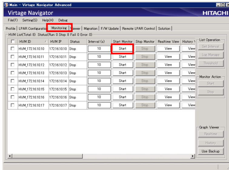
図 3-1 Main ウィンドウ (モニタリングの開始)
