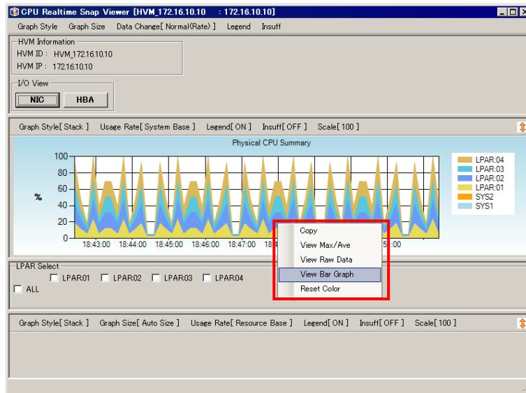
図 4-91 CPU Realtime Snap Viewer[HVM_ID : HVM_IP]ウインドウ (View Bar Graph 表示)
