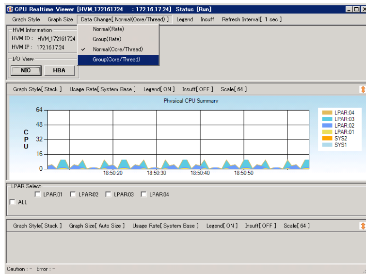
図 4-16 CPU Realtime Viewer[HVM_ID : HVM_IP]ウインドウ ([Data Change]-[Group(Core/Thread)]選択)
