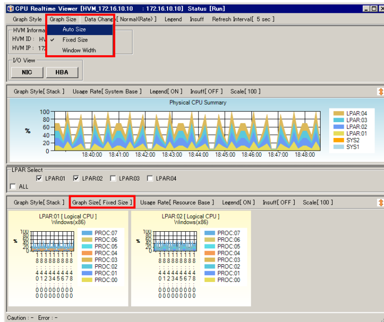
図 4-72 CPU/NIC/HBA Realtime Viewer[HVM_ID : HVM_IP]ウインドウ ([Graph Size]-[Auto Size]選択)
