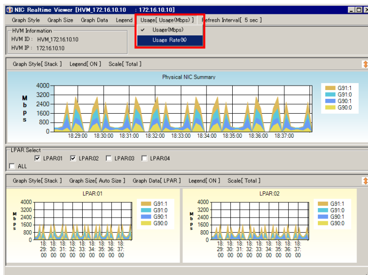
図 4-59 NIC/HBA Realtime Viewer[HVM ID : HVM IP]ウインドウ ([Usage]-[Usage Rate(%)]選択)
