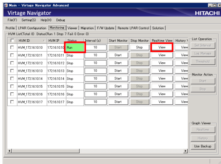
図 3-2 Main ウィンドウ (Realtime View 表示)
