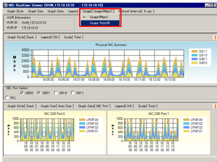
図 4-41 NIC/HBA Realtime Viewer[HVM ID : HVM IP]ウインドウ ([Usage]-[Usage Rate(%)]選択)
