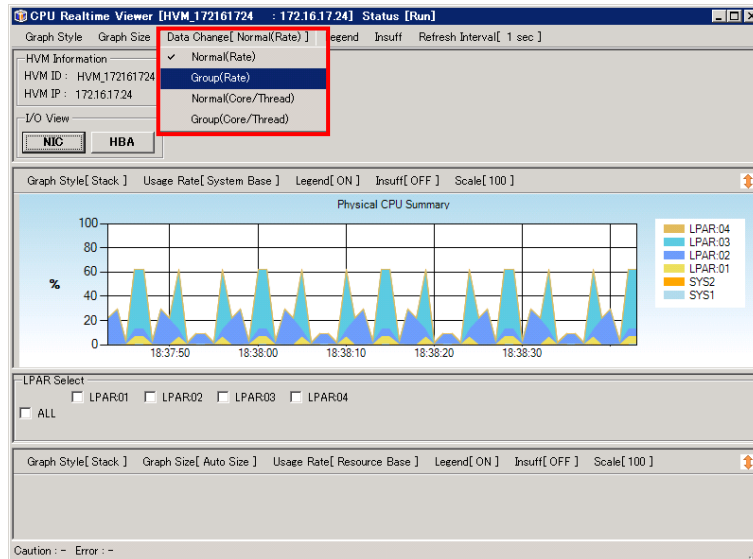
図 4-29 CPU Realtime Viewer[HVM_ID : HVM_IP]ウインドウ ([Data Change]-[Group(Rate)]選択)
