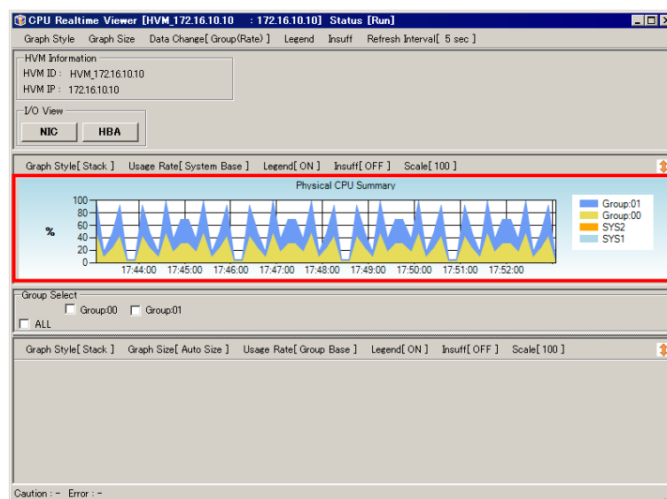
図 4-13 CPU Realtime Viewer[HVM_ID : HVM_IP]ウィンドウ (プロセッサグループごとの CPU 使用率の表示)
