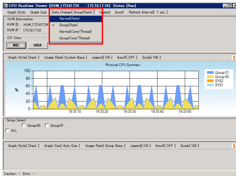
図 4-18 CPU Realtime Viewer[HVM_ID : HVM_IP]ウインドウ ([Data Change]–[Normal (Rate)]選択)
