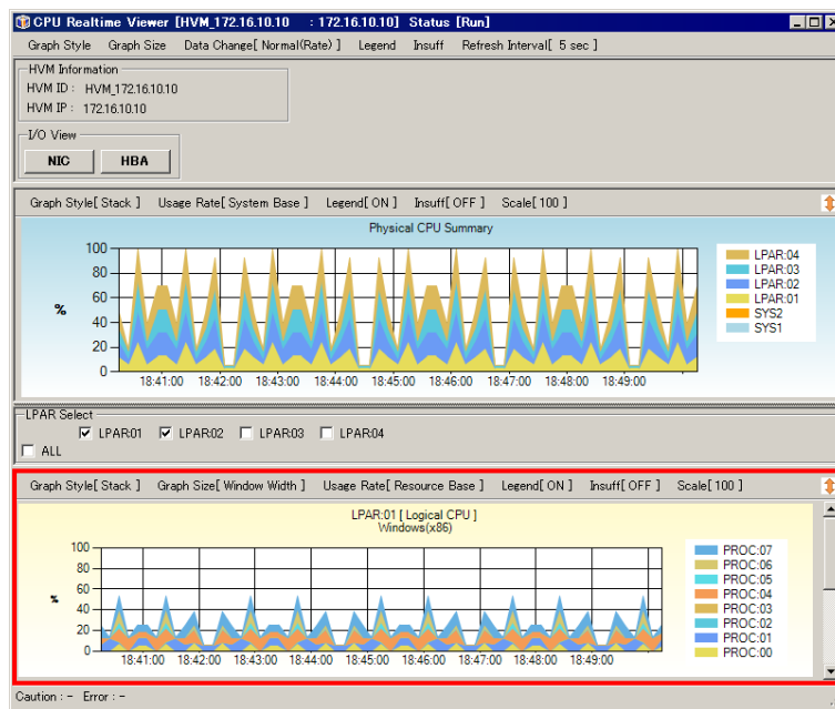
図 4-77 CPU/NIC/HBA Realtime Viewer[HVM_ID : HVM_IP]ウィンドウ ([Window Width]表示)
