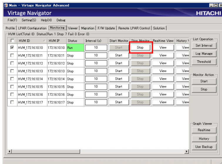
図 4-1 Main ウィンドウ(モニタリング停止)
