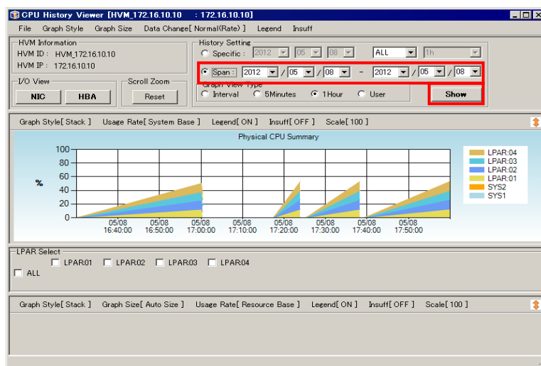
図 4-70 CPU/NIC/HBA History Viewer ウィンドウ (グラフ表示時間範囲設定(Span))
