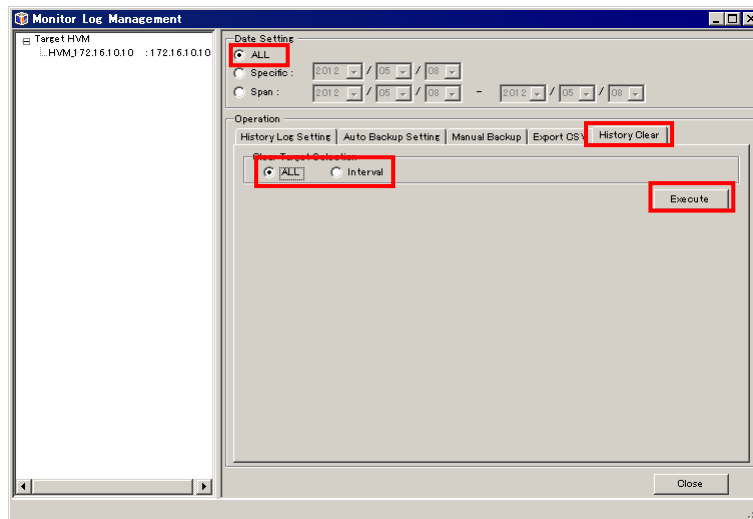
図 4-124 Monitor Log Management ウィンドウ (履歴情報手動削除実行)
