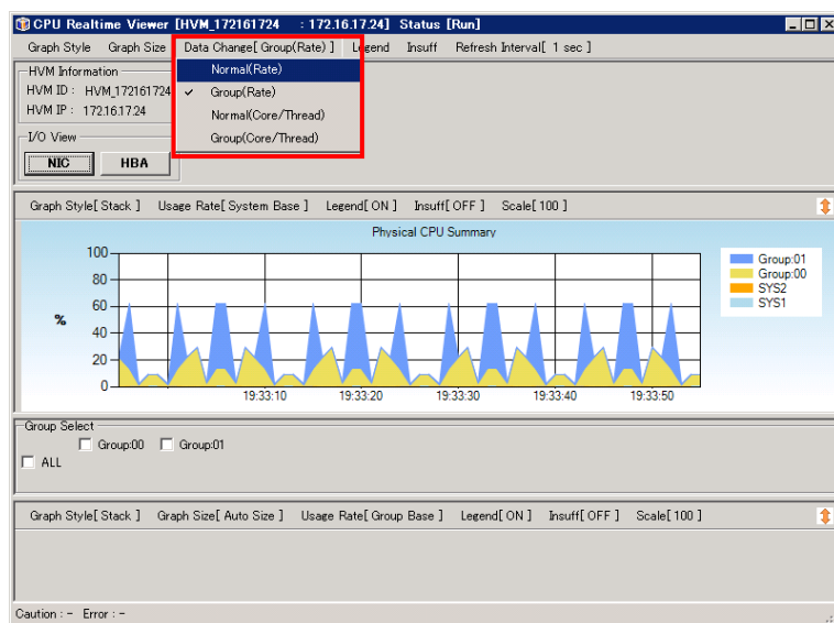
図 4-21 CPU Realtime Viewer [HVM_ID : HVM_IP] ウィンドウ ([Data Change]-[Normal (Rate)]選択)
