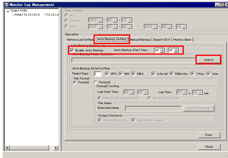
図 4-114 Monitor Log Management ウィンドウ
