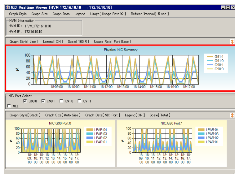
図 4-48 NIC/HBA Realtime Viewer[HVM ID : HVM IP]ウインドウ (物理(共有)のポート基準の NIC/HBA 使用率表示)
