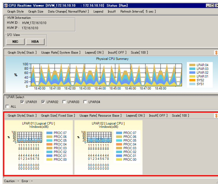
図 4-75 CPU/NIC/HBA Realtime Viewer [HVM_ID : HVM_IP] ウィンドウ ([Fixed Size]表示)
