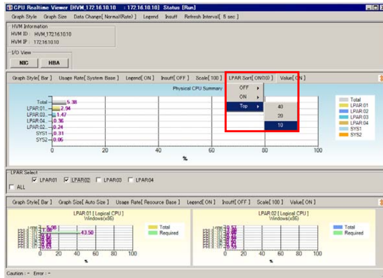
図 4-39 CPU Realtime Viewer[HVM_ID : HVM_IP]ウインドウ ([LPAR Sort]-[Top]-[10]選択)
