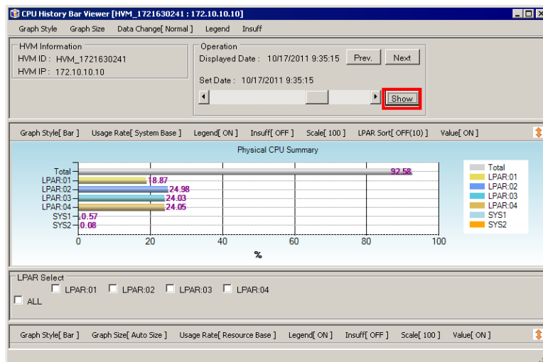
図 4-94 CPU History Bar Viewer [HVM_ID : HVM_IP] ウィンドウ (瞬間バーグラフ表示)
