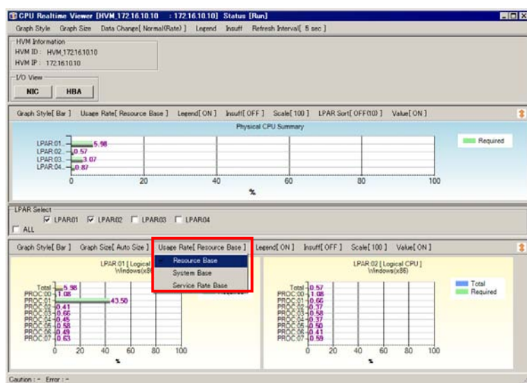
図 4-22 CPU Realtime Viewer [HVM_ID : HVM_IP] ウィンドウ ([Usage Rate]-[Resource Base]選択)
