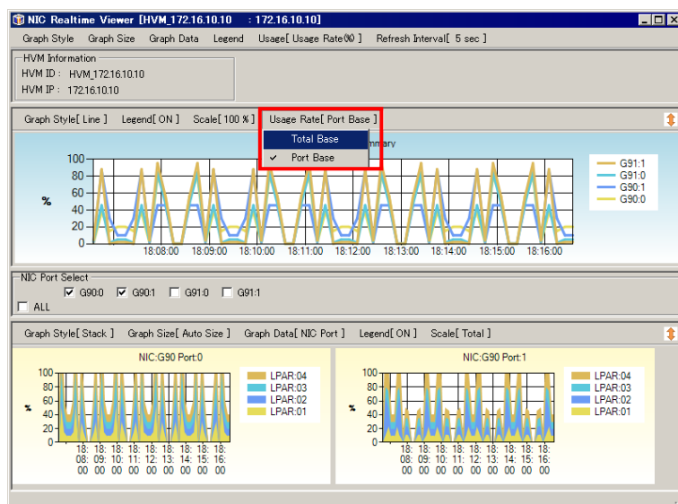
図 4-43 NIC/HBA Realtime Viewer[HVM ID : HVM IP]ウインドウ ([Usage Rate]-[Total Base]選択)
