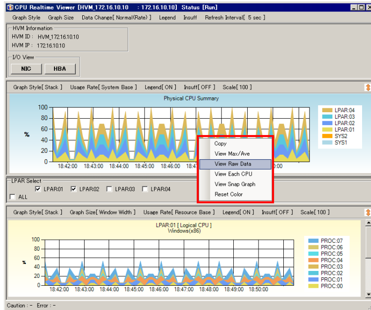
図 4-81 CPU/NIC/HBA Realtime Viewer ウィンドウ (View Raw Data 選択)
