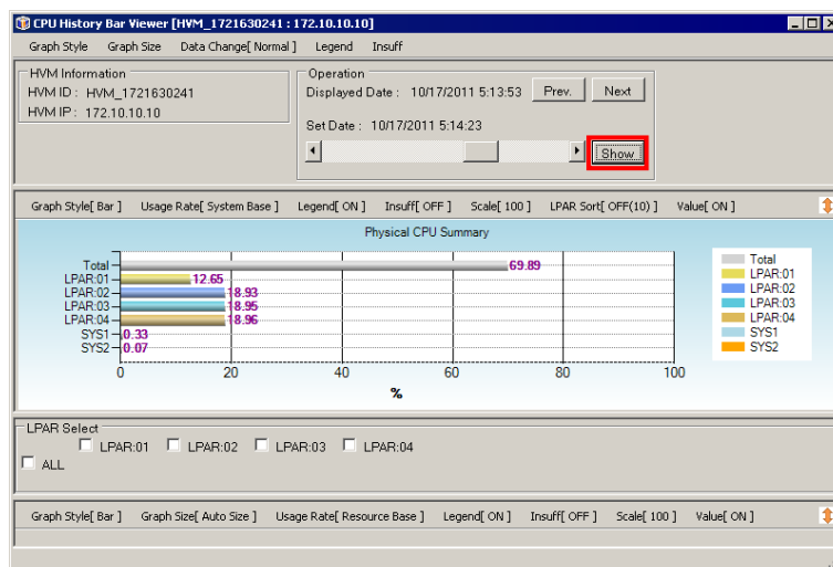
図 4-100 NIC/HBA History Bar Viewer[HVM_ID : HVM_IP]ウィンドウ
