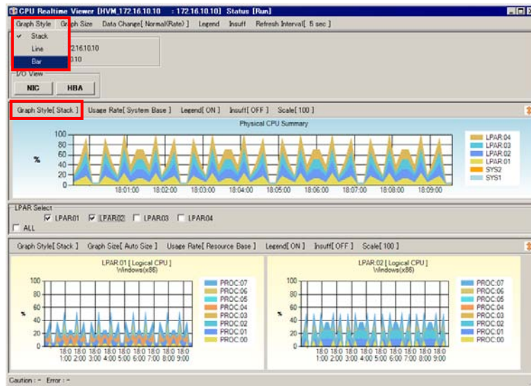
図 4-33 CPU Realtime Viewer[HVM_ID : HVM_IP]ウィンドウ ([Graph Style]-[Bar]選択)
