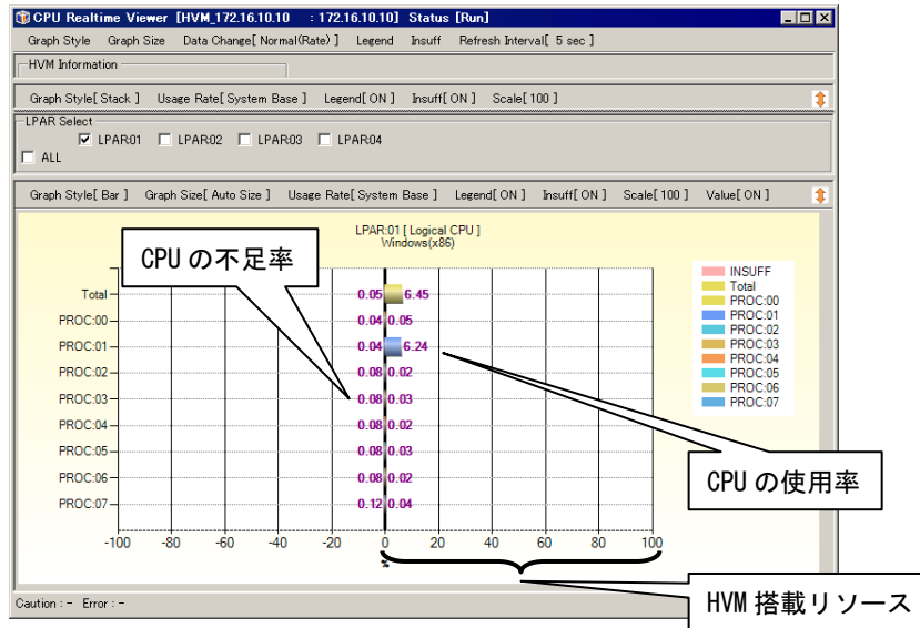
図 2-16 CPU Realtime Viewer[HVM ID : HVM IP]ウインドウ (LPAR:nn[Logical CPU] [Case 2])
