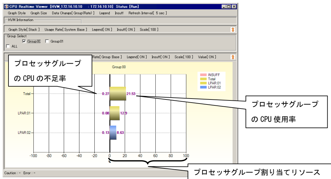
図 2-22 CPU Realtime Viewer[HVM ID : HVM IP] ウィンドウ (Group:nn [Case 1])
