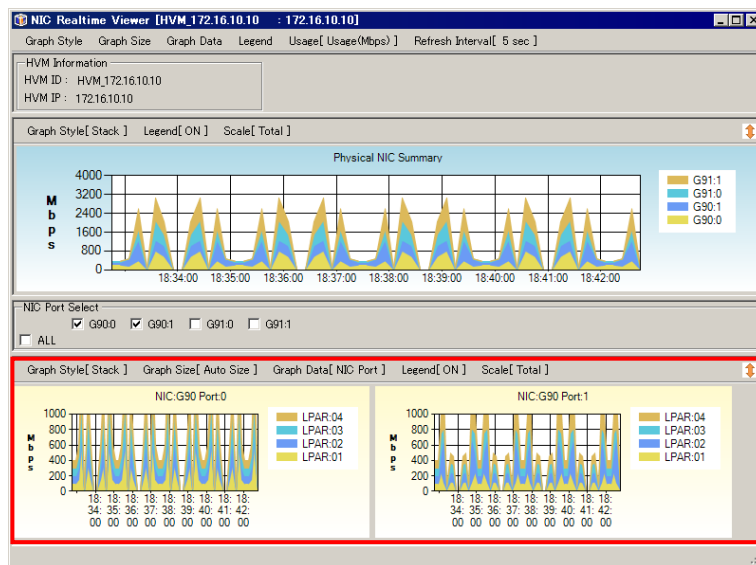
図 4-51 NIC/HBA Realtime Viewer[HVM ID : HVM IP]ウィンドウ (NIC/HBA のポートごとの使用量表示)
