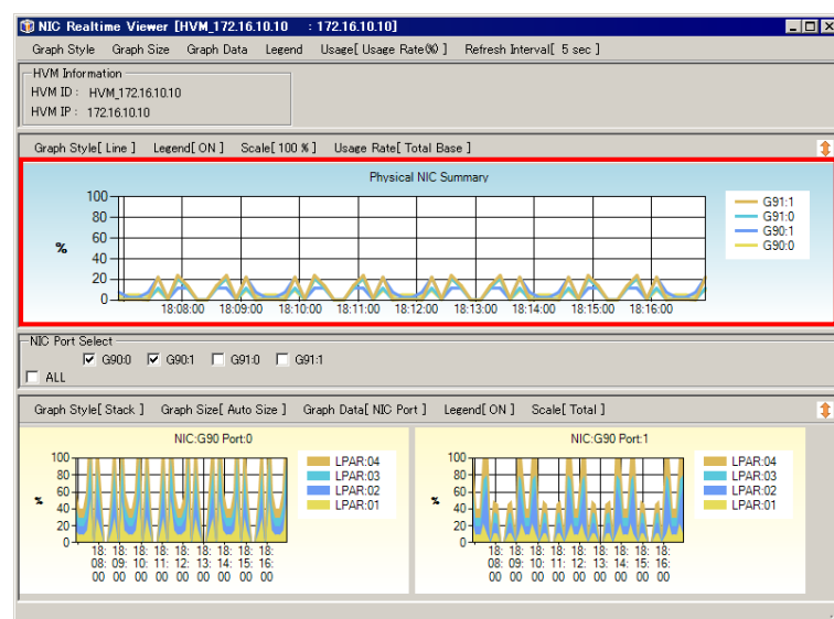
図 4-44 NIC/HBA Realtime Viewer[HVM ID : HVM IP]ウインドウ (全物理(共有)基準の NIC/HBA 使用率表示)
