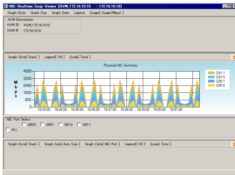
図 4-96 NIC/HBA Realtime Snap Viewer[HVM_ID : HVM_IP]ウインドウ
