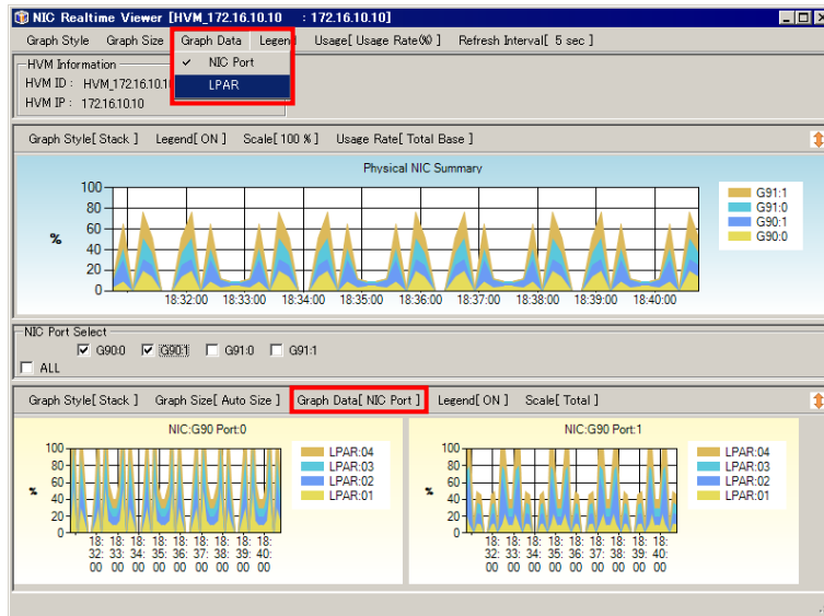
図 4-55 NIC/HBA Realtime Viewer[HVM ID : HVM IP]ウィンドウ ([Graph Data]-[LPAR]選択)
