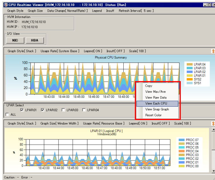
図 4-83 CPU Realtime Viewer[HVM_ID : HVM_IP]ウィンドウ (View Each CPU 選択)
