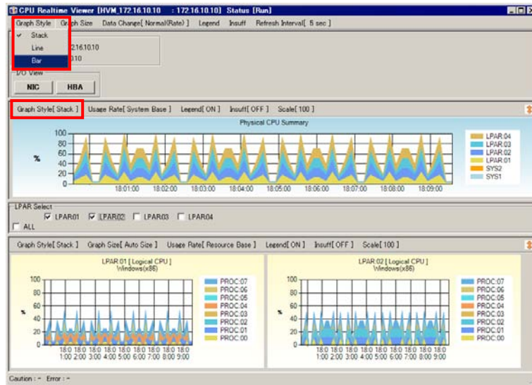
図 4-37 CPU Realtime Viewer[HVM_ID : HVM_IP]ウィンドウ ([Graph Style]-[Bar]選択)
