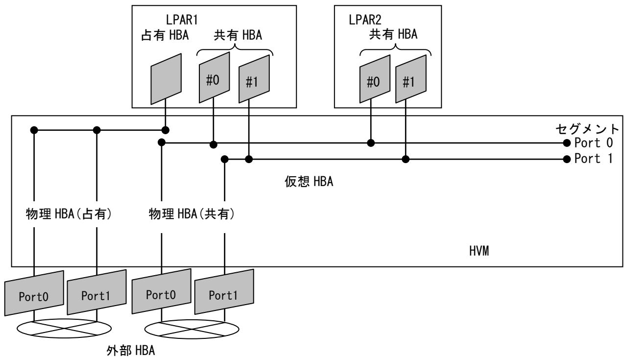
図 2-35 1HVM 上の LPAR への HBA の割り当て
