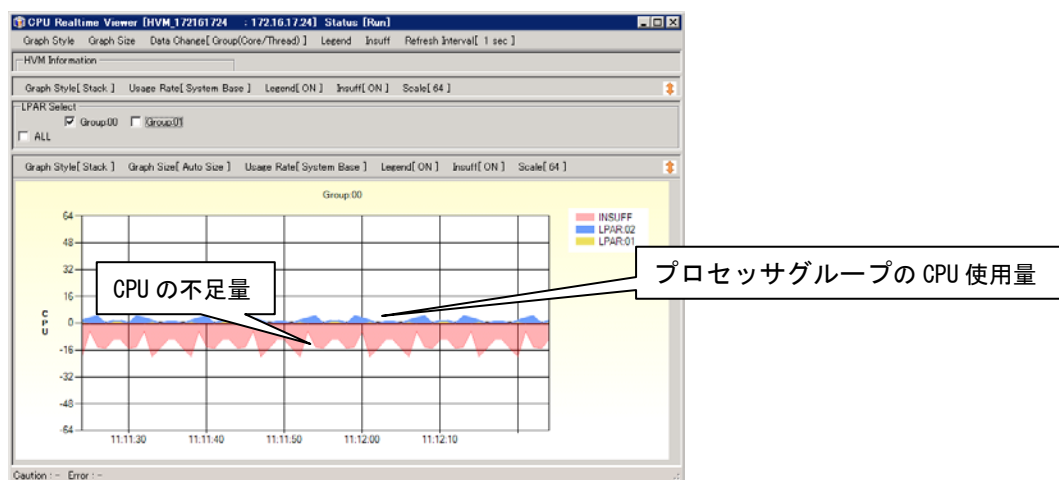
図 2-26 CPU Realtime Viewer[HVM ID : HVM IP]ウインドウ (Group:nn [Case 3])
