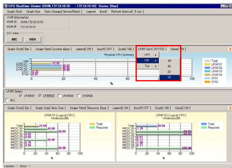
図 4-35 CPU Realtime Viewer[HVM_ID : HVM_IP]ウインドウ ([LPAR Sort]-[ON]-[10]選択)
