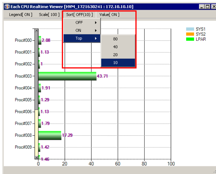
図 4-87 Each CPU Realtime Viewer ウィンドウ ([Sort]-[Top]-[10]選択)
