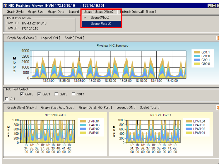
図 4-53 NIC/HBA Realtime Viewer[HVM ID : HVM IP]ウィンドウ ([Usage]-[Usage Rate(%)]選択)
