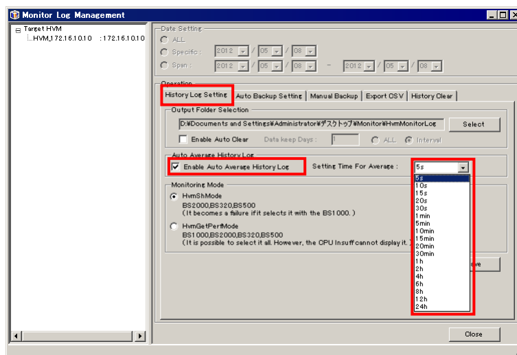
図 4-110 Monitoring Log Management ウィンドウ (集計時間間隔設定)
