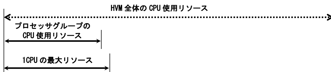
図 2-27 Data Change:Group(Core/Thread) の場合の性能データ
