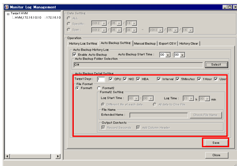
図 4-116 Monitor Log Management ウィンドウ(履歴情報自動バックアップ設定保存)
