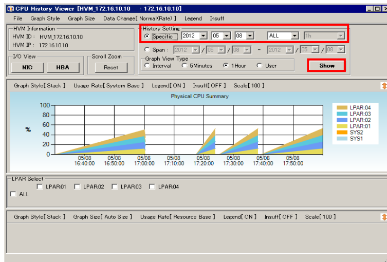
図 4-69 CPU/NIC/HBA History Viewer ウィンドウ (グラフ表示時間範囲設定(Specific))
