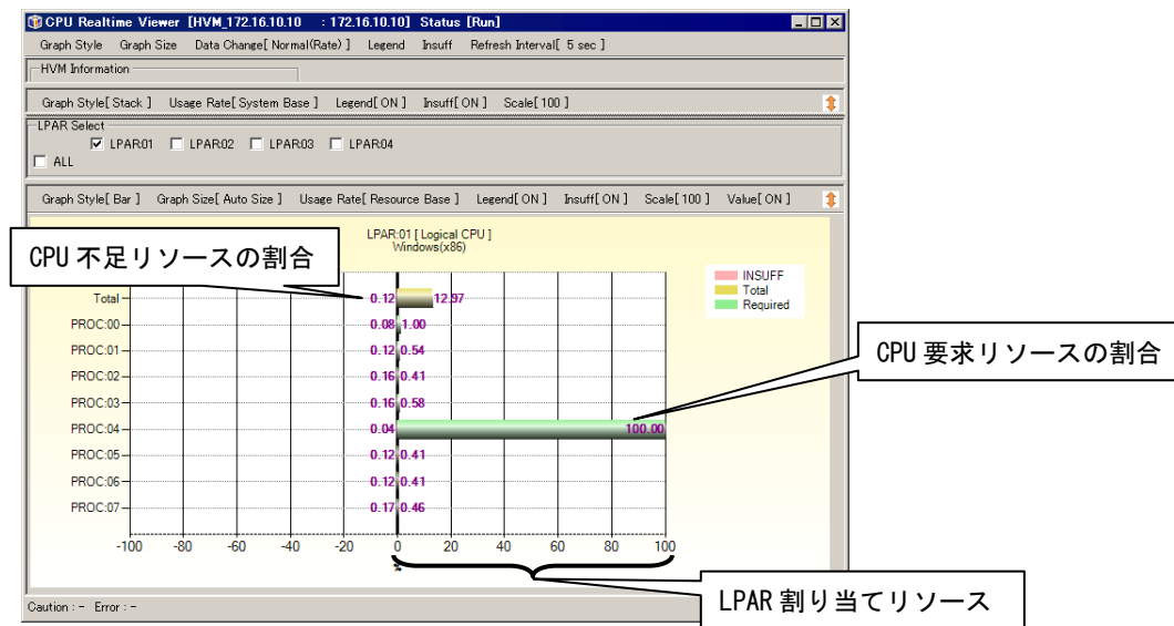
図 2-14 CPU Realtime Viewer[HVM ID : HVM IP]ウインドウ (LPAR:nn[Logical CPU] [Case 1])
