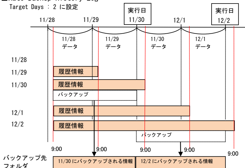
図 4-117 Auto BackUp History Log(履歴情報自動バックアップ機能概要)
