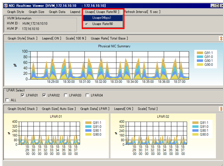
図 4-56 NIC/HBA Realtime Viewer[HVM ID : HVM IP]ウィンドウ ([Usage]-[Usage(Mbps)]選択)
