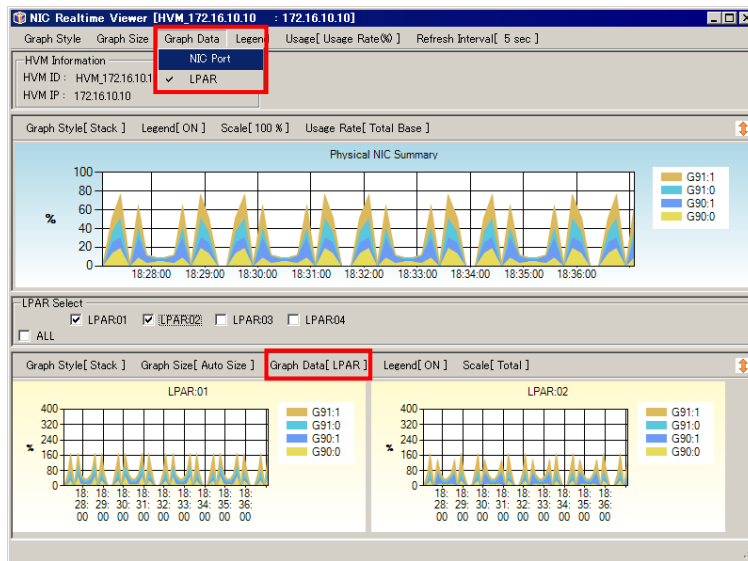
図 4-52 NIC/HBA Realtime Viewer[HVM ID : HVM IP]ウィンドウ ([Graph Data]-[NIC/HBA Port]選択)
