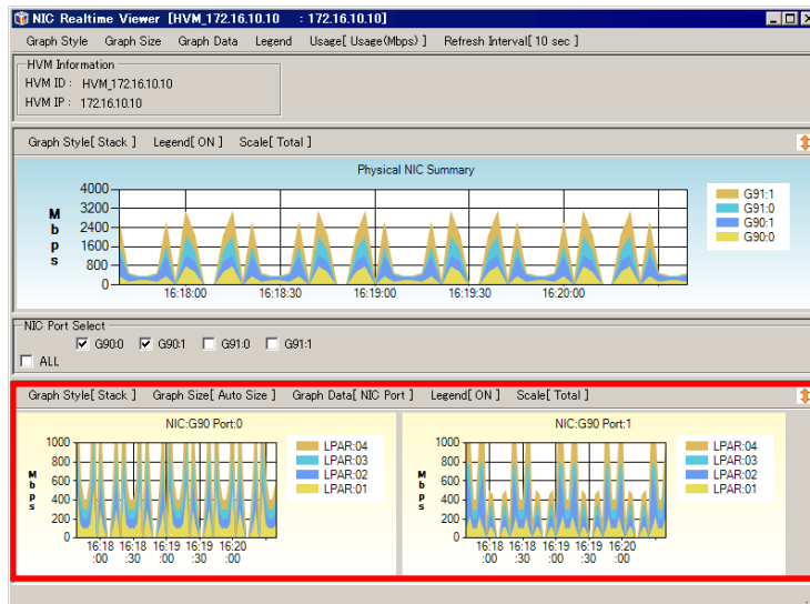
図 2-29 NIC Realtime Viewer[HVM ID : HVM IP]ウインドウ (NIC:xxx Port:n)
