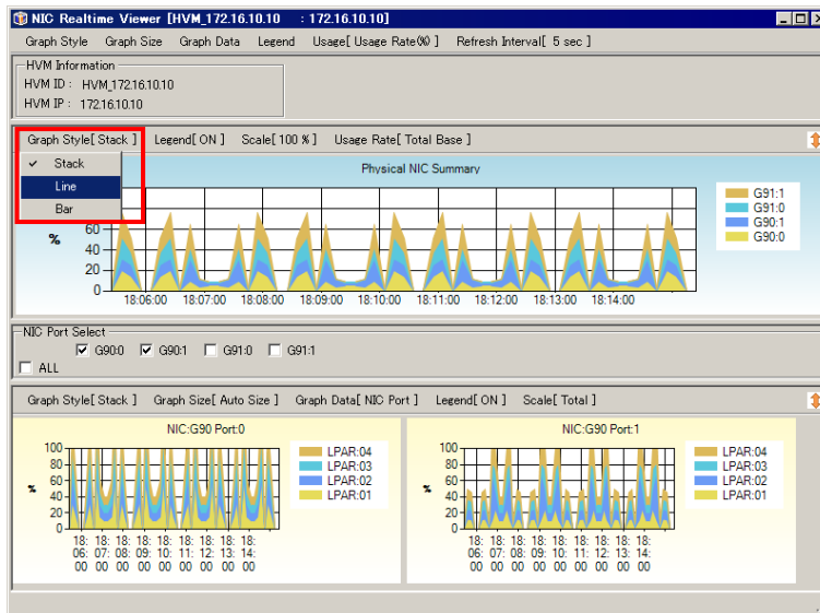
図 4-46 NIC/HBA Realtime Viewer[HVM ID : HVM IP]ウインドウ ([Graph Style]-[Line]選択)
