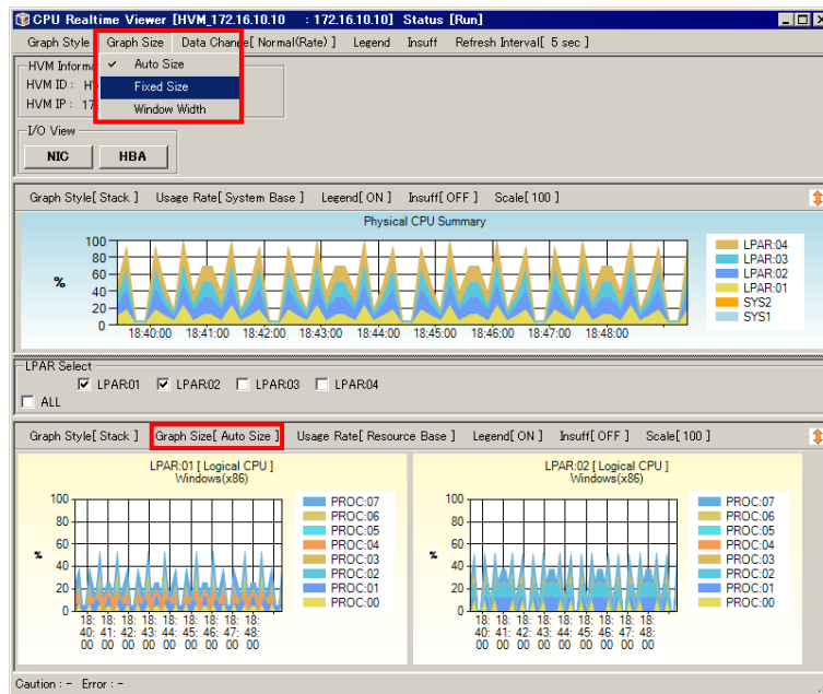
図 4-74 CPU/NIC/HBA Realtime Viewer[HVM_ID : HVM_IP]ウィンドウ ([Graph Size]-[Fixed Size]選択)
