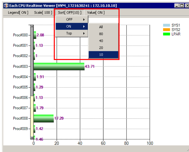
図 4-85 Each CPU Realtime Viewer ウィンドウ([Sort]-[ON]-[10]選択)
