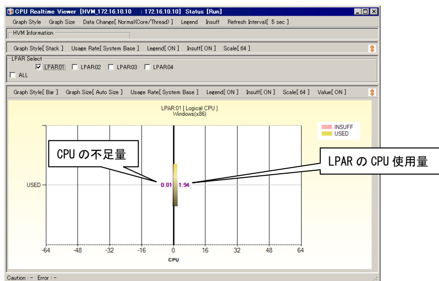
図 2-20 CPU Realtime Viewer[HVM ID : HVM IP]ウインドウ (LPAR:nn[Logical CPU] [Case 4])
