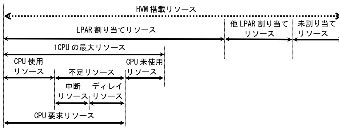
図 2-15 Data Change:Normal (Rate)、Usage Rate: Resource Base の場合の性能データ
