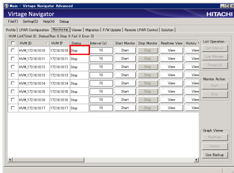
図 4-2 Main ウィンドウ(Status 列確認)
