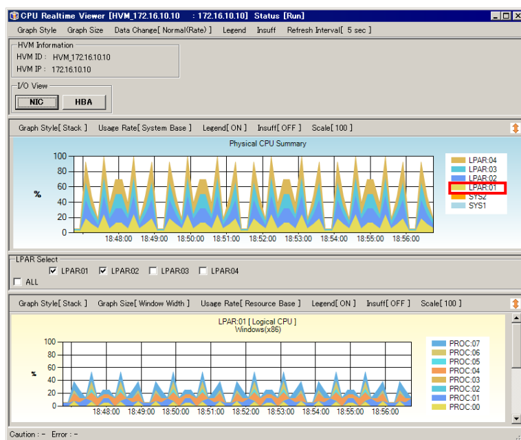
図 4-104 CPU/NIC/HBA Realtime Viewer[HVM_ID : HVM_IP] ウィンドウ (レジェンドクリック)
