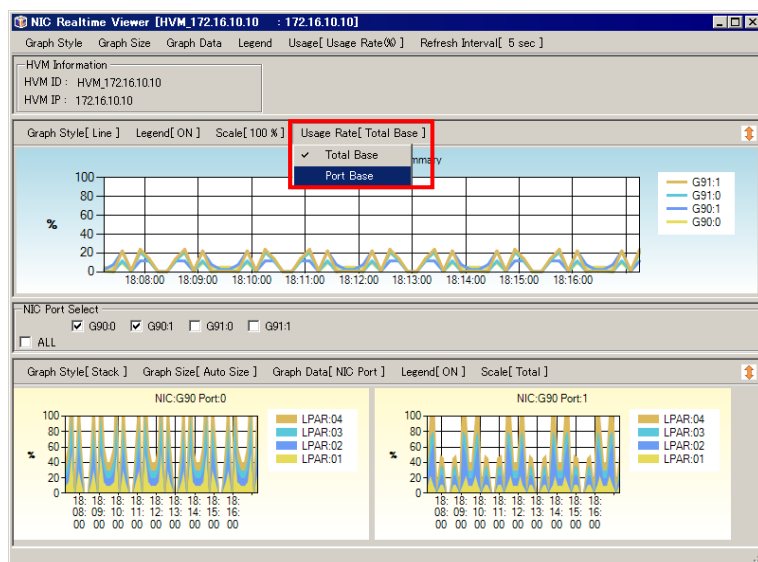
図 4-47 NIC/HBA Realtime Viewer[HVM ID : HVM IP]ウインドウ ([Usage Rate]–[Port Base]選択)
