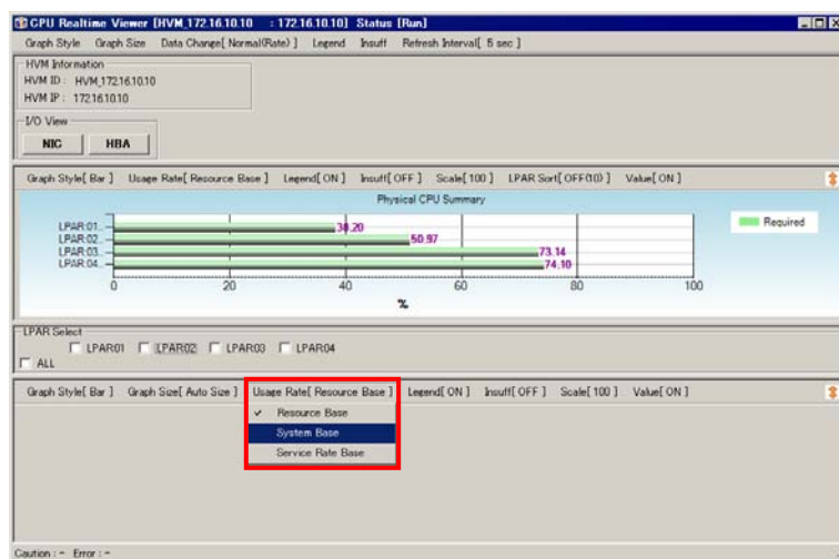
図 4-26 CPU Realtime Viewer[HVM_ID : HVM_IP]ウインドウ ([Usage Rate]-[System Base]選択)
