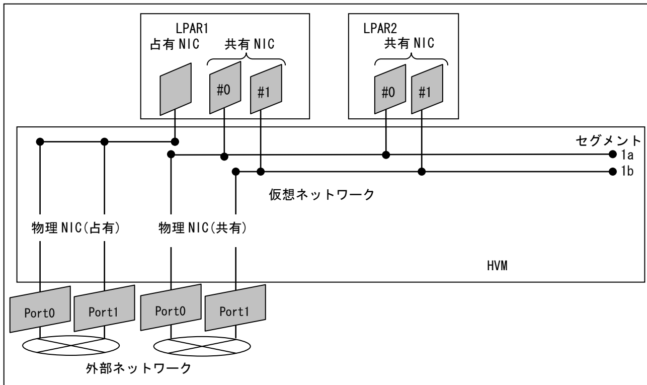
図 2-31 1HVM 上の LPAR への NIC の割り当て
