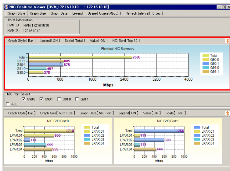
図 4-68 NIC/HBA Realtime Viewer[HVM ID : HVM IP]ウインドウ (Top10 表示)
