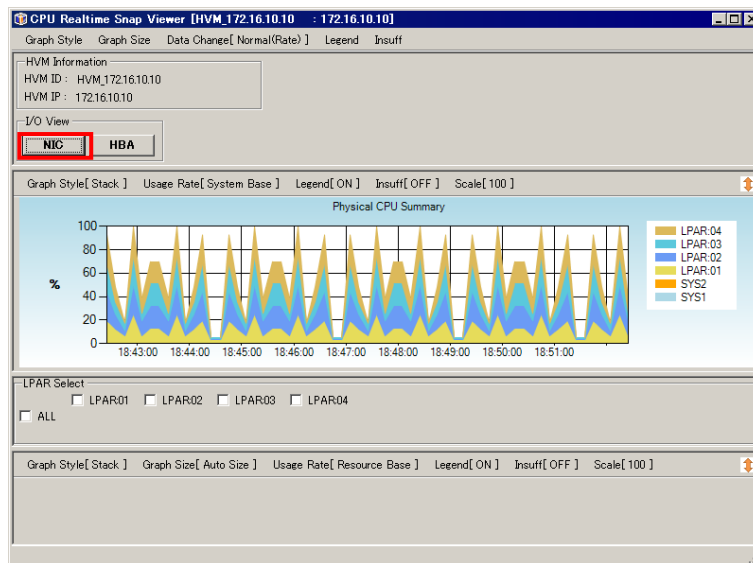
図 4-95 CPU Realtime Snap Viewer[HVM_ID : HVM_IP]ウインドウ
