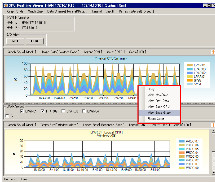
図 4-89 CPU Realtime Viewer[HVM_ID : HVM_IP]ウィンドウ
