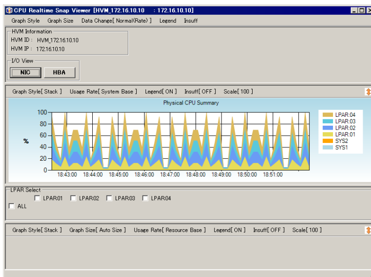
図 4-90 CPU Realtime Snap Viewer[HVM_ID : HVM_IP]ウィンドウ
