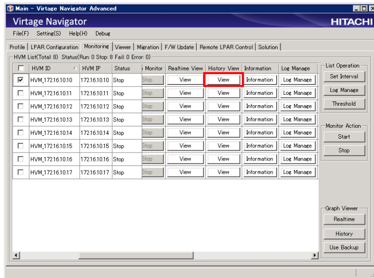
図 3-17 Main ウィンドウ(履歴情報の表示)
