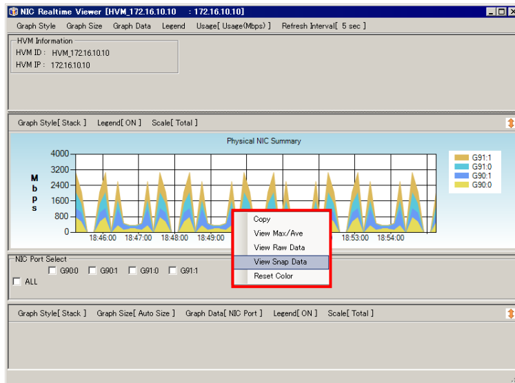
図 4-101 NIC/HBA Realtime Viewer ウィンドウ (View Snap Data 選択)
