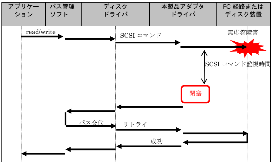
図 18 タイムアウト障害の閾値設定
