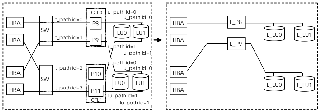
図 2-1 構成図 (2/2)
