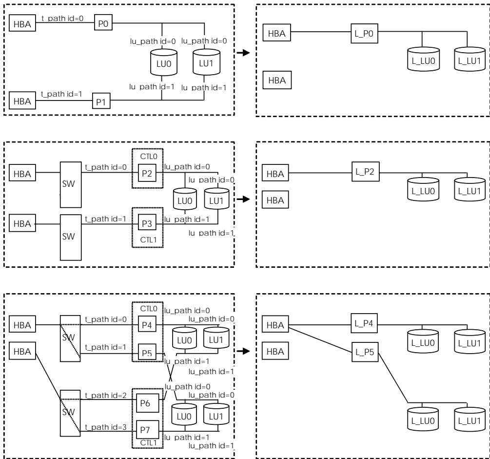
図 2-1 構成図 (1/2)
