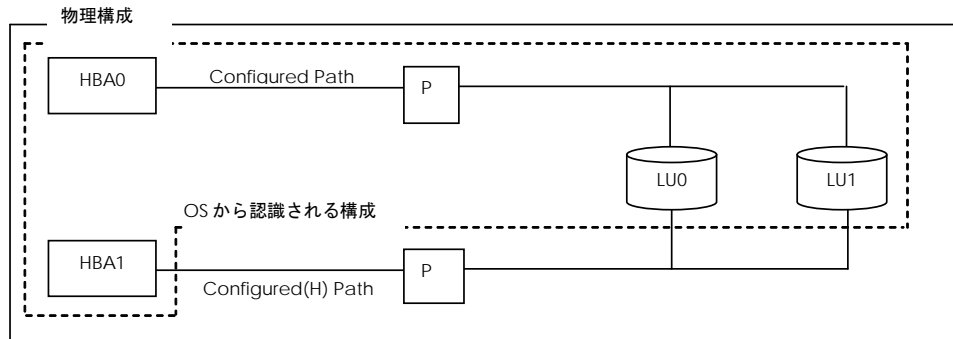
図 2-2 構成例
