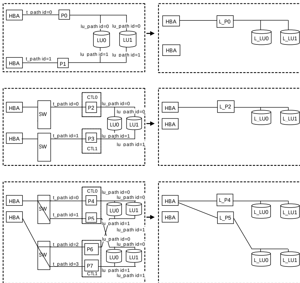
図 2-1 構成図 (1/2)
