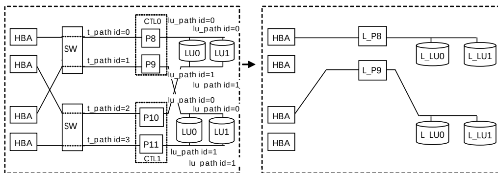
図 2-1 構成図 (2/2)
