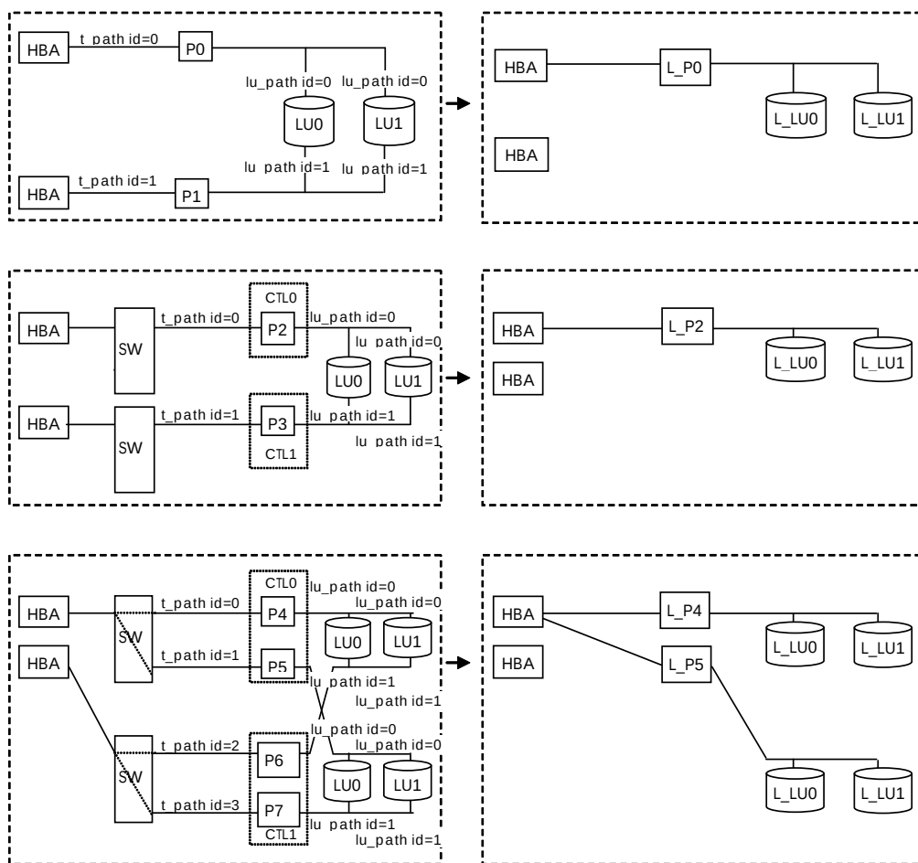
図 2-1 構成図 (1/2)
