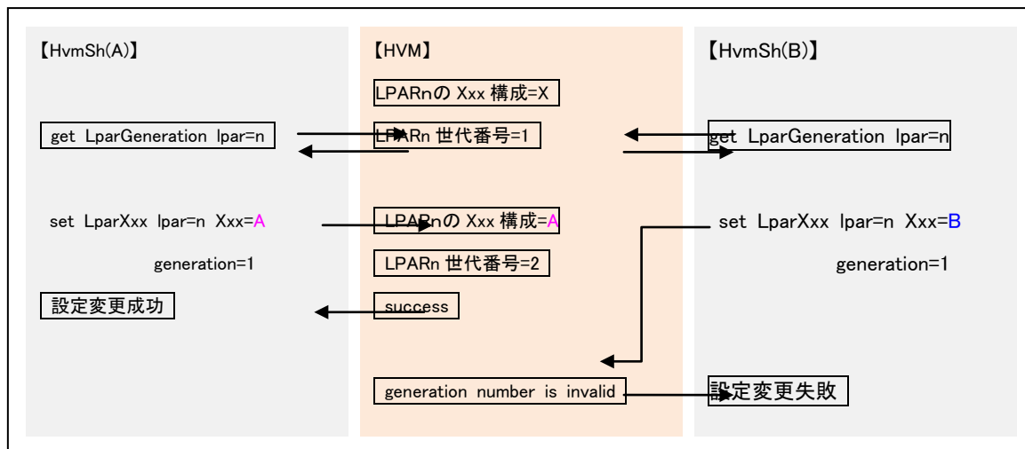
図 7 構成変更競合時の動作例(世代番号を指定した場合)
