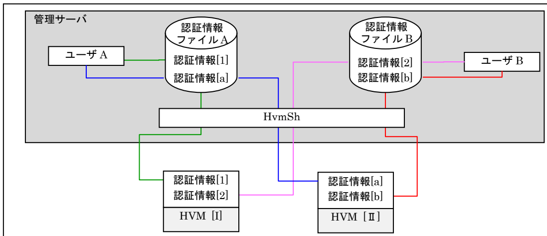
図 4 認証情報ファイルの例
