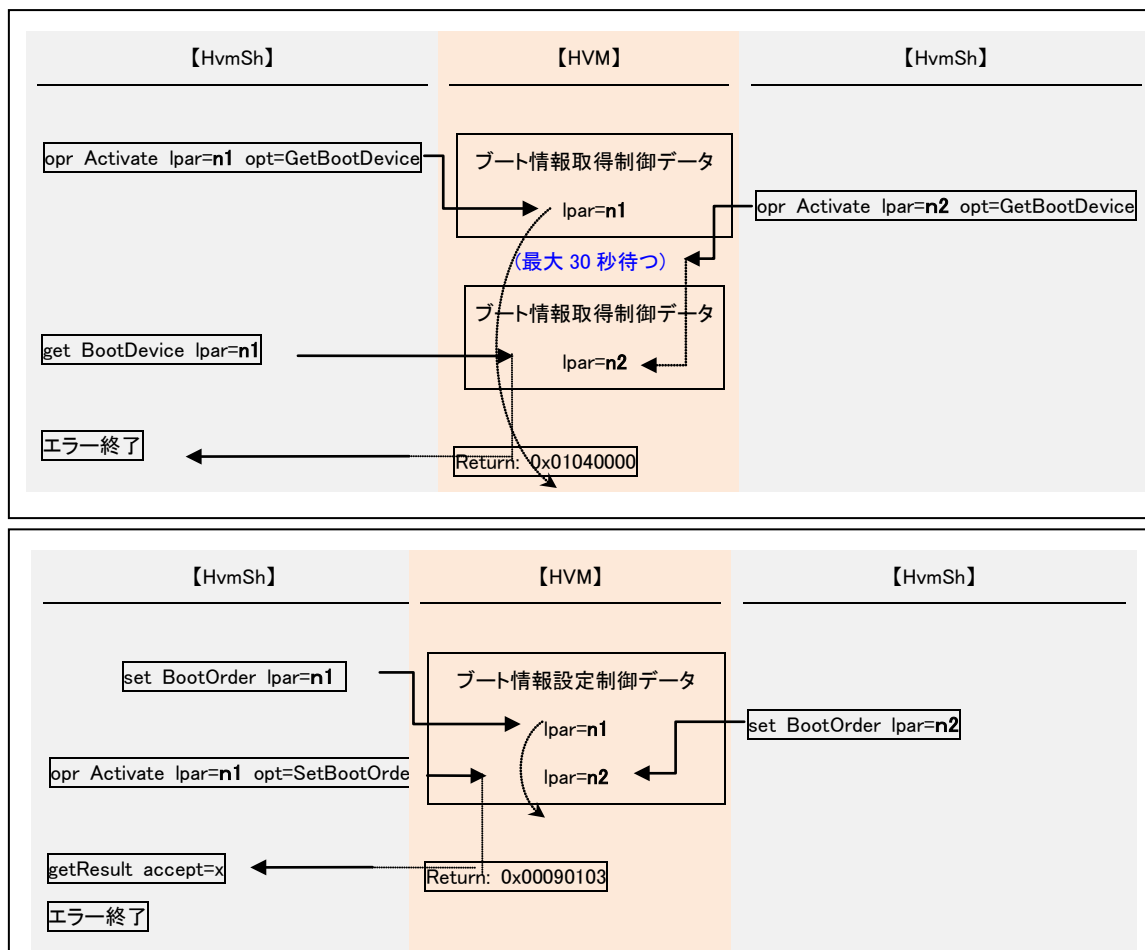
図 6 LPAR のブート情報制御処理の競合例
