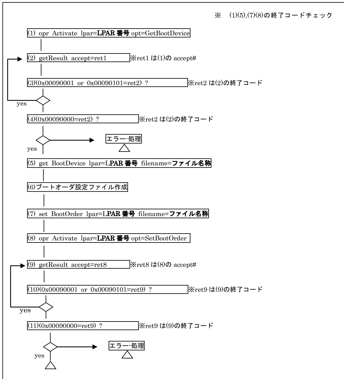
図 5 LPAR のブート情報制御シーケンス
