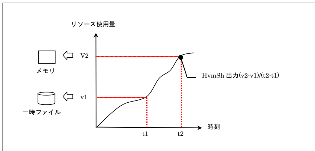
図 4 HvmSh コマンドの統計情報採取
