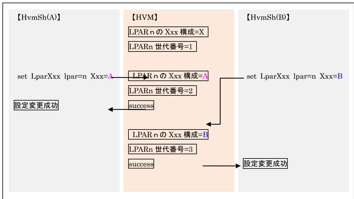
図 8 構成変更競合時の動作例(世代番号を指定しない場合)
