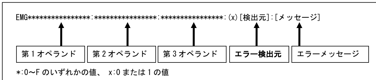
図 4-2 エラーメッセージのフォーマット
