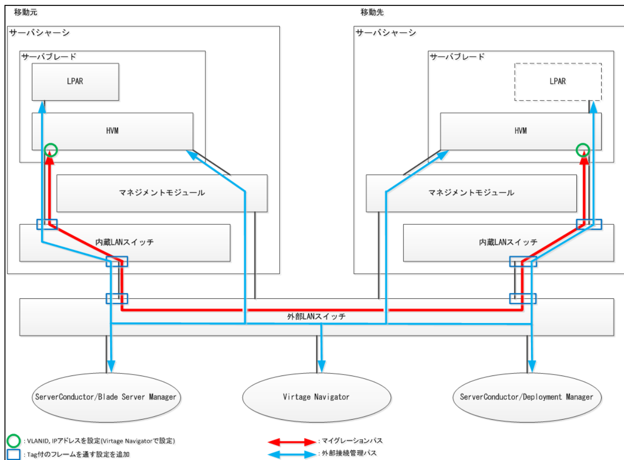
図 2-10 ネットワークの推奨構成
