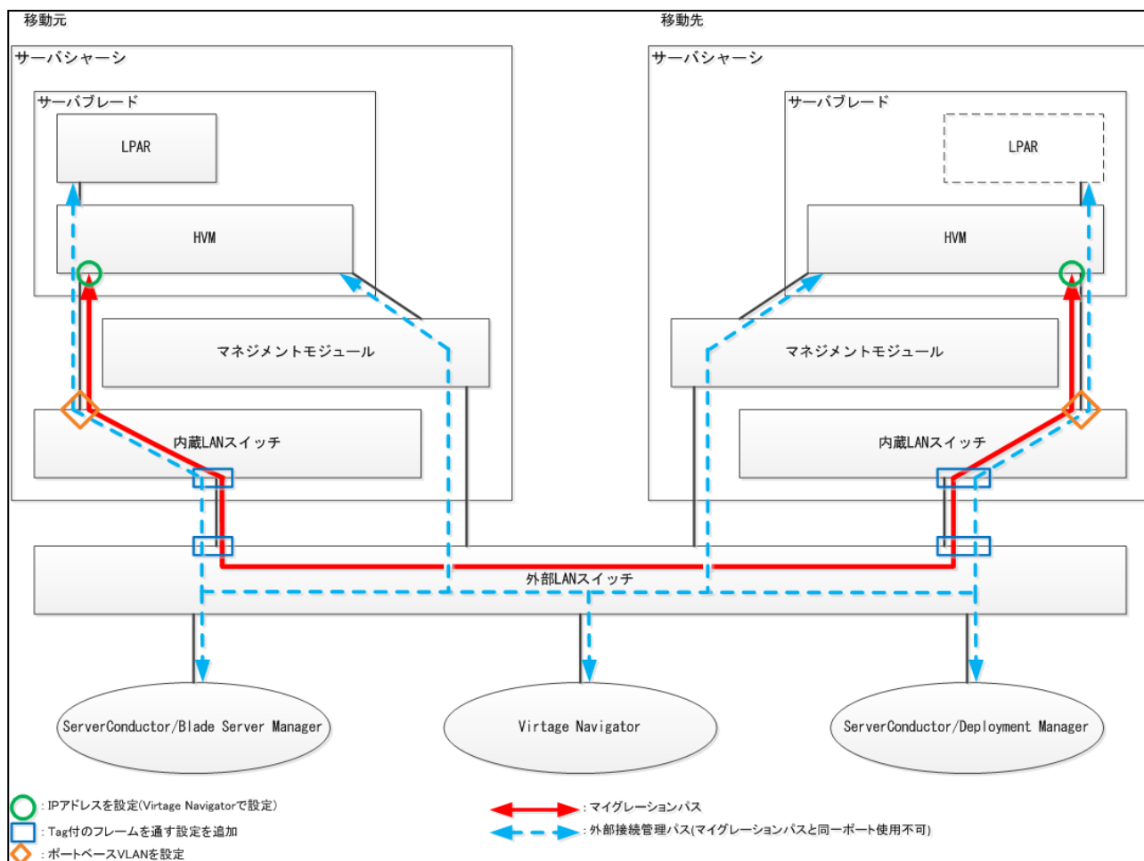
図 2-11 ネットワークの推奨構成
