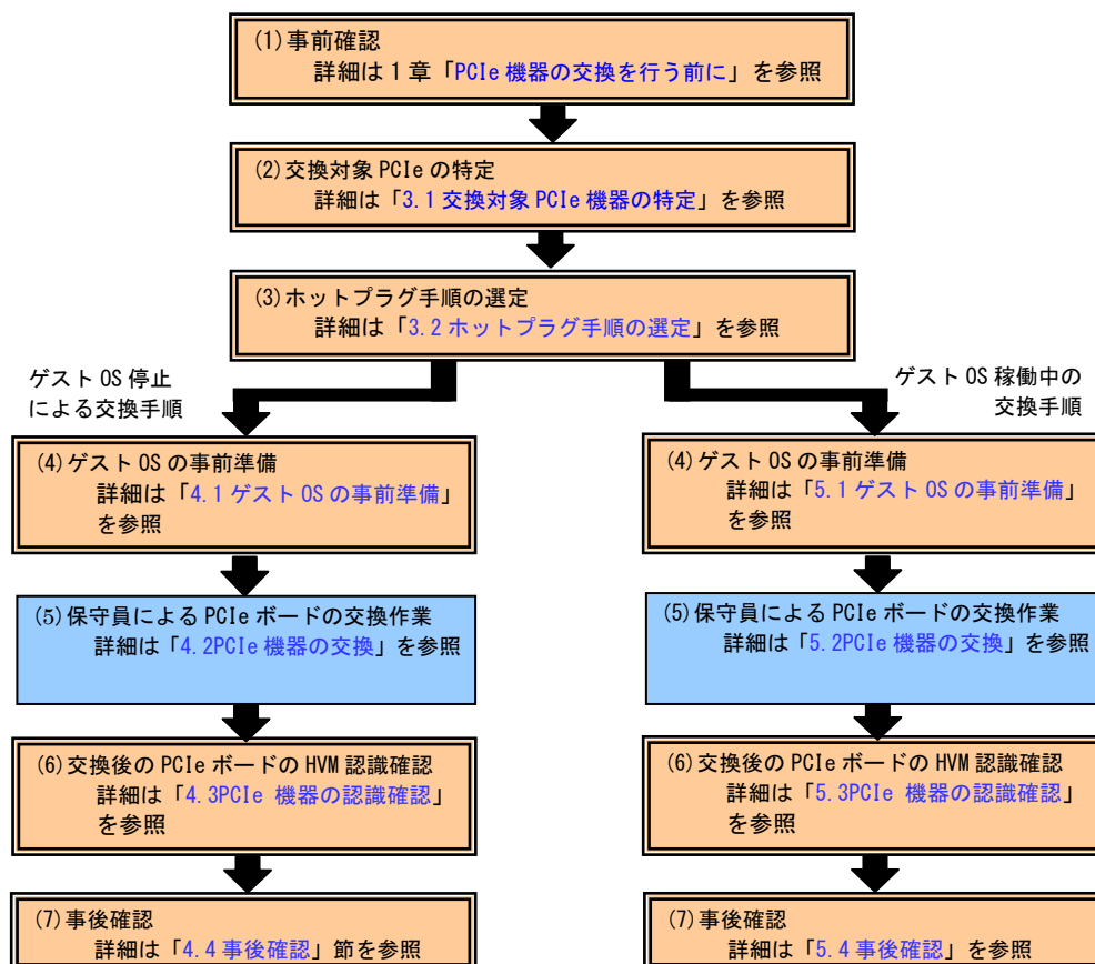
図 2 PCIe ボードの交換手順
