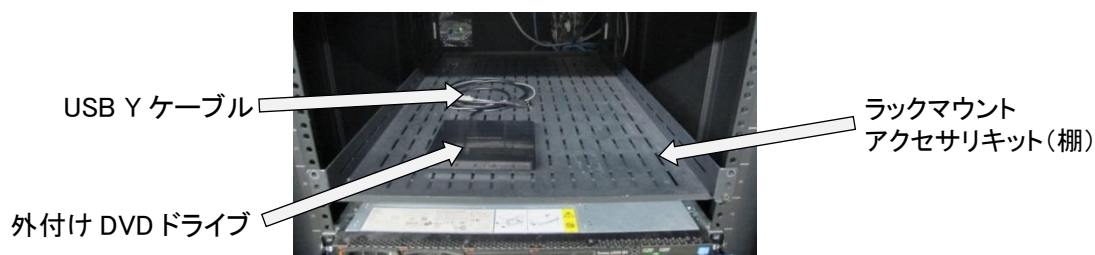
ラックマウントアクセサリキットへの搭載図
