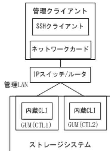
図 75 SSH クライアントから内蔵 CLI を使用する場合のシステム構成
