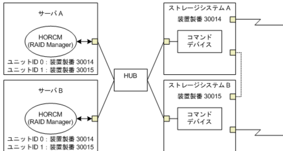
図 8 複数台のストレージシステムがある構成とユニット ID
