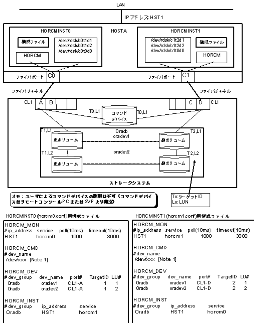
図 23 2 インスタンス用 TrueCopy 構成例
