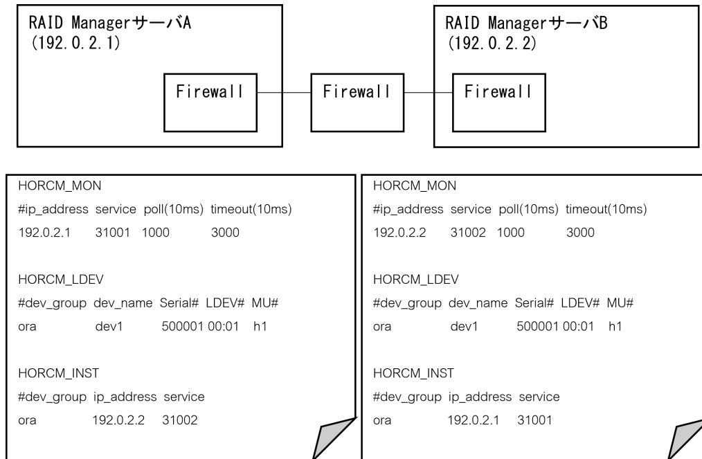
図 11 RAID Manager サーバおよびネットワークとファイアウォールの構成例
