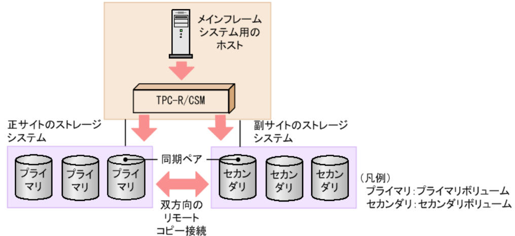
図 3 TPC-R/CSM を使用した、TC-MF 同期ペアのプライマリボリュームとセカンダリボリュームの交換
