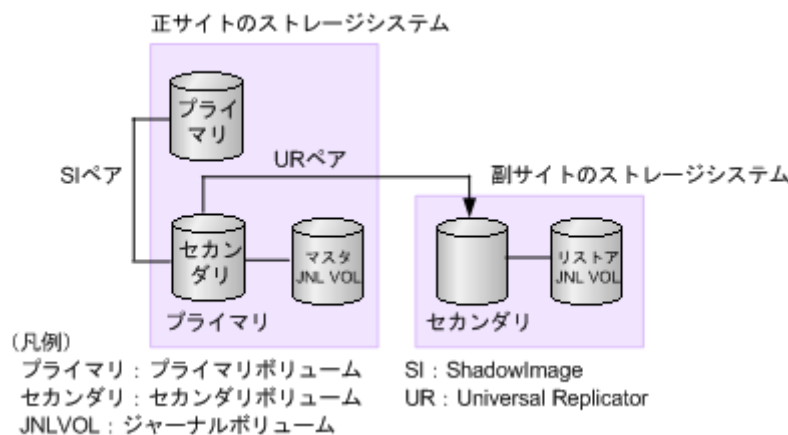
図 18 ShadowImage プライマリボリュームの復旧手順 (9)
