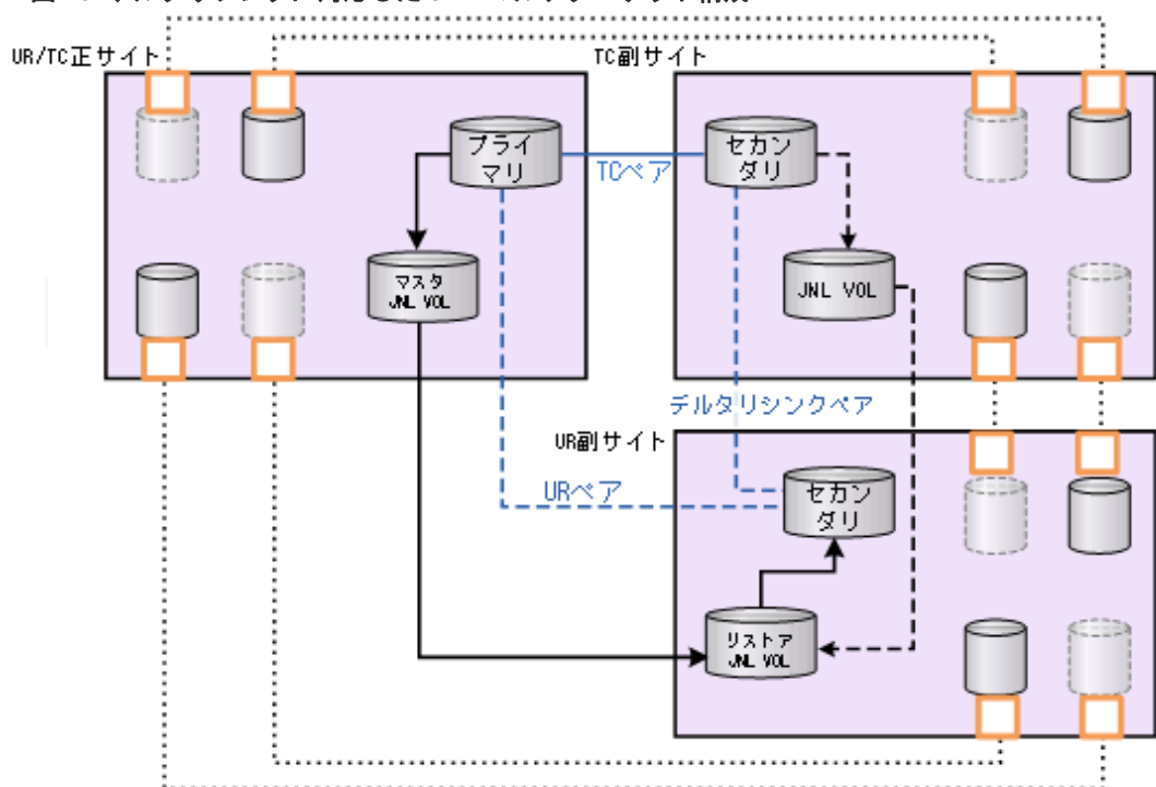
図 20 デルタリシンクに対応した 3DC マルチターゲット構成
