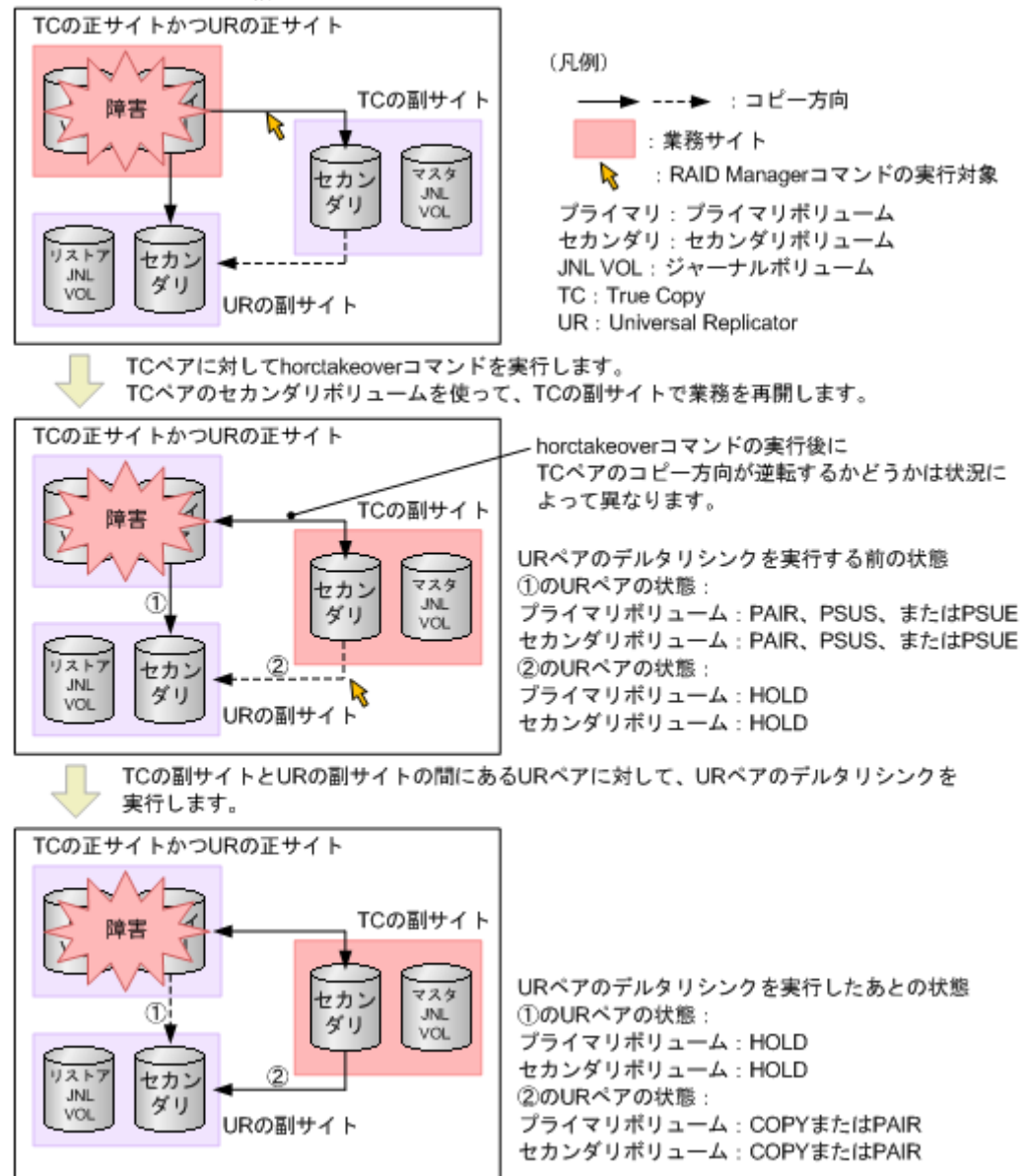
図 5 正サイトでの障害からの復旧（デルタリシンクを実行した場合）
