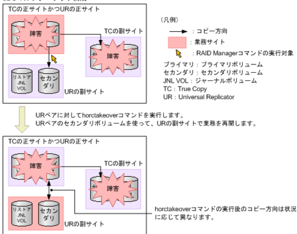
図 7 正サイトおよび TrueCopy の副サイトでの障害からの復旧
