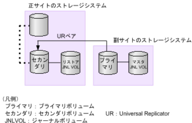
図 11 ShadowImage プライマリボリュームの復旧手順 (2)
