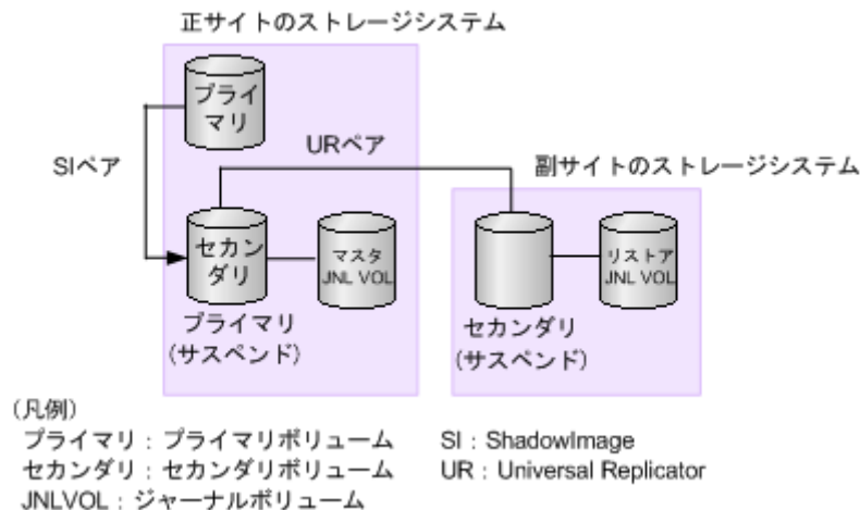
図 16 ShadowImage プライマリボリュームの復旧手順 (7)
