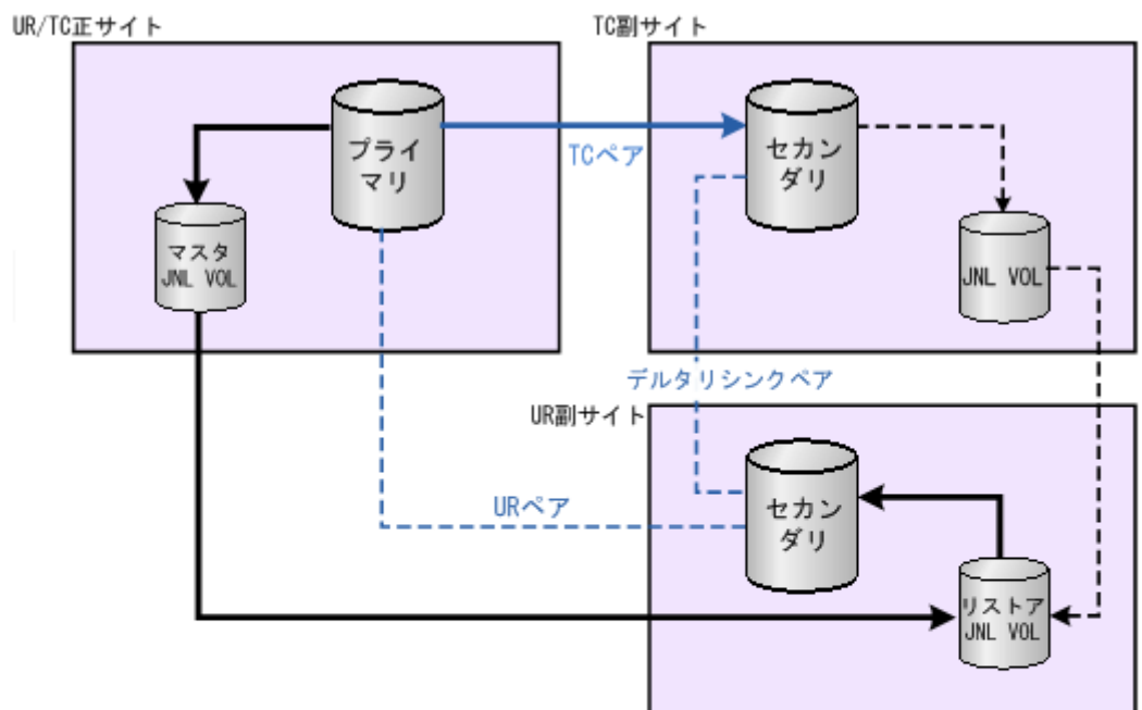
図 21 デルタリシンク用 3DC マルチターゲット構成
