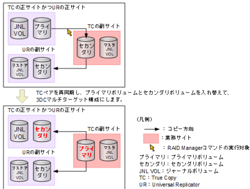
図 2 正サイト復旧後に 3DC マルチターゲット構成にする
