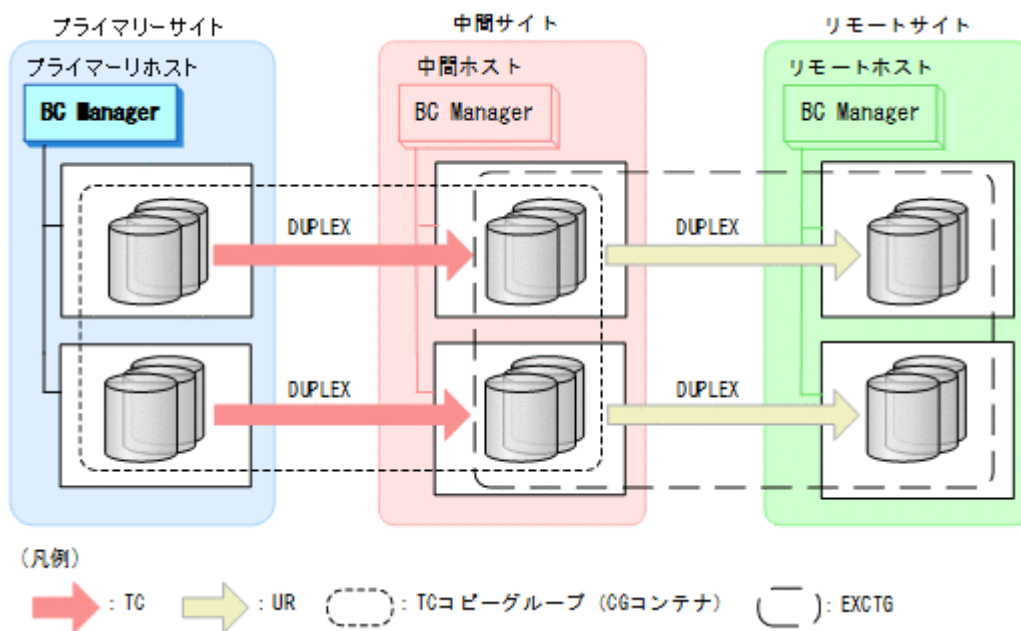
図 29 4x4 Cascade 構成の例
