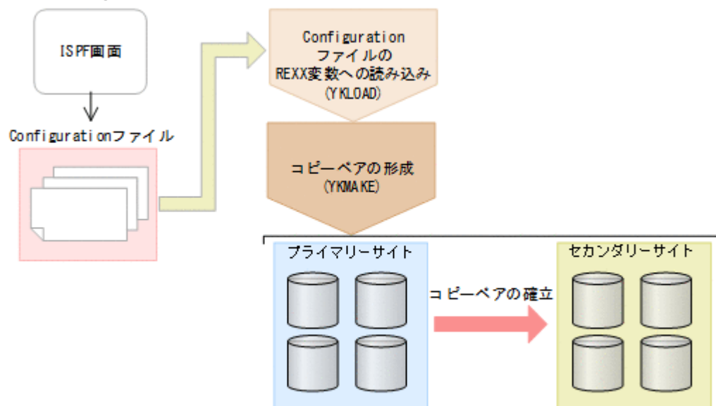
図 139 Configuration ファイルの利用
