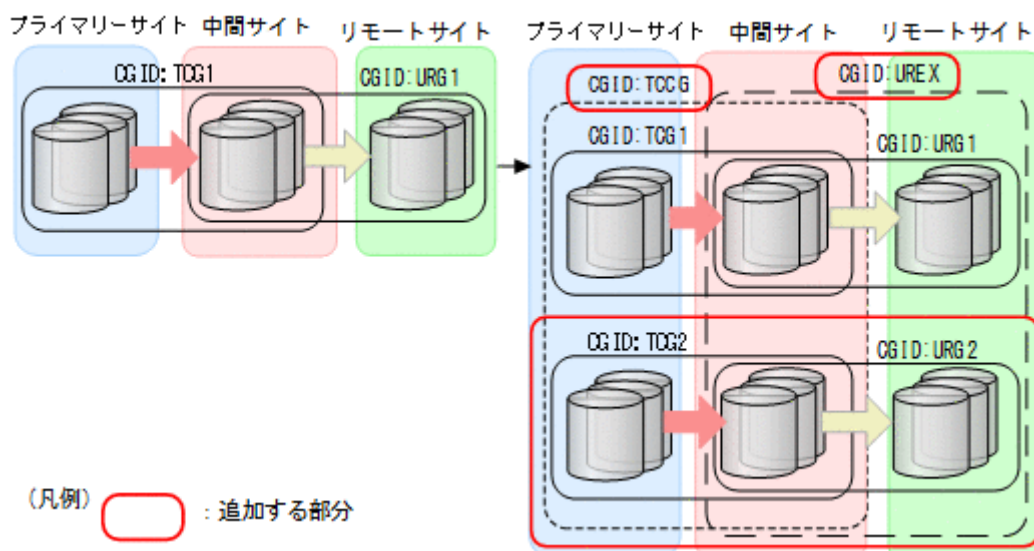
図 125 3DC Cascade (TCxUR)構成を 4x4x4 Cascade 構成に拡張する場合のコピーグループ例
