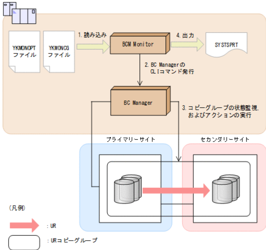
図 168 BCM Monitor の動作概要
