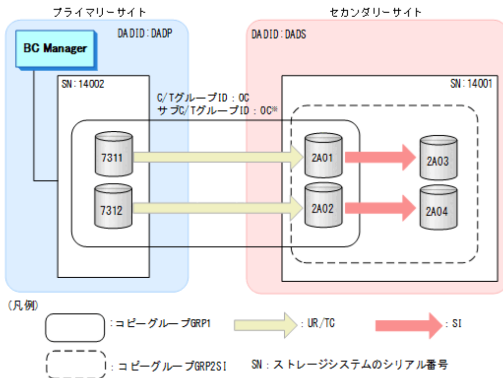
図 155 CG コンテナではないコピーグループの定義例
