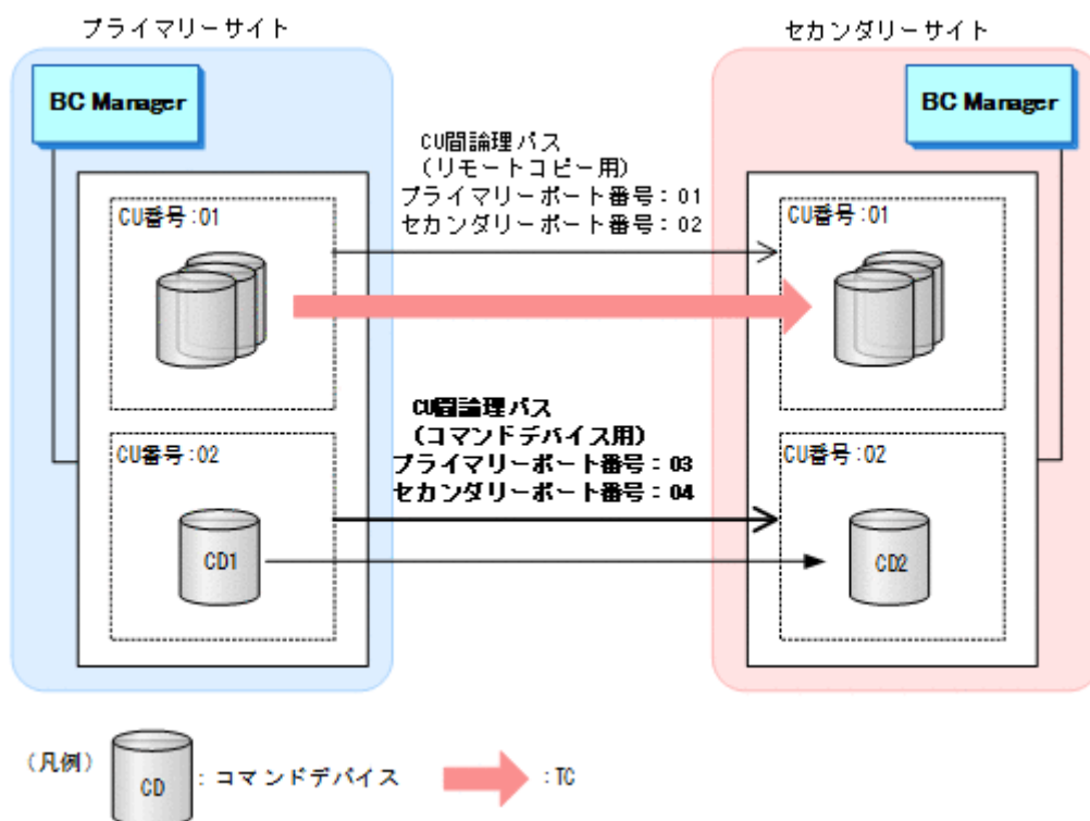
図 98 TC コピーグループの構成例
