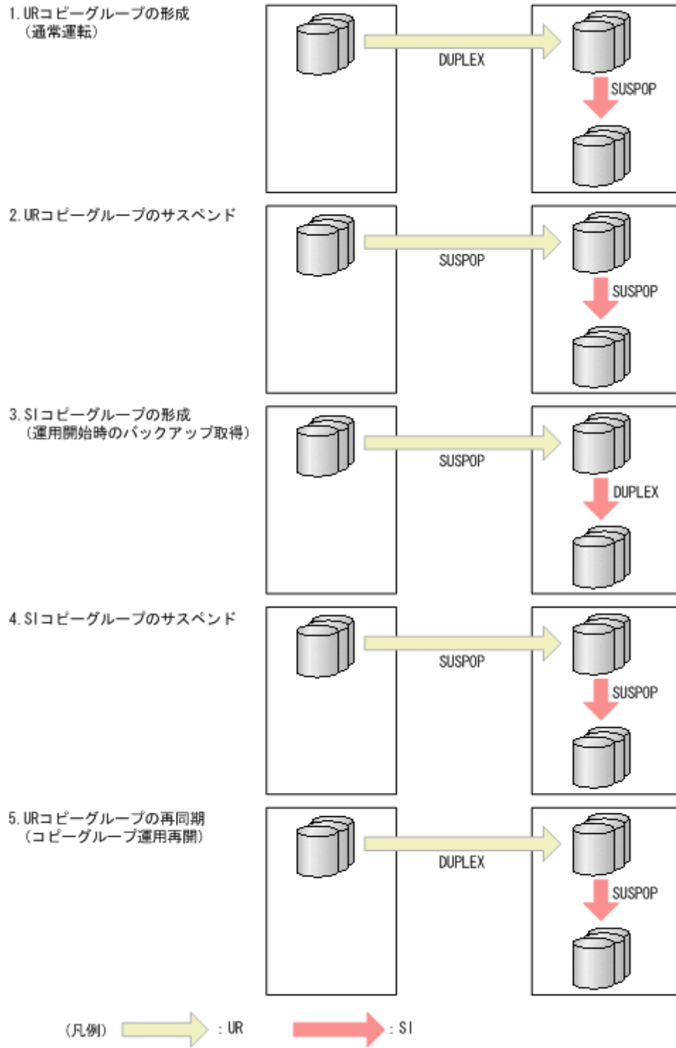
図 141 コピーグループを形成する手順
