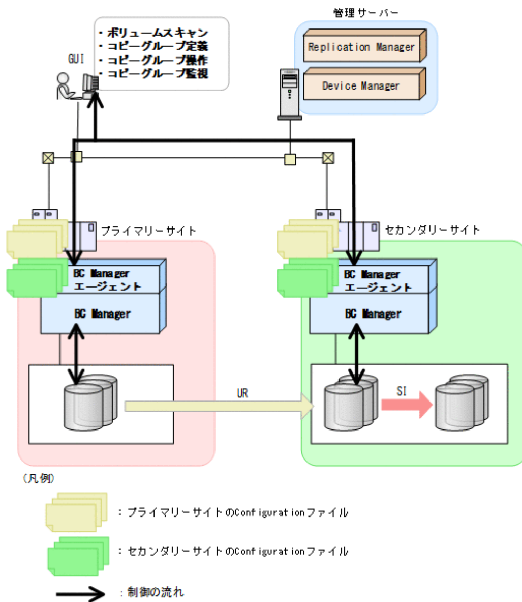
図 175 Replication Manager と連携する運用の概要
