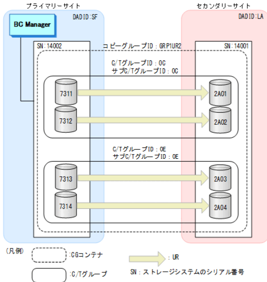
図 158 CG コンテナの定義例
