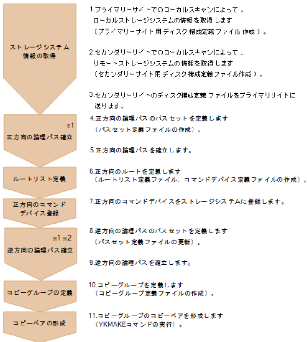
図 104 2DC 構成をプライマリーサイトで運用するための定義フロー（ケース A）
