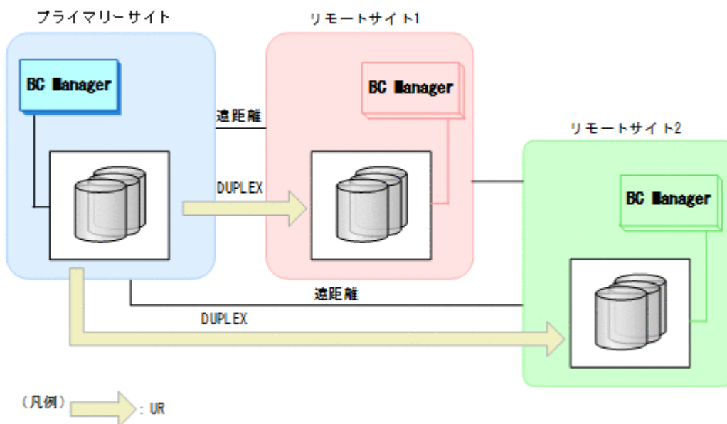
図 21 3DC Multi-Target (URxUR)構成の例
