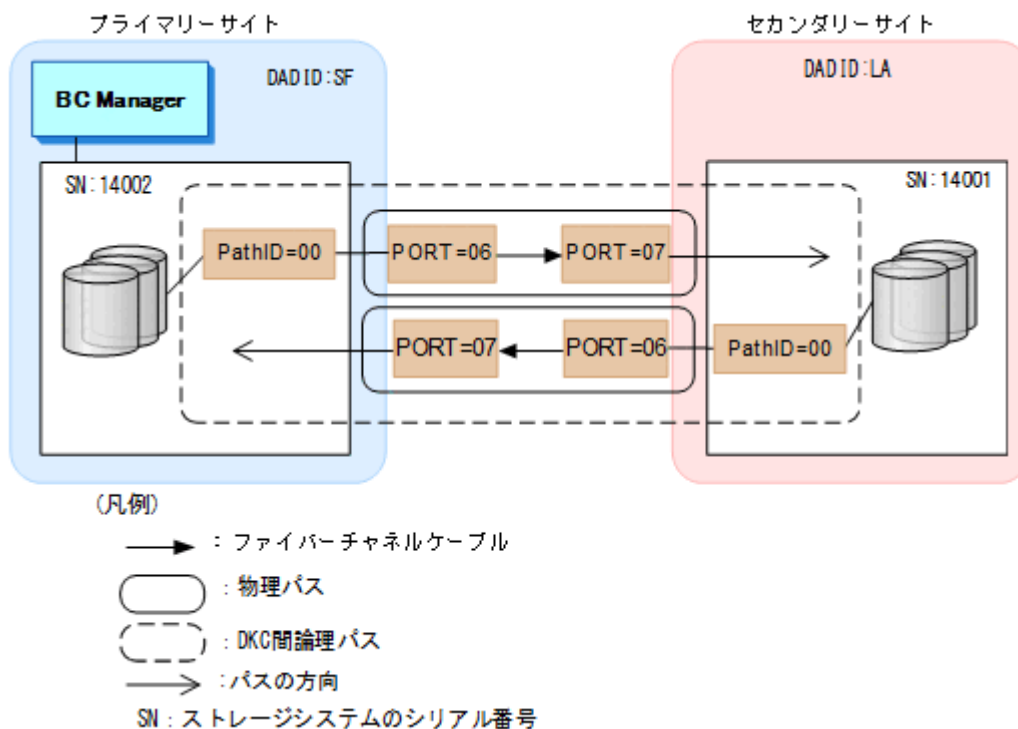
図 149 DKC 間論理パスの定義例
