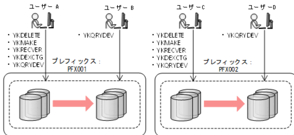
図 84 プレフィックスおよびコマンドごとに操作するユーザーを分ける例
