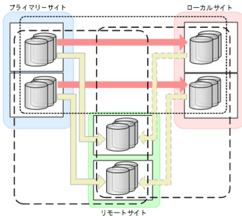
図 127 4x4x4 デルタリシンのコピーグループに関する構成例 (2x2x2)
