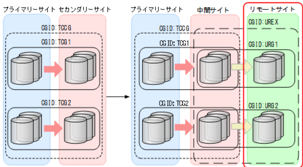
図 123 UR コピーグループを追加して 4x4 Cascade 構成に拡張する場合のコピーグループ例
