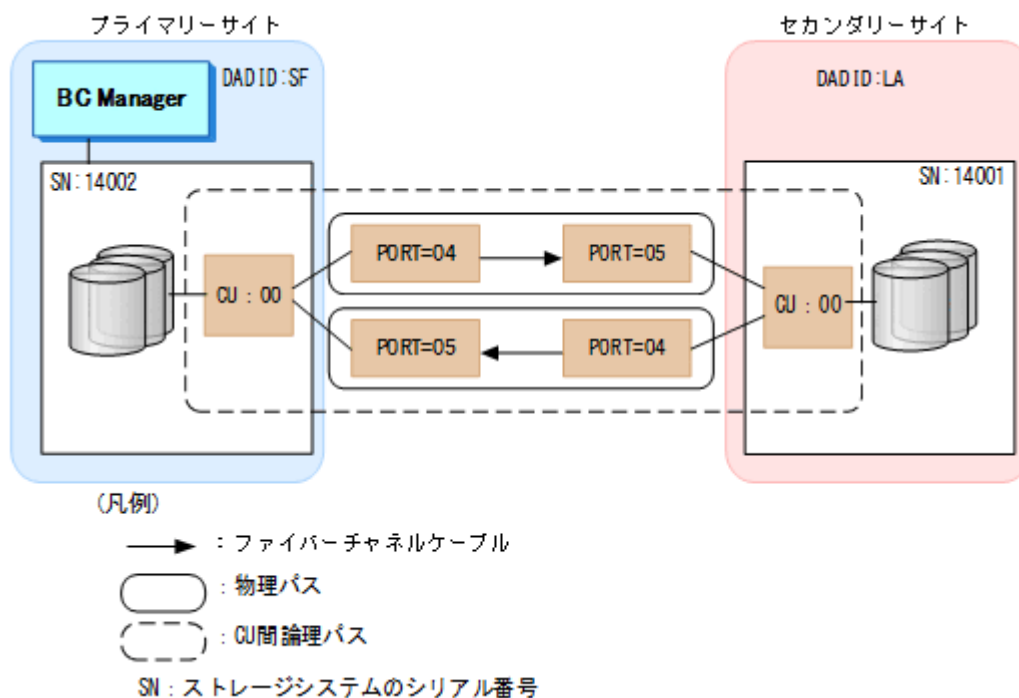
図 150 CU 間論理パスの定義例
