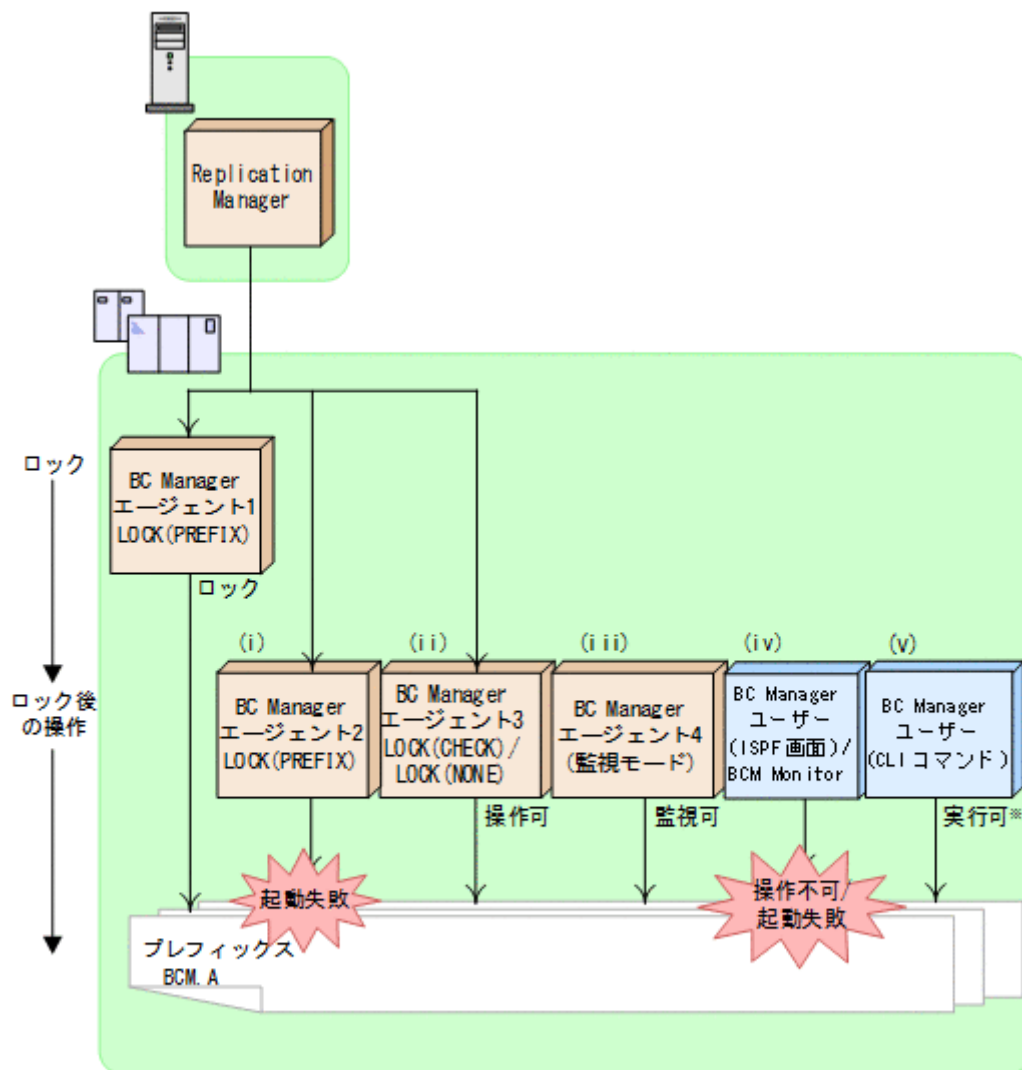
図 177 BC Manager エージェントがすでに起動されていた場合
