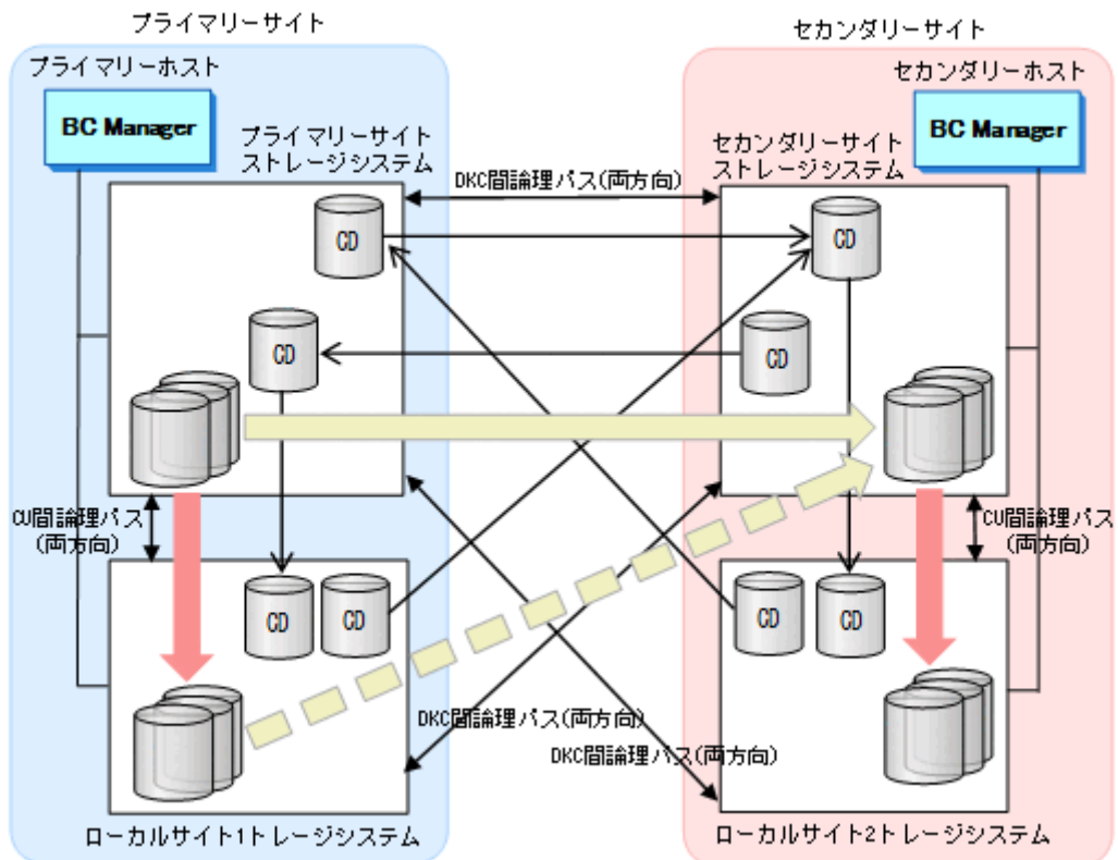
図 135 Multi-Site Multi-Region (4DCz)構成の構成例
