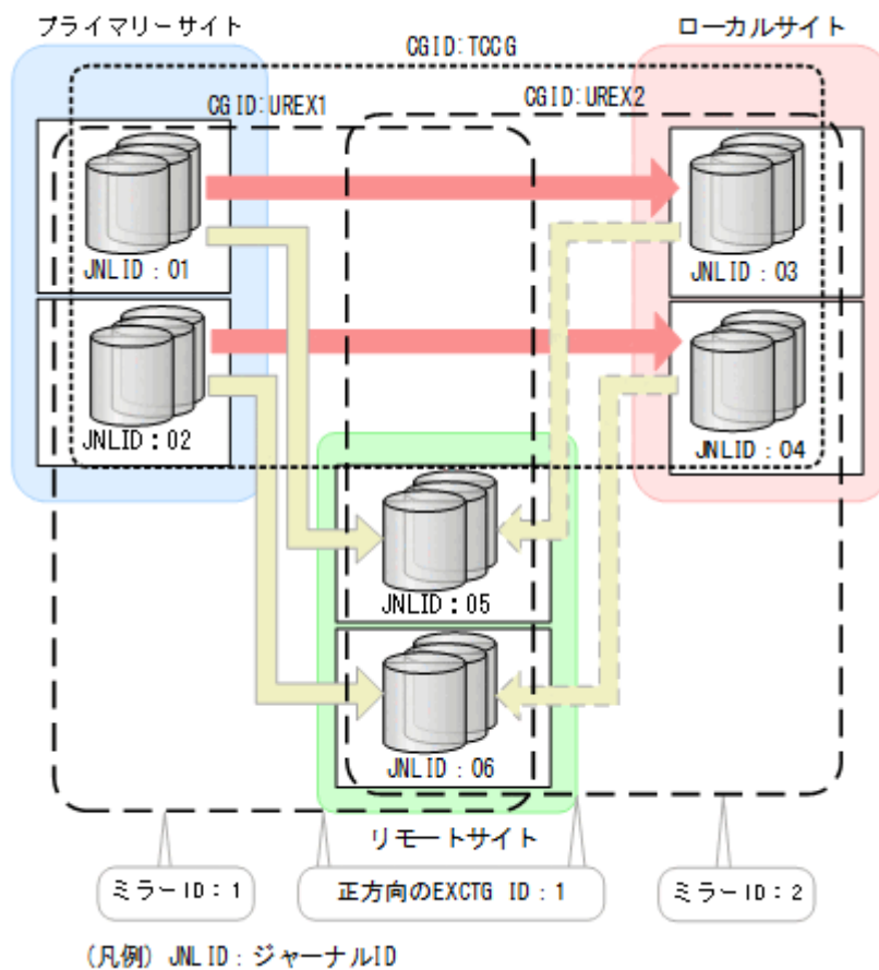
図 128 4x4x4 デルタリシンのコピーグループ
