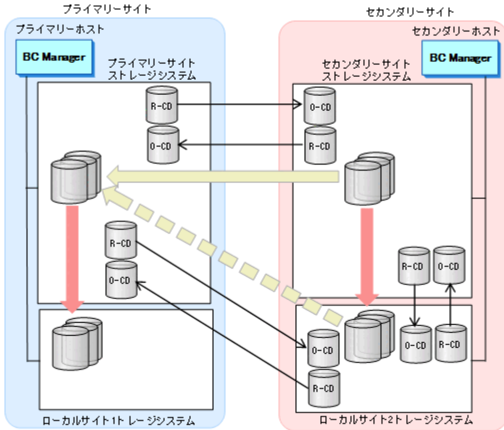
図 138 4DC 構成のリモートコマンドデバイスと Open 用コマンドデバイスの構成例
