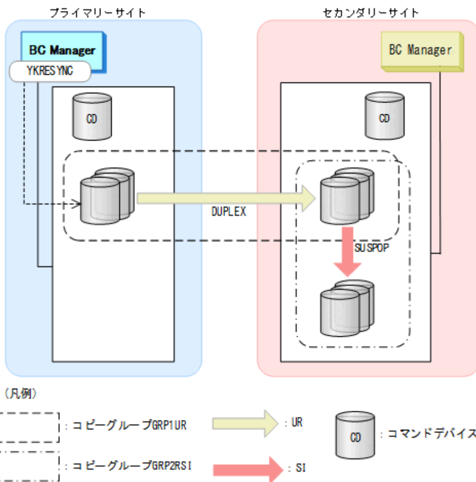
図 160 コピーグループの構成例
