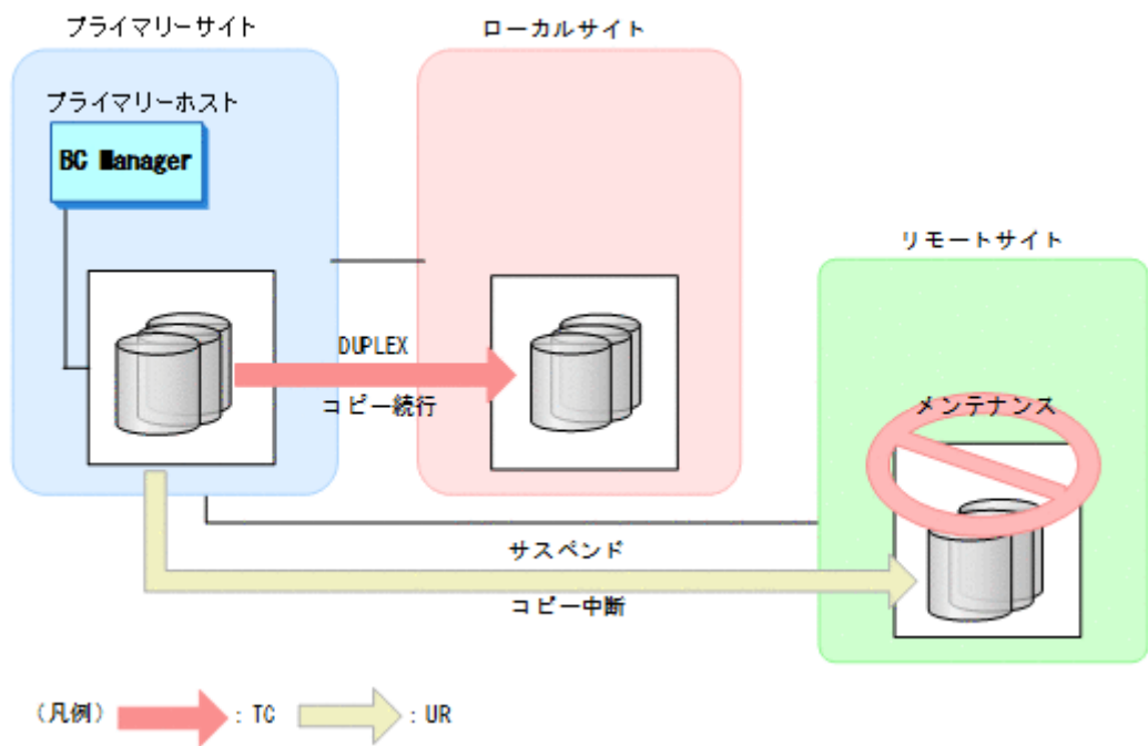
図 19 リモートサイトのストレージシステムメンテナンスの場合 (3DC Multi-Target (TCxUR) 構成)
