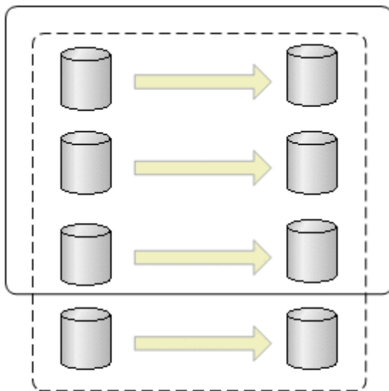
図 48 コピーグループ内に C/T グループの一部のボリュームを含む場合 (SI/TC/UR)
