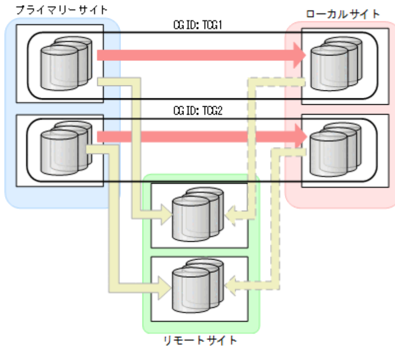
図 129 4x4x4 デルタリシンのコピーグループ (TCGG の障害時操作)
