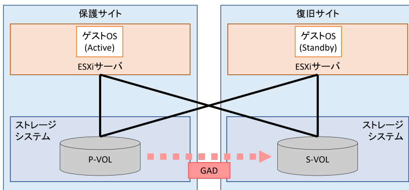
図 77 GAD を使用する構成
