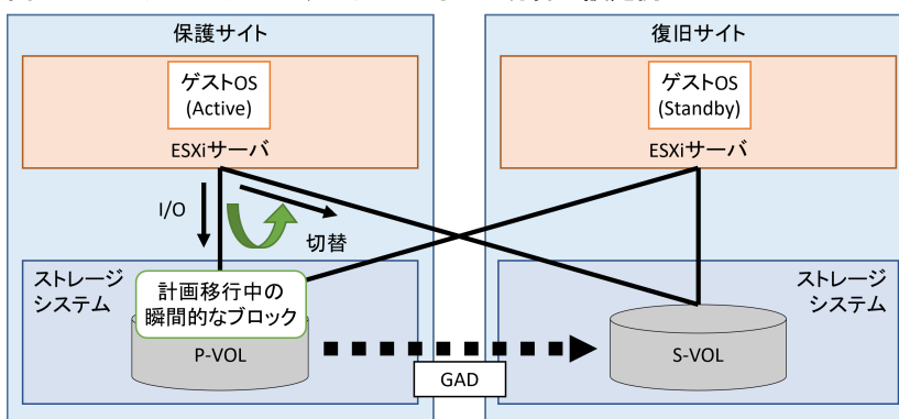
図 78 マルチパスソフトウェアによる I/O 切替の設定例
