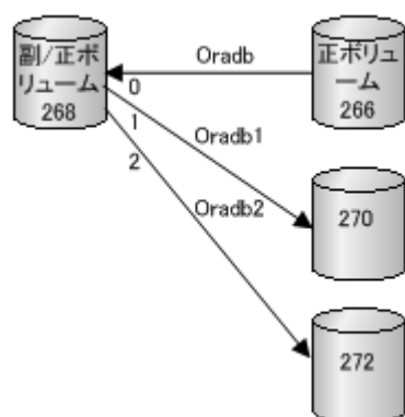
図 32 HORCMINST1 -g の Pairedisplay
