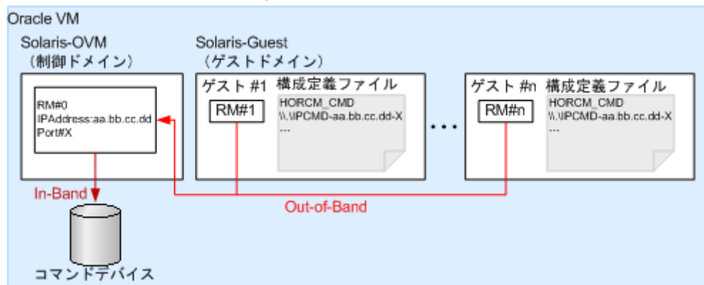
図 4 Oracle VM 上の RAID Manager 構成
