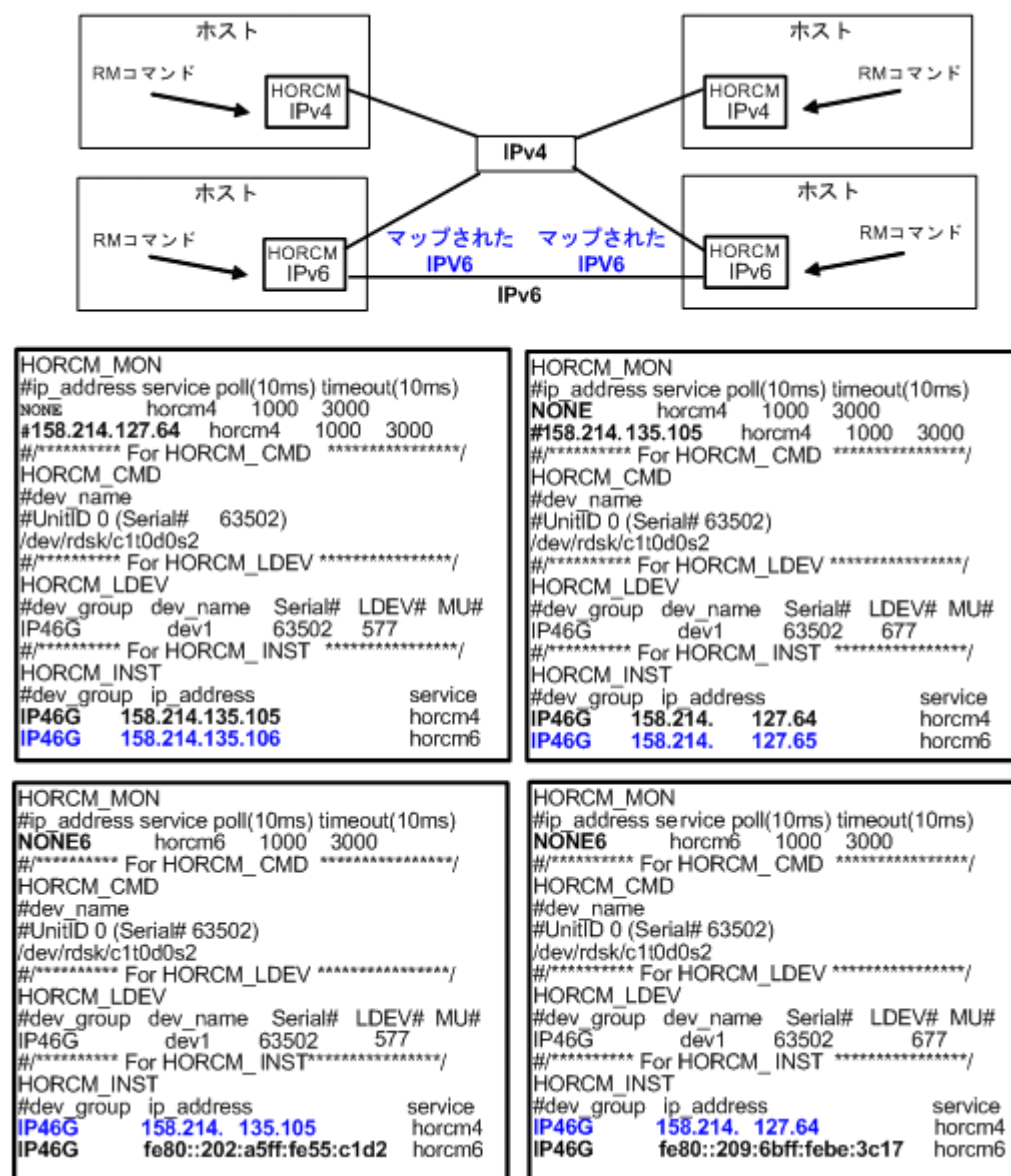
図 20 IPv4 と IPv6 混在のネットワーク構成
