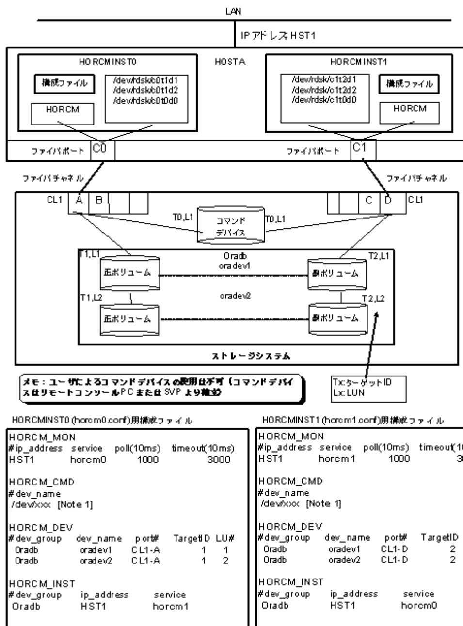
図 23 2 インスタンス用 TrueCopy 構成例
