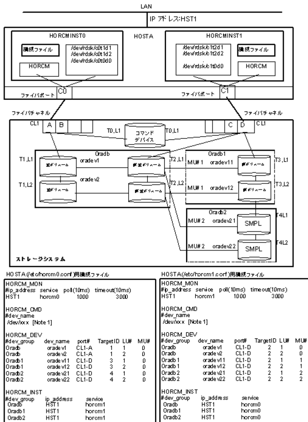
図 26 Cascade Pairs を伴う ShadowImage の構成例
