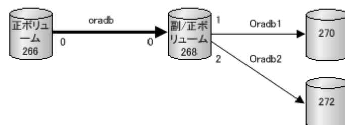
図 31 HORCMINST0 の Pairedisplay -g
