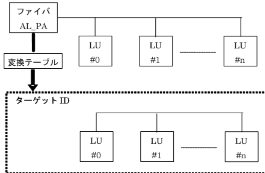
図 12 Fibre アドレス変換の例
