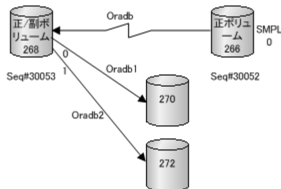
図 36 HOST2 (HORCMINST) の TrueCopy 用 Pairedisplay
