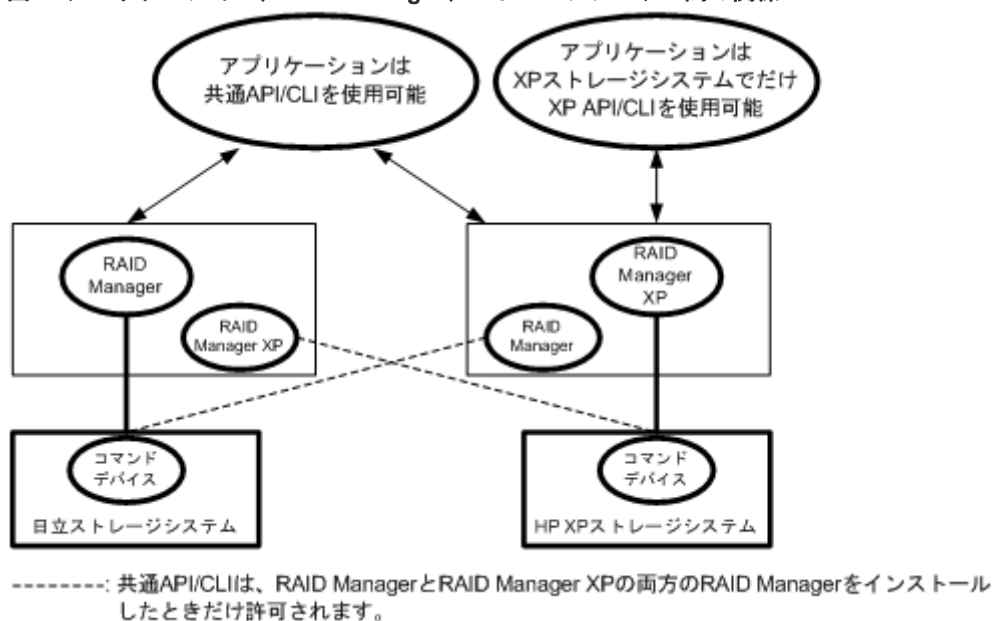
図 6 アプリケーション、RAID Manager、ストレージシステム間の関係
