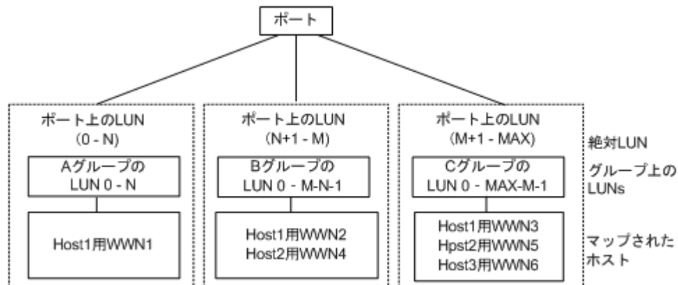
図 13 LUN 構成
