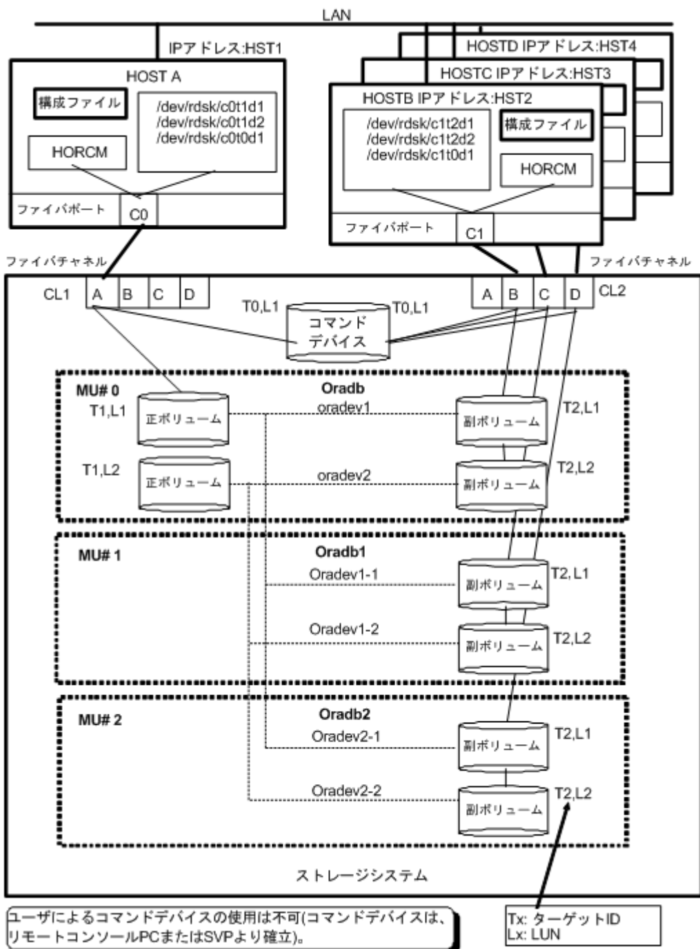
図 24 ShadowImage 構成例 (次ページに続く)
