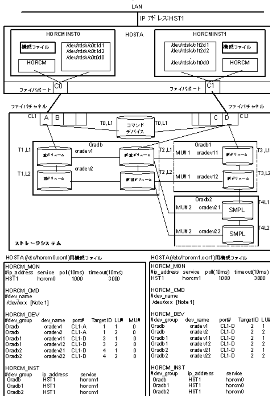
図 26 Cascade Pairs を伴う ShadowImage の構成例
