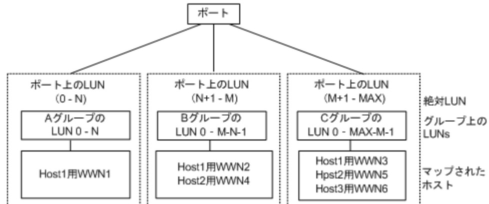
図 13 LUN 構成
