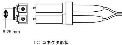
図 7 ケーブル側コネクタ形状
