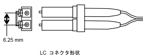
図 7 ケーブル側コネクタ形状
