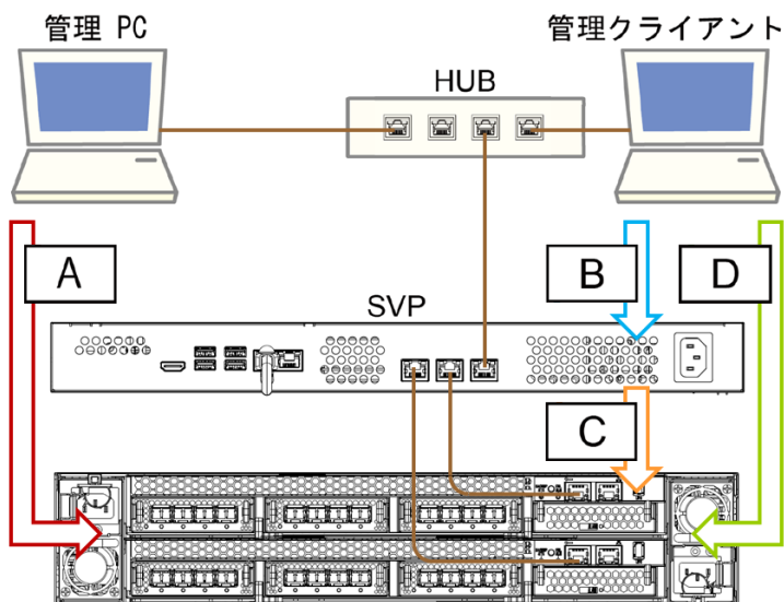
図 3 SSL 通信の接続経路 (VSP E390、VSP E590、VSP E790 および VSP E1090 の場合)
