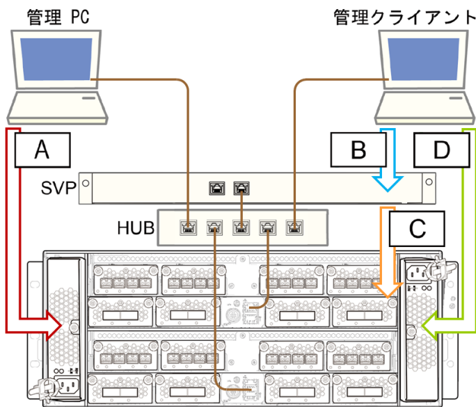
図 4 SSL 通信の接続経路 (VSP E390、VSP E590、VSP E790 および VSP E1090 以外の場合)
