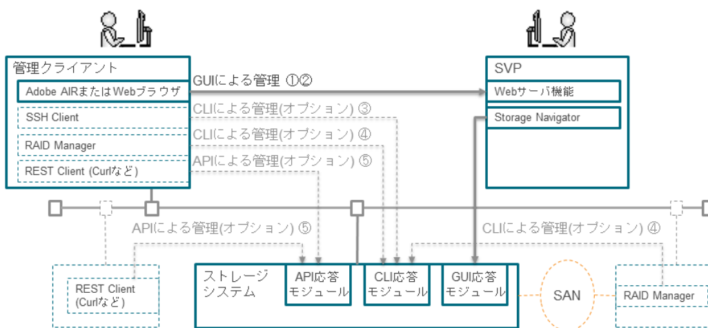
図 2 Storage Navigator 利用の構成
