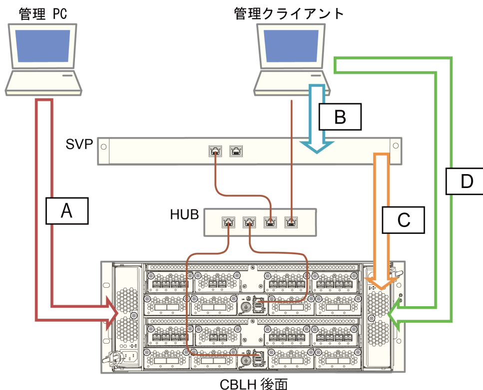
図 3 SSL 通信の接続経路
