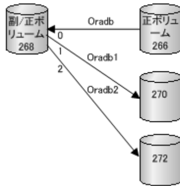
図 B-19 : HORCMINST1 -g の Pairedisplay
