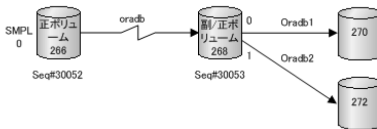
図 B-22 : HOST1 の TrueCopy 用 Pairdisplay
