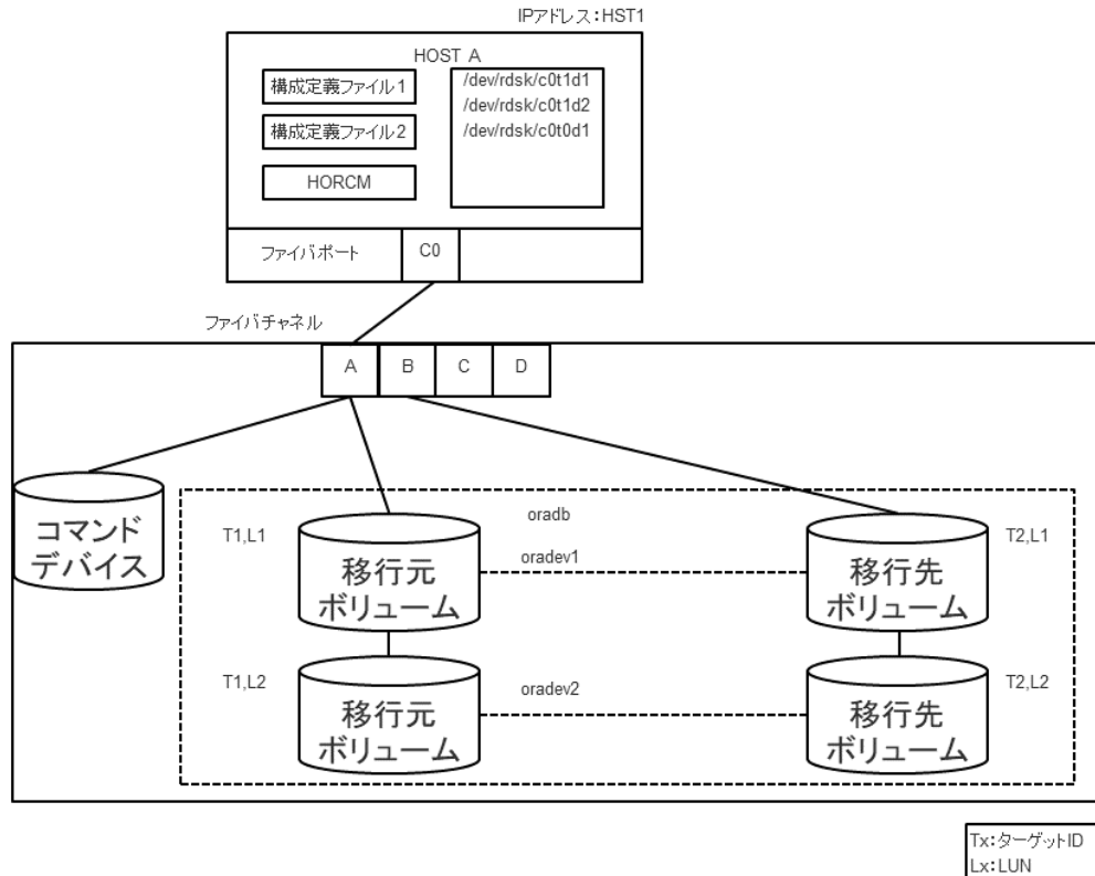
図 B-15 : Volume Migration 構成例
