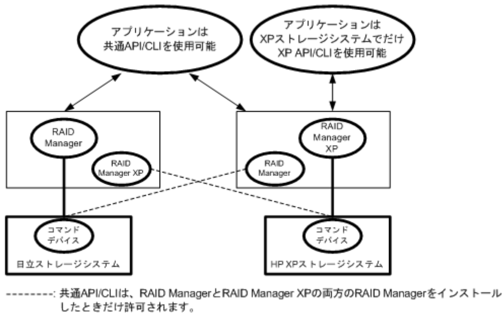
図 1-6 : アプリケーション、RAID Manager、ストレージシステム間の関係
