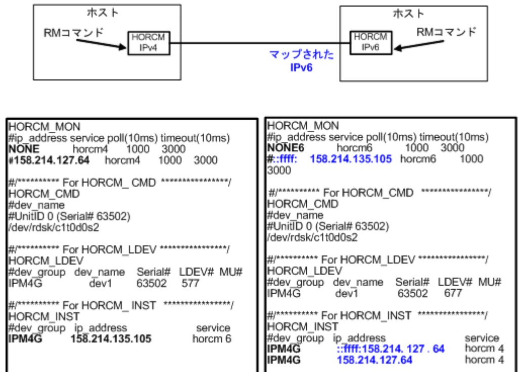
図 B-6 : IPv4 mapped IPv6 用のネットワーク構成
