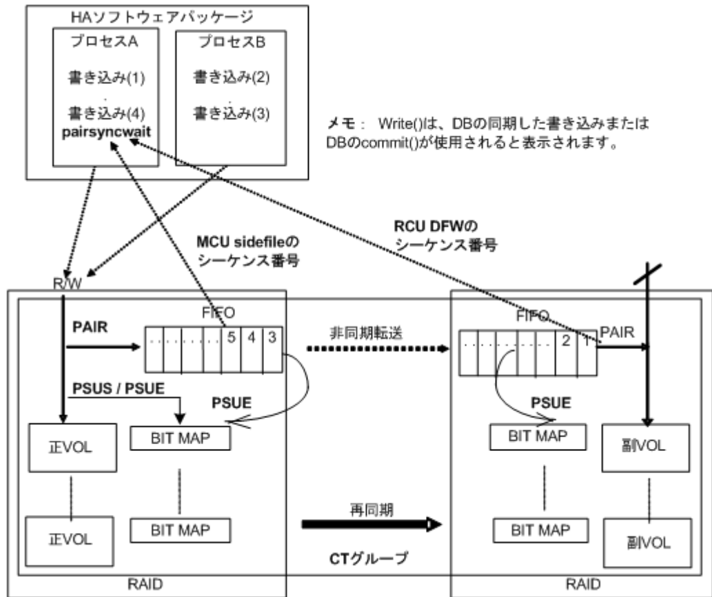
図 19 TrueCopy Async/Universal Replicator の同期
