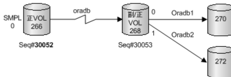
図 17 pairdisplay -m オプション例
