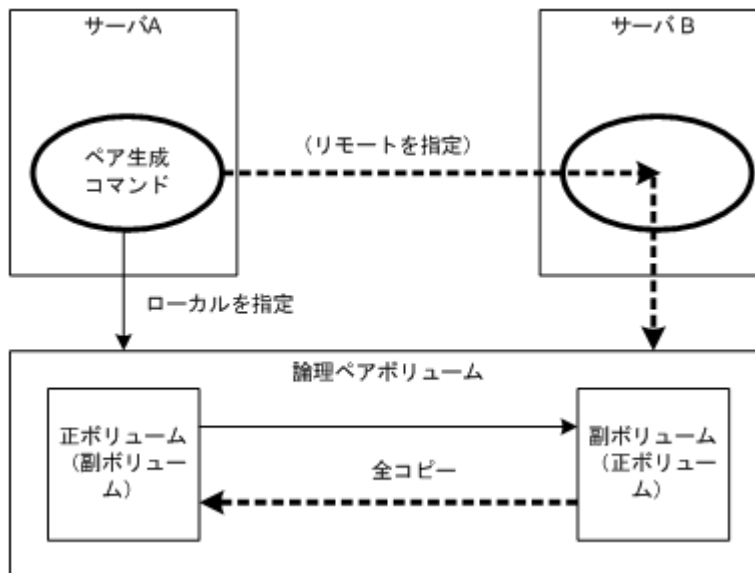
図 3 ペア生成
