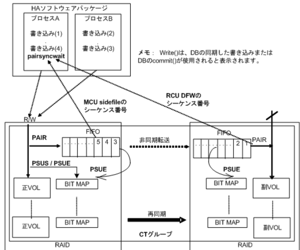
図 2-17 : TrueCopy Async/Universal Replicator の同期
