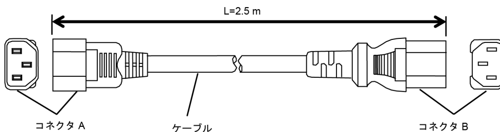
図 17 200V 電源ケーブル (J2H)
