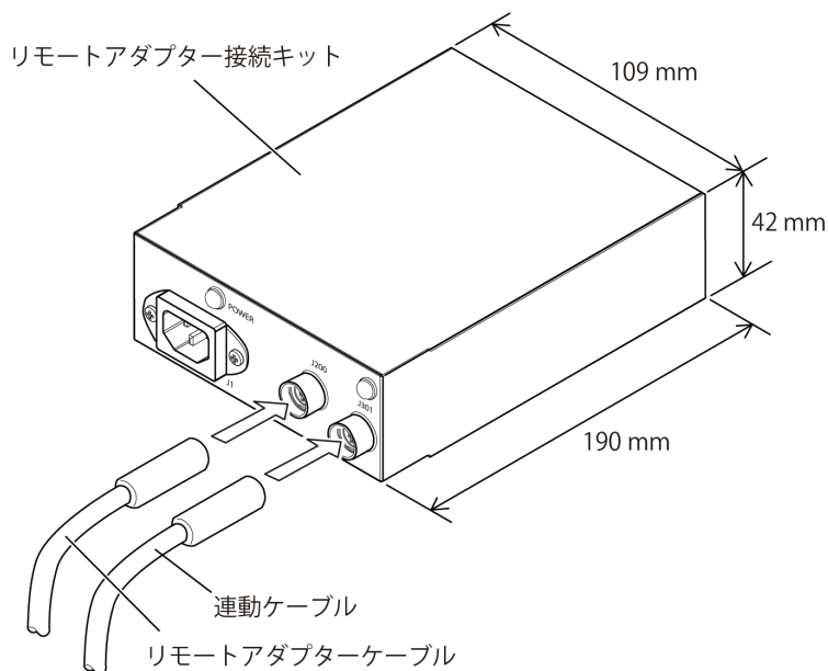
図 21 リモートアダプター接続キット (HT-F40SE-VR4C) 外観図
