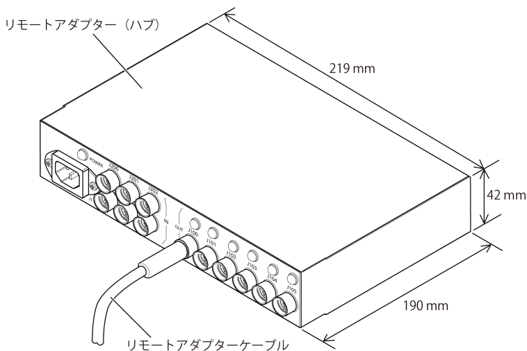
図 22 リモートアダプター (ハブ) (HT-F40SE-VR4H) 外観図
