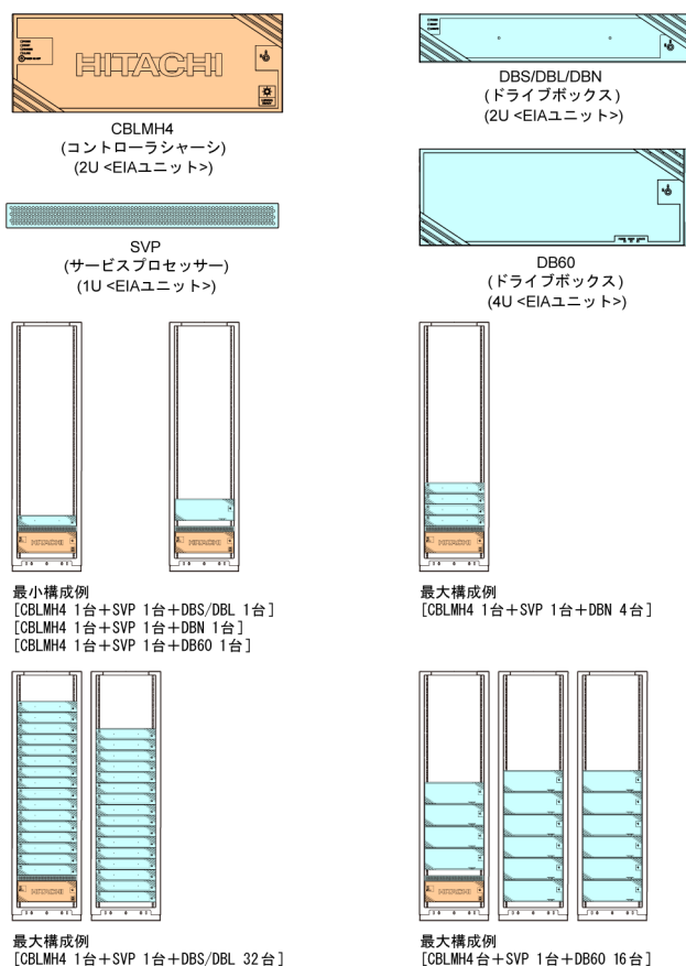
図9 ストレージシステム構成例 (CBLMH4 + SVP + DBS/DBL/DB60/DBN)
