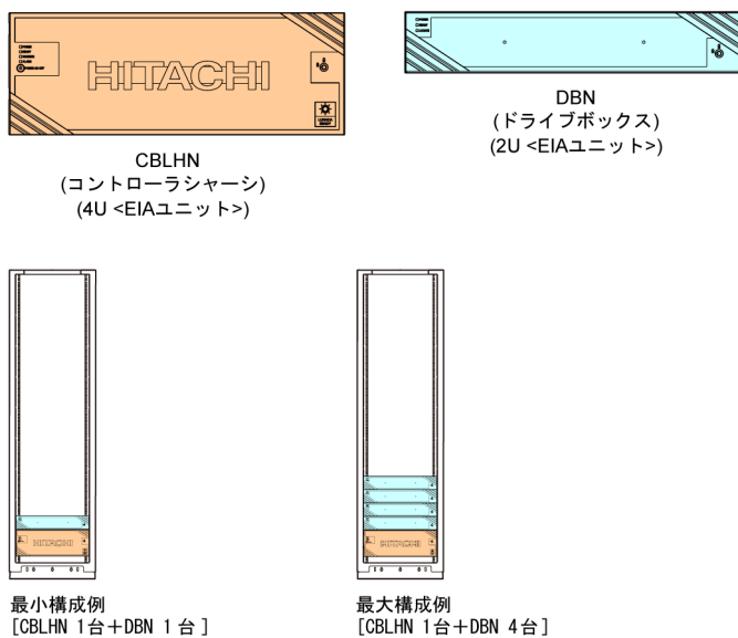
図 8 ストレージシステム構成例 (CBLHN + DBN)
