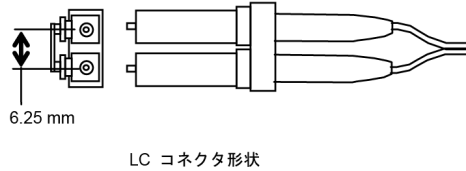
図 11 ケーブル側コネクタ形状
