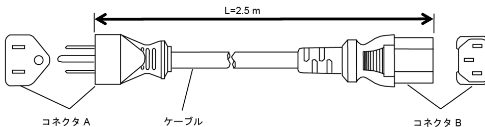
図 16 100V 電源ケーブル (J1K)
