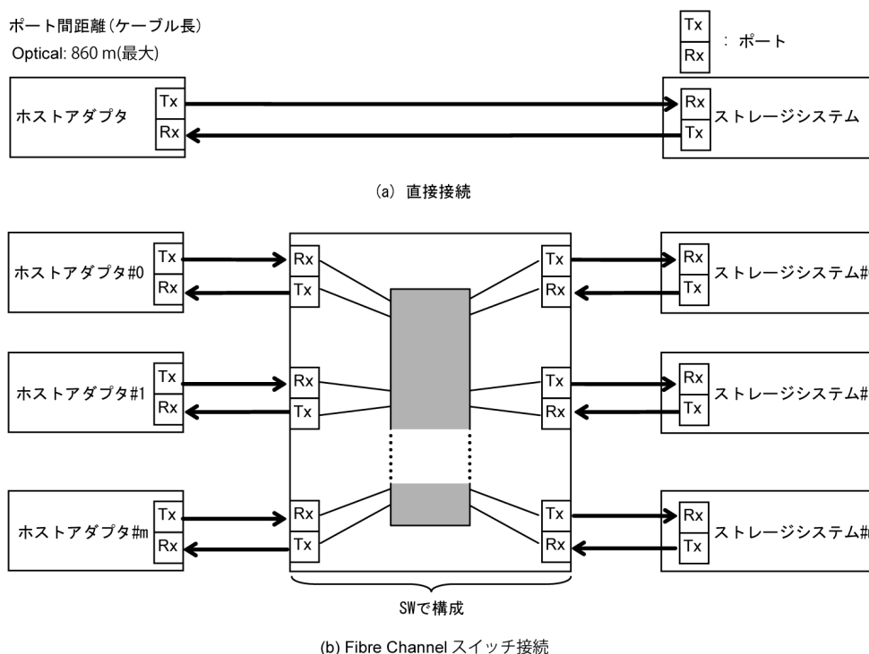
図 10 Fibre Channel 接続仕様
