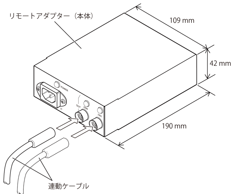
図 20 リモートアダプター (HT-F40SE-VR4B) 外観図
