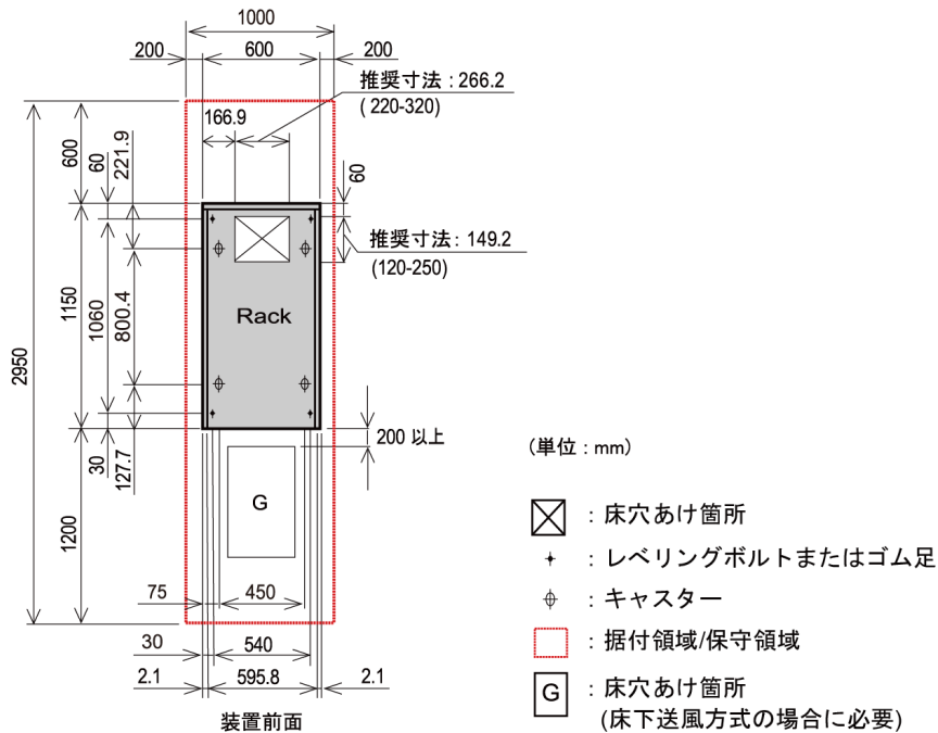
図 5 ラックの設置スペース・保守スペースと床穴あけ箇所
