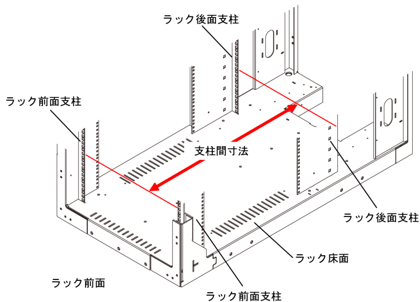
図 4 ラックの支柱間寸法
