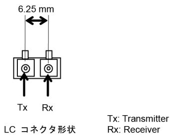
図 12 ストレージシステム側コネクタ形状
