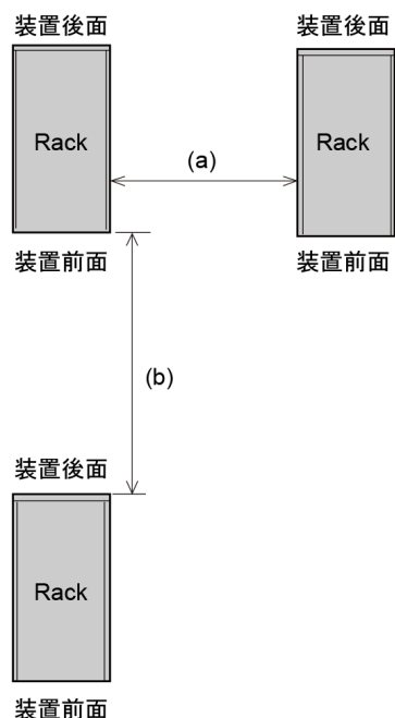
図 6 ラック間距離
