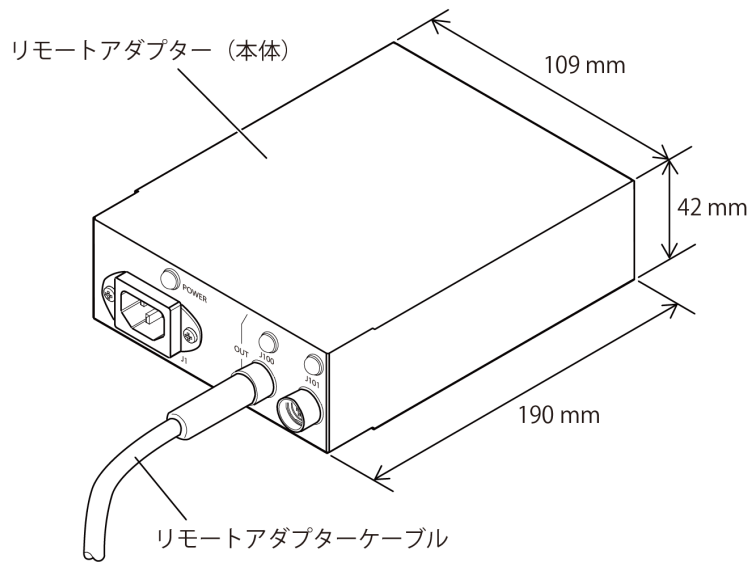
図 19 リモートアダプター (HT-F40SE-VR4A) 外観図
