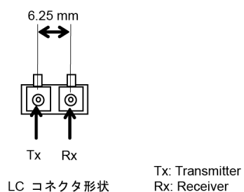
図 5-8 : ストレージシステム側コネクタ形状
