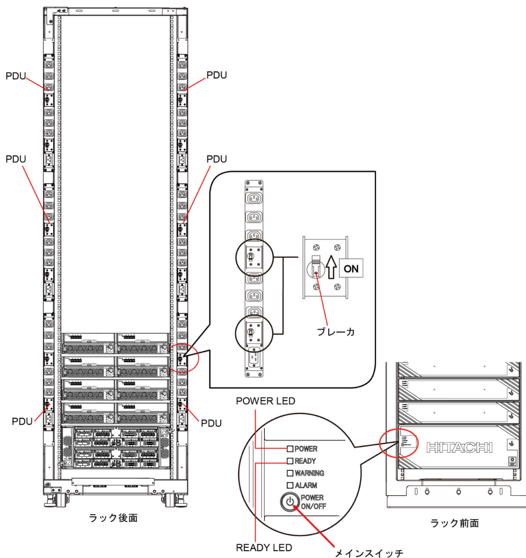
図 3-2 : 電源 ON (VSP E990)
