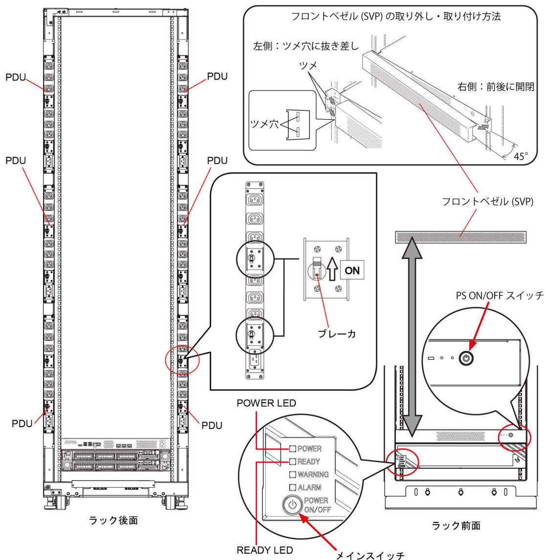
図 3-1 : 電源 ON (VSP E590, E790)
