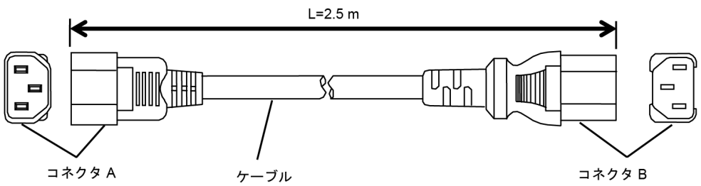
図 5-12 : 200V 電源ケーブル (J2H)
