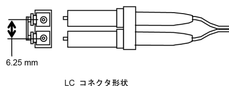
図 5-7 : ケーブル側コネクタ形状
