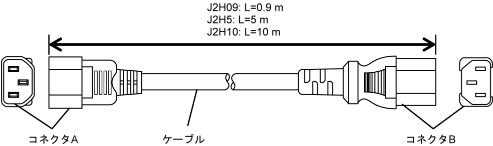
図 5-13 : 200V 電源ケーブル (J2H09、J2H5、J2H10)
