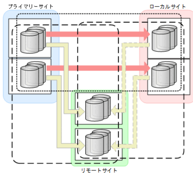
図 123 4x4x4 デルタリシンのコピーグループに関する構成例 (2x2x2)
