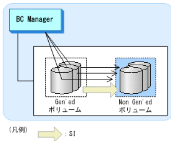
図 75 SI コピーペアの片方が Gen'ed ボリュームの場合の SI コピーグループの操作例
