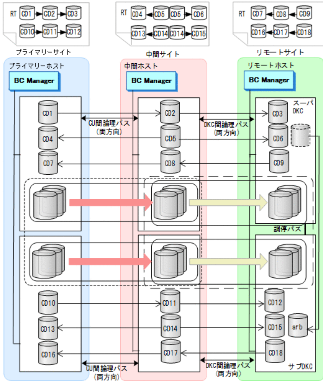
図 116 4x4x4 Cascade の構成例（2x2x2）
