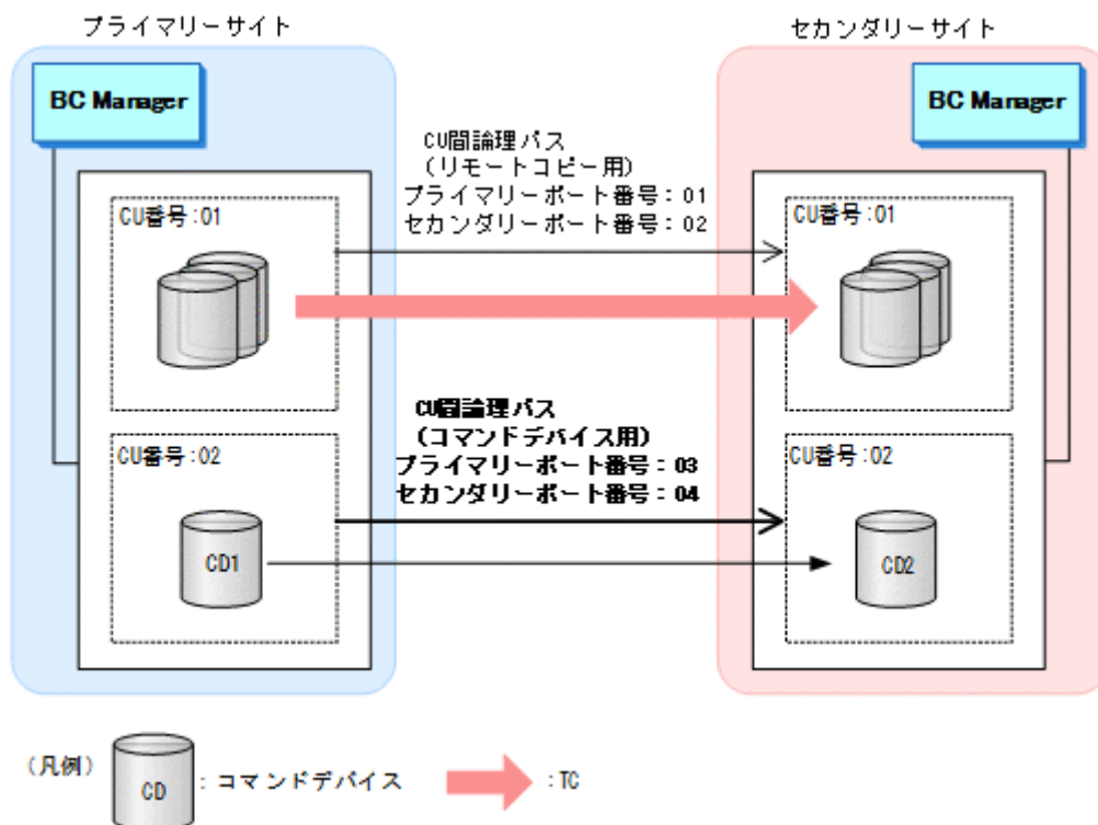
図 94 TC コピーグループの構成例
