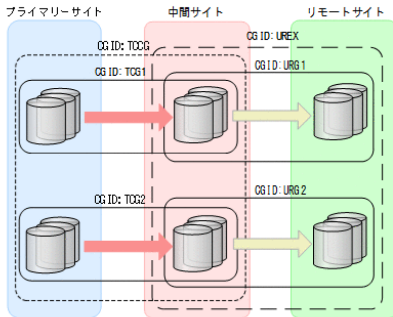
図 117 4x4x4 Cascade のコピーグループ
