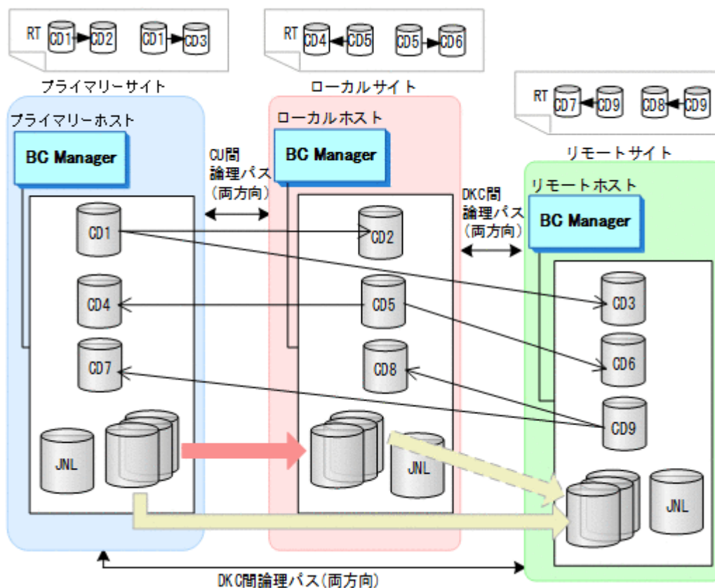
図 109 デルタリシンク構成例
