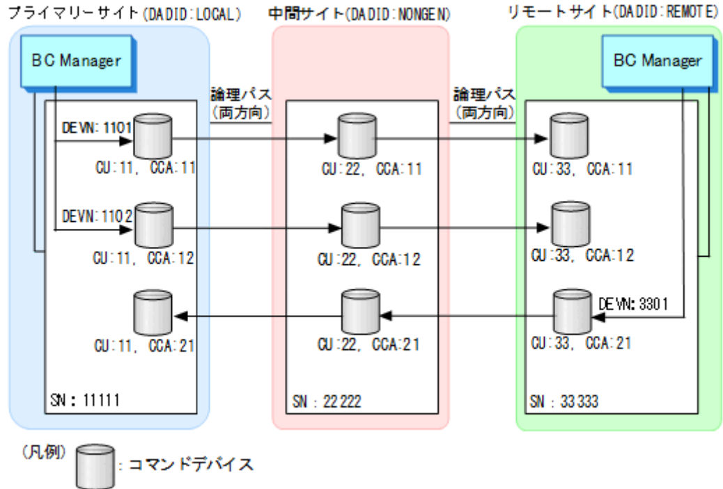
図 88 リモート DKC 制御機能を使用した構成例
