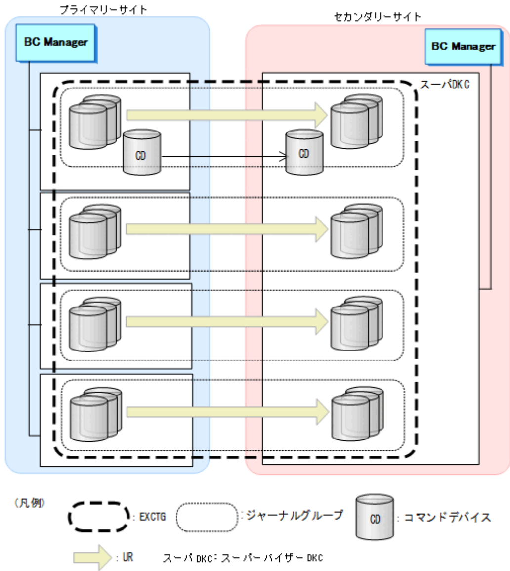
図 114 4x4 構成の構成例 (4 ストレージシステム : 1 ストレージシステム構成)
