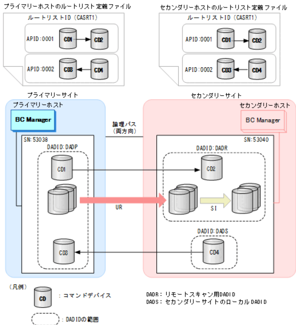
図 99 ケース B の構成例
