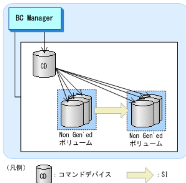
図 74 SI コピーペアの両方が Non Gen'ed ボリュームの場合の SI コピーグループの操作例
