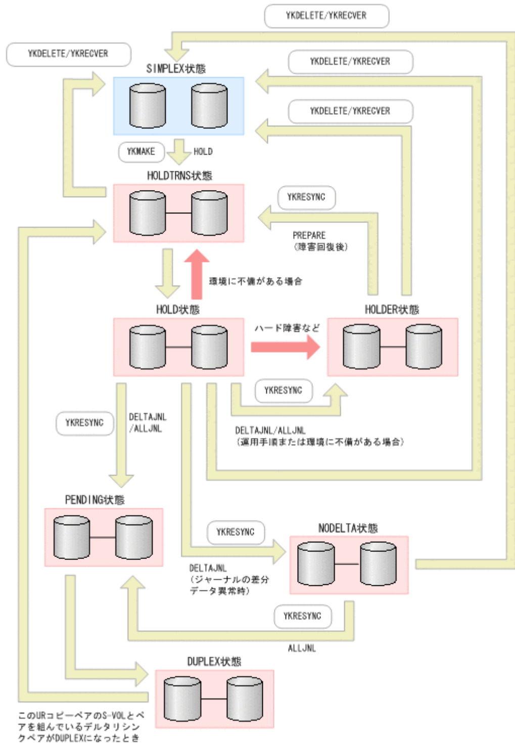
図 110 デルタリシンクペアのコピーペア状態の遷移
