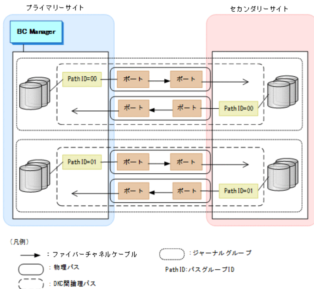
図 77 DKC 間論理パスの概要
