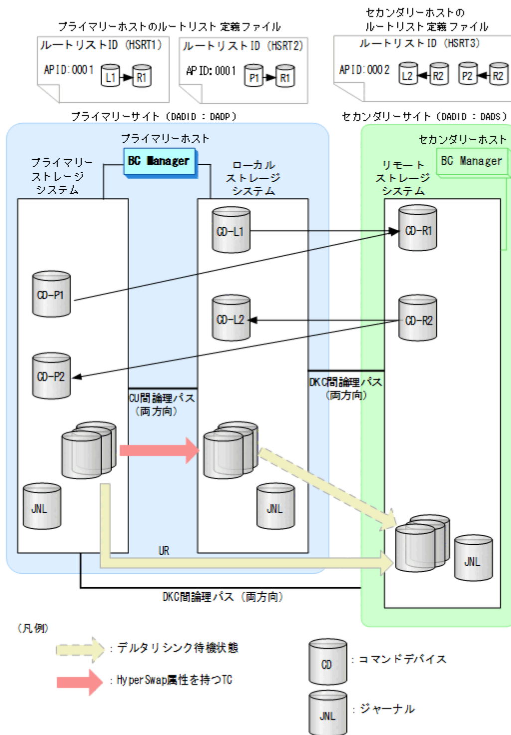
図 111 HyperSwap と UR を併用する 2DC 構成の構成例
