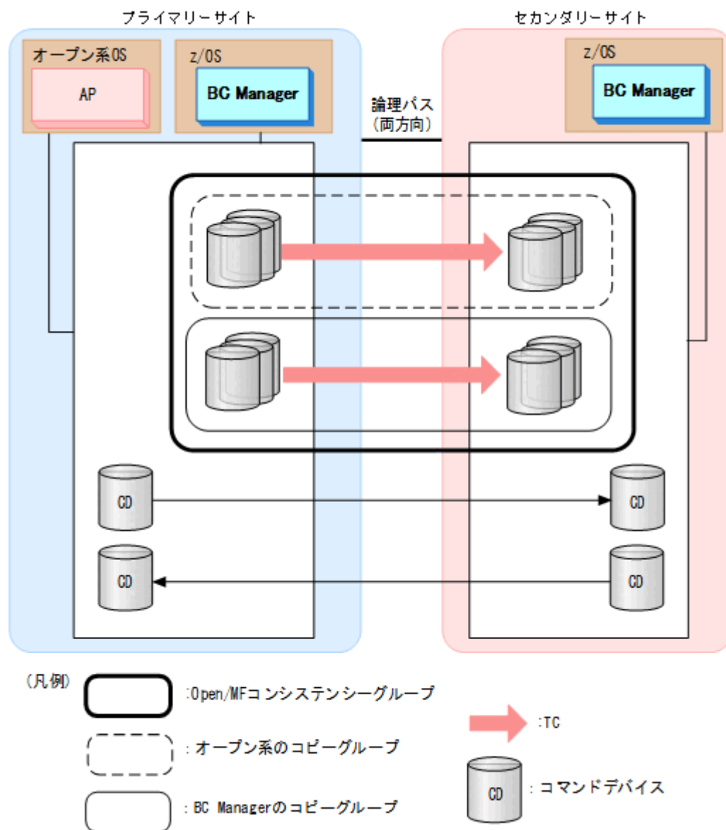
図 130 Open/MF コンシステンシー維持機能を使用した場合の構成例
