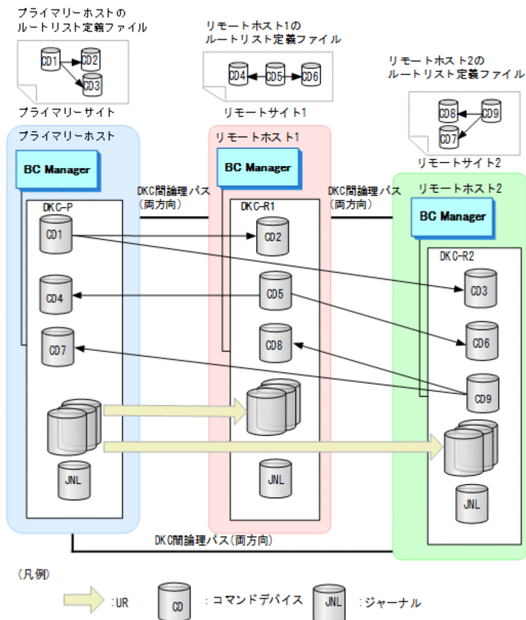
図 107 3DC Multi-Target (URxUR)構成例
