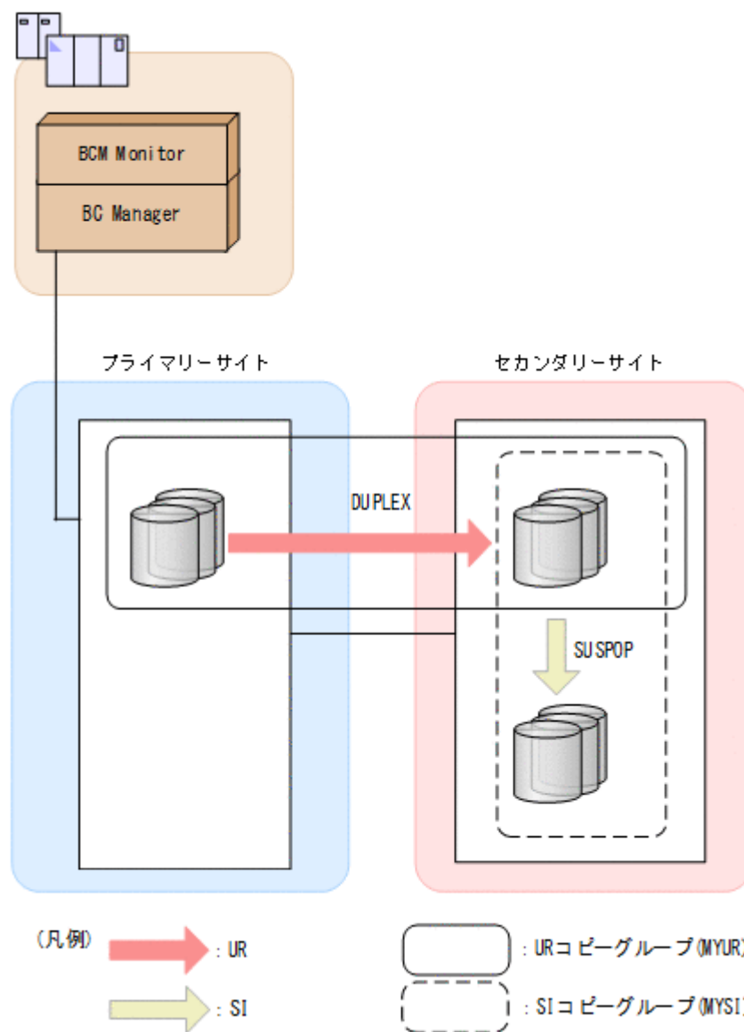
図 163 BCM Monitor を使用したバックアップ運用の構成例
