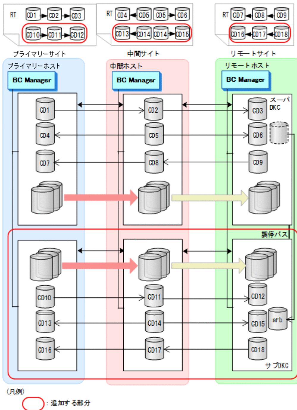
図 120 3DC Cascade (TCxUR)構成を 4x4 Cascade 構成に拡張する構成例
