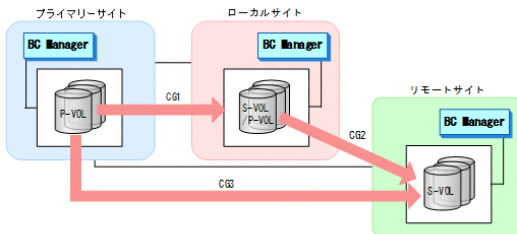
図 83 3DC Multi-Target 構成の例
