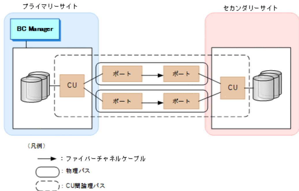
図 76 正方向の CU 間論理パスの概要
