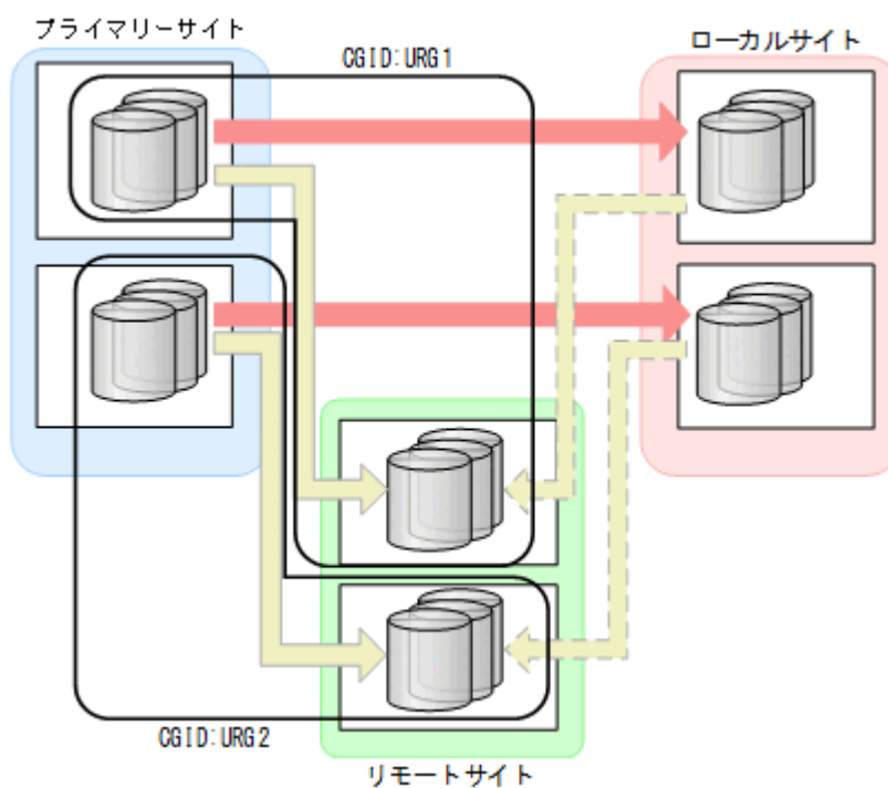
図 126 4x4x4 デルタリシンのコピーグループ (UREX1 の障害時操作)
