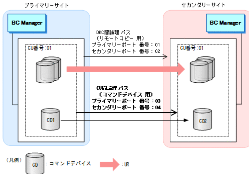
図 95 UR コピーグループの構成例
