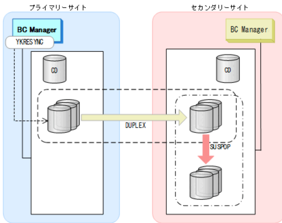
図 152 コピーグループの構成例
