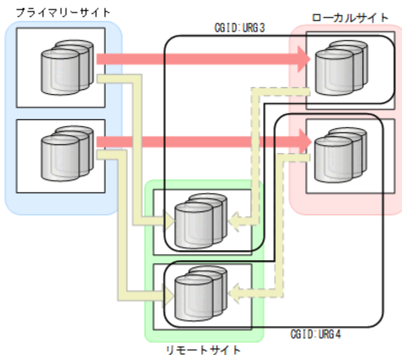
図 127 4x4x4 デルタリシンのコピーグループ (UREX2 の障害時操作)
