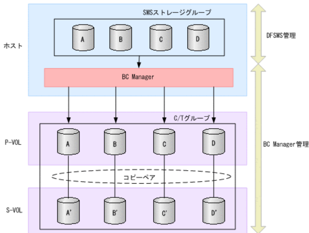
図 62 SMS ストレージグループと複製製品の関係
