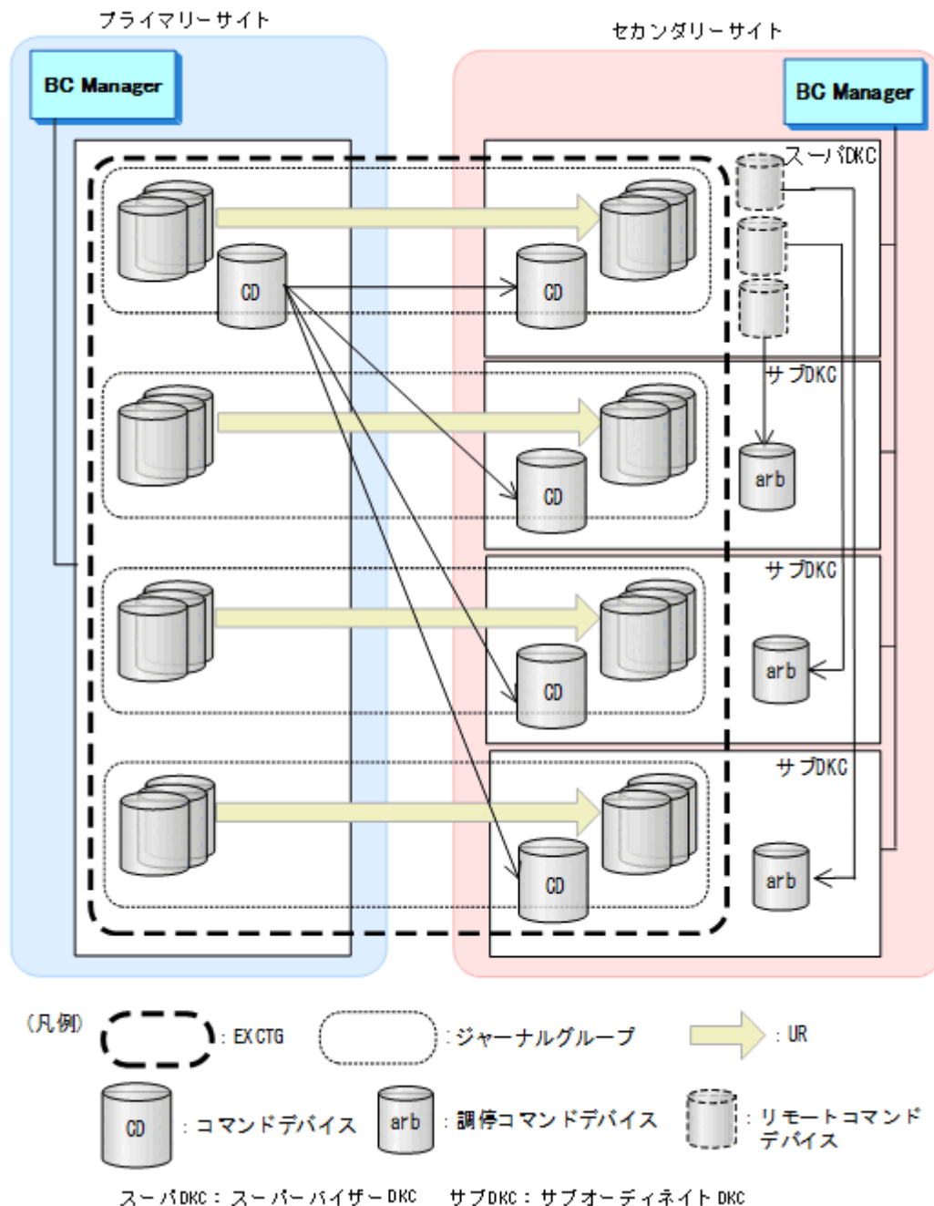
図 115 4x4 構成の構成例 (1 ストレージシステム : 4 ストレージシステム構成)
