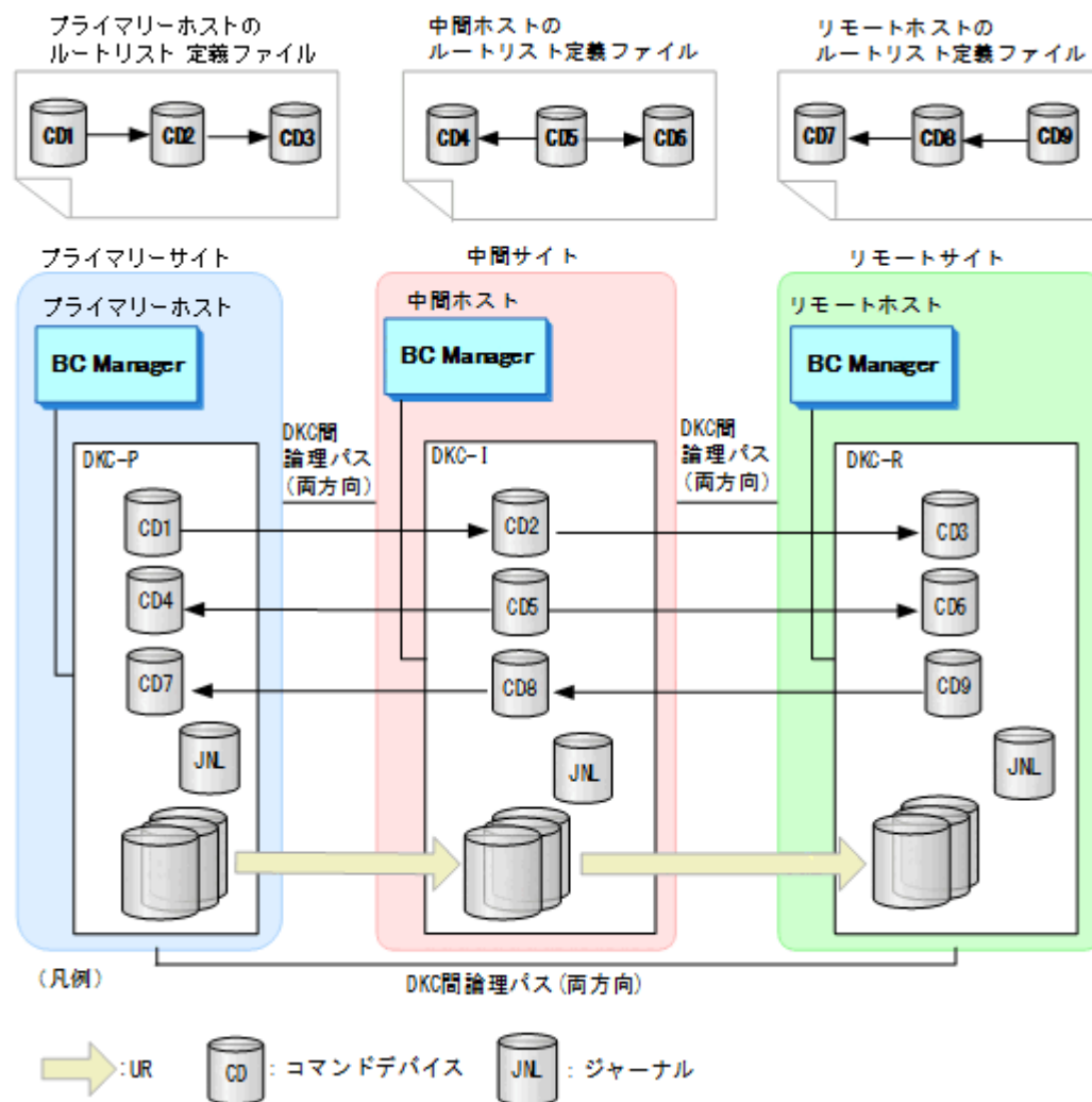
図 105 3DC Cascade (URxUR)構成例
