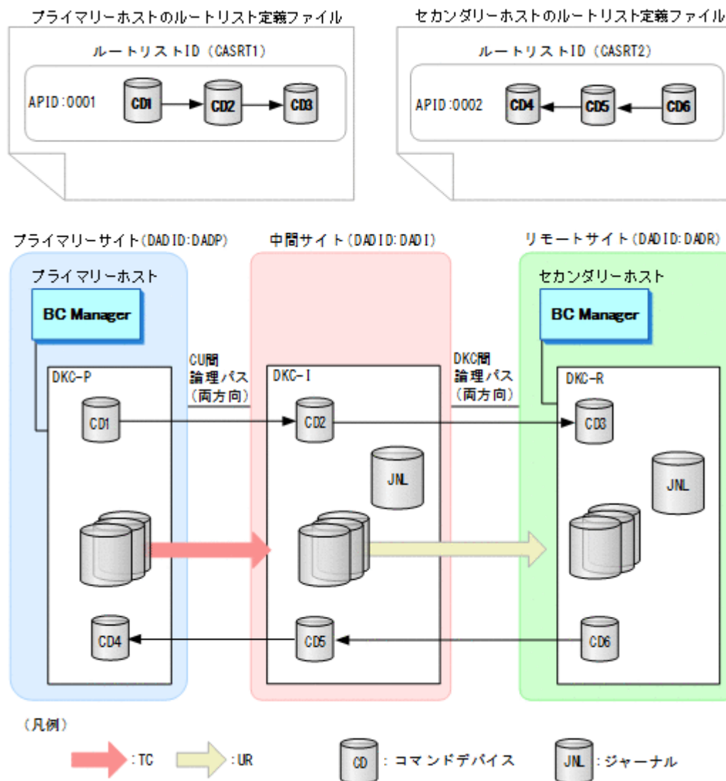
図 104 3DC Cascade (TCxUR)構成例
