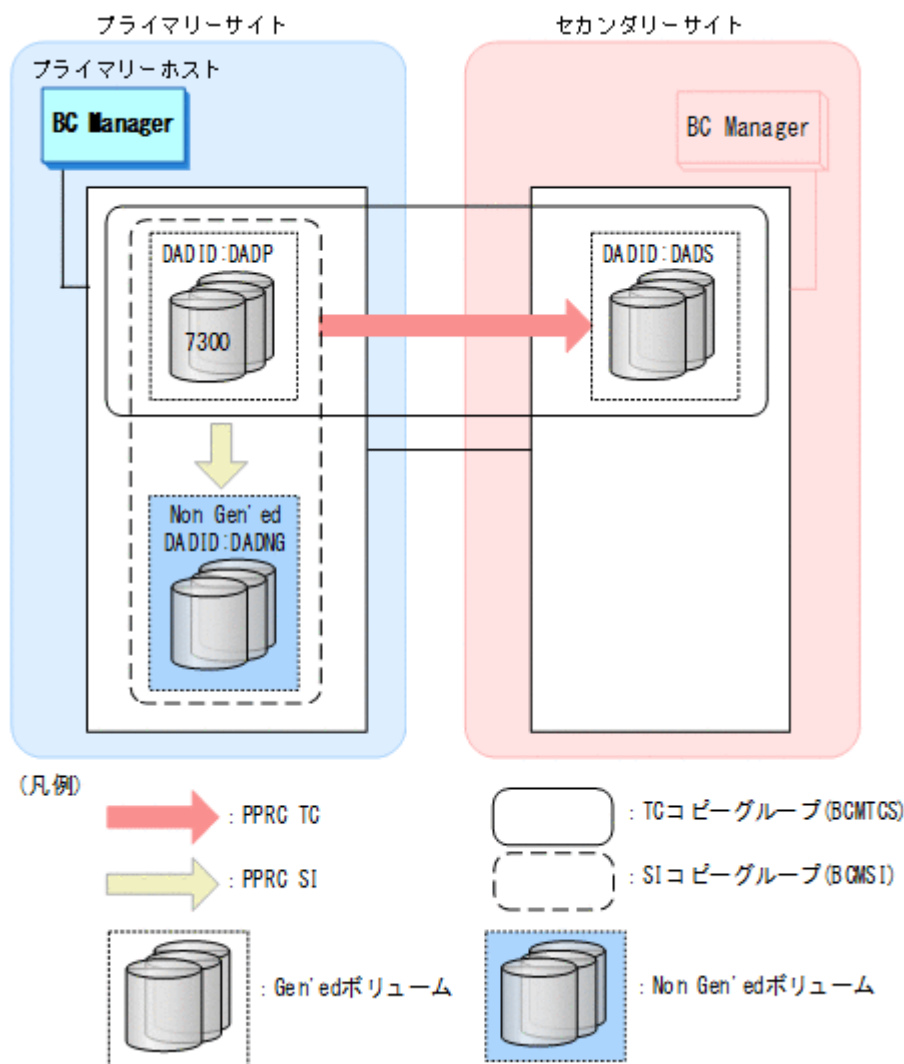
図 158 PPRC TC/SI コピーペアの構成例
