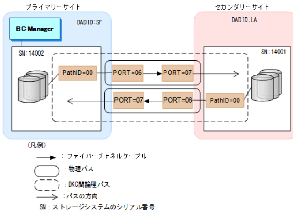
図 141 DKC 間論理パスの定義例
