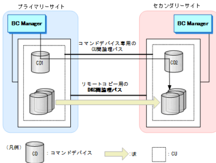
図 52 UR の場合のコマンドデバイス専用の CU 間論理パスのイメージ
