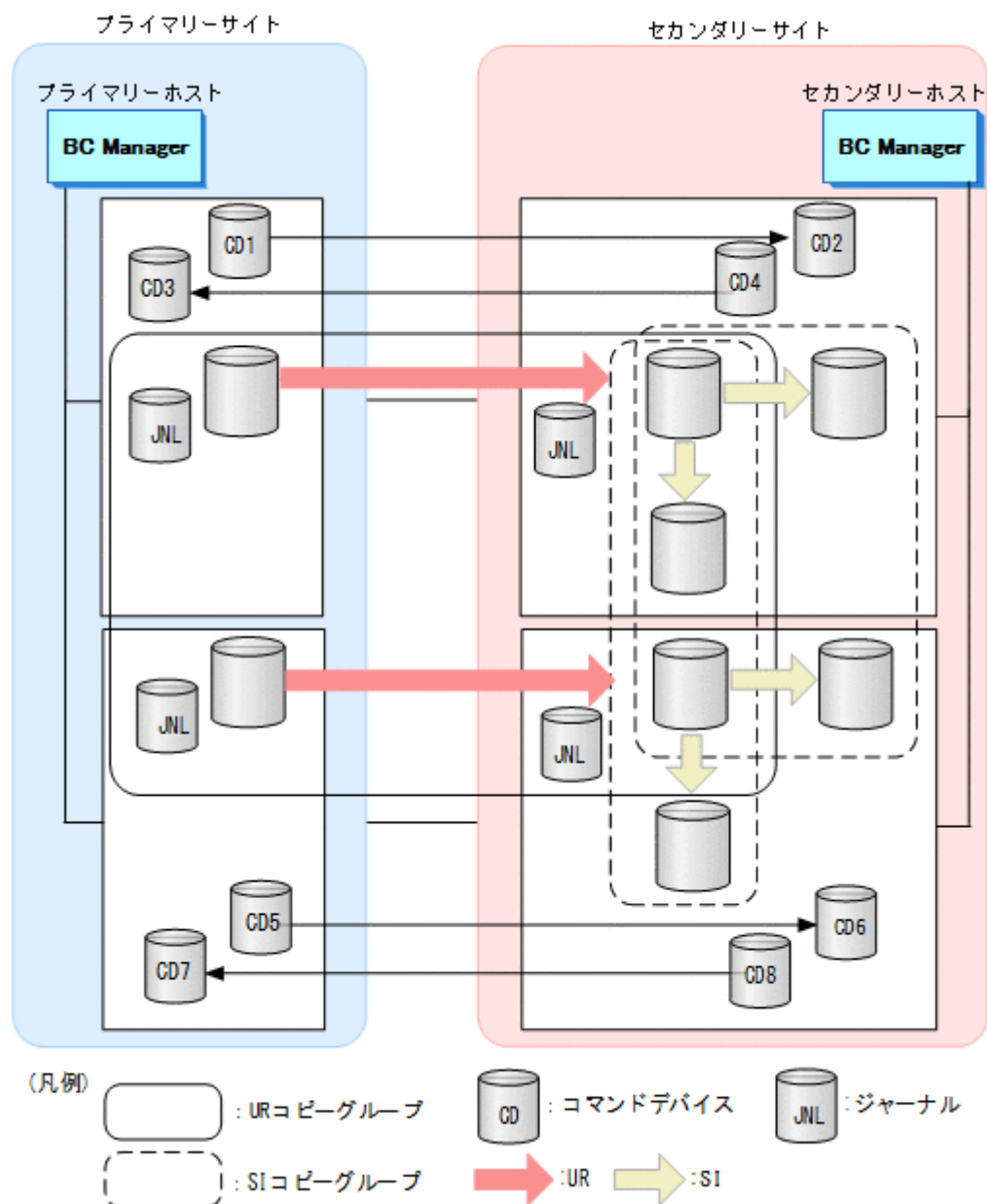
図 128 UR ATTIME サスペンド機能を使用するための構成例
