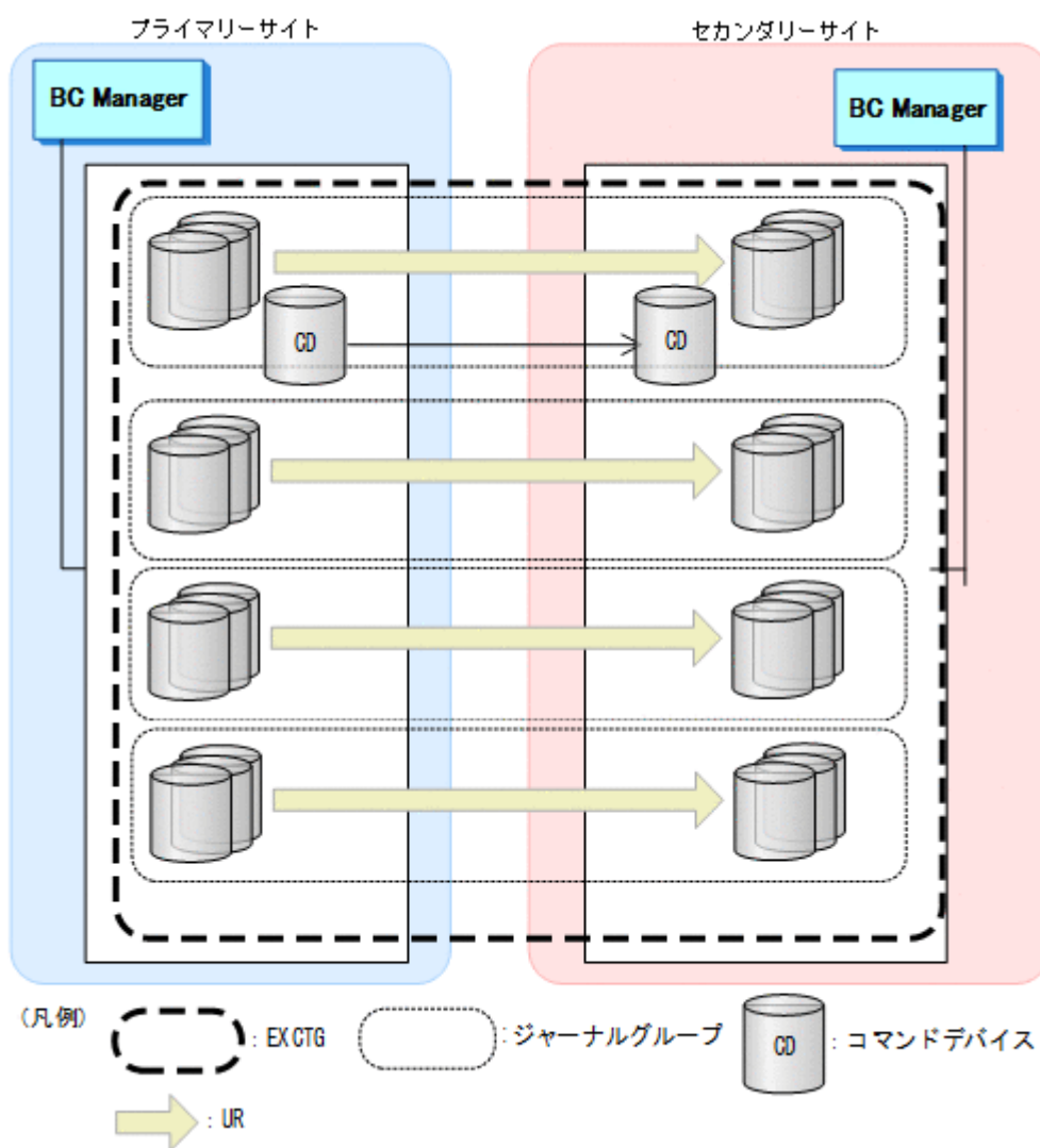
図 112 4x4 構成の構成例 (1 ストレージシステム : 1 ストレージシステム構成)
