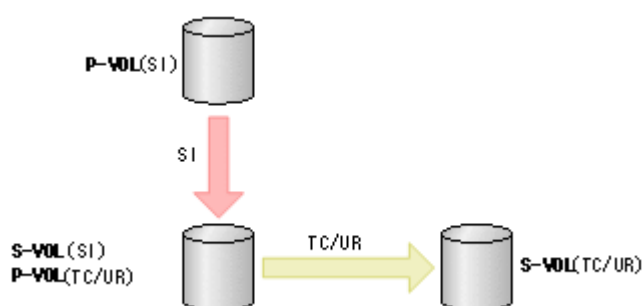
図 40 SI の S-VOL と TC または UR の P-VOL が同じ構成
