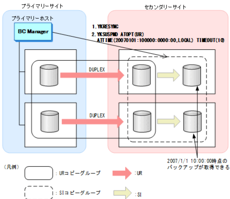
図 65 UR ATTIME サスペンド機能を使用した UR のバックアップ構成例
