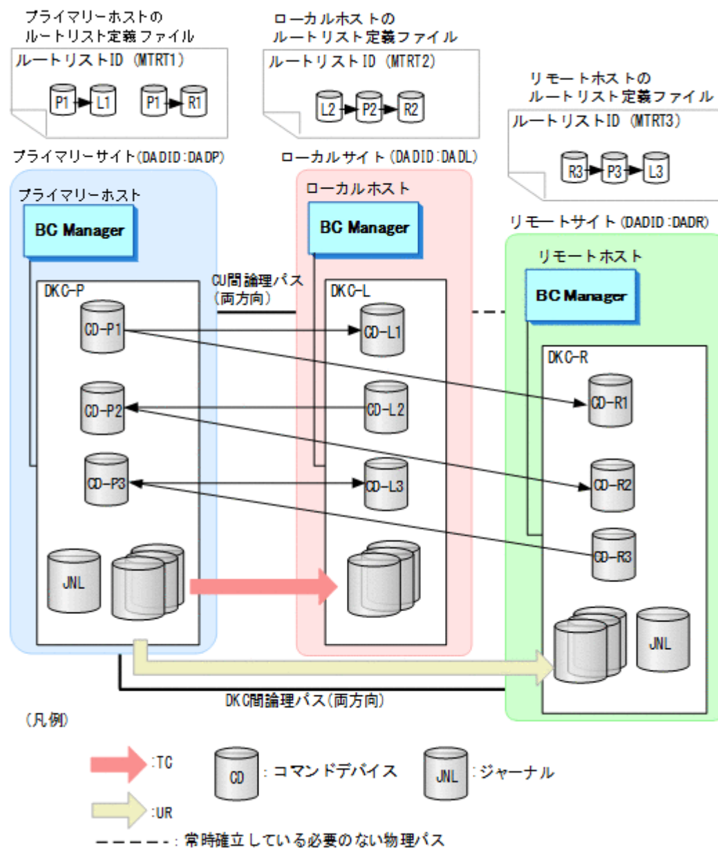
図 106 3DC Multi-Target (TCxUR)構成例
