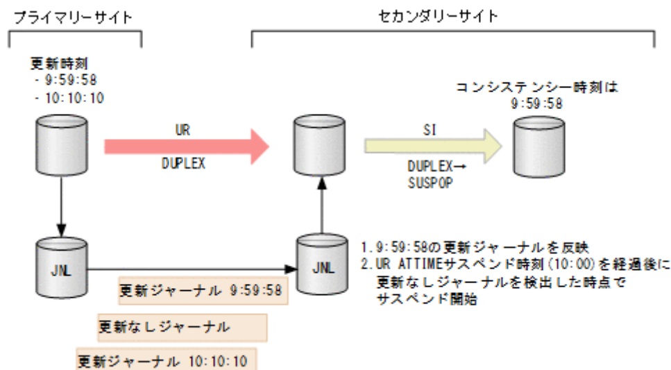
図 68 指定した UR ATTIME サスペンド時刻よりあとの更新なしジャーナル検出によるサスペンド実行
