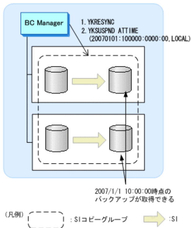
図 64 NORMAL ATTIME サスペンド機能を使用した SI のバックアップ構成例
