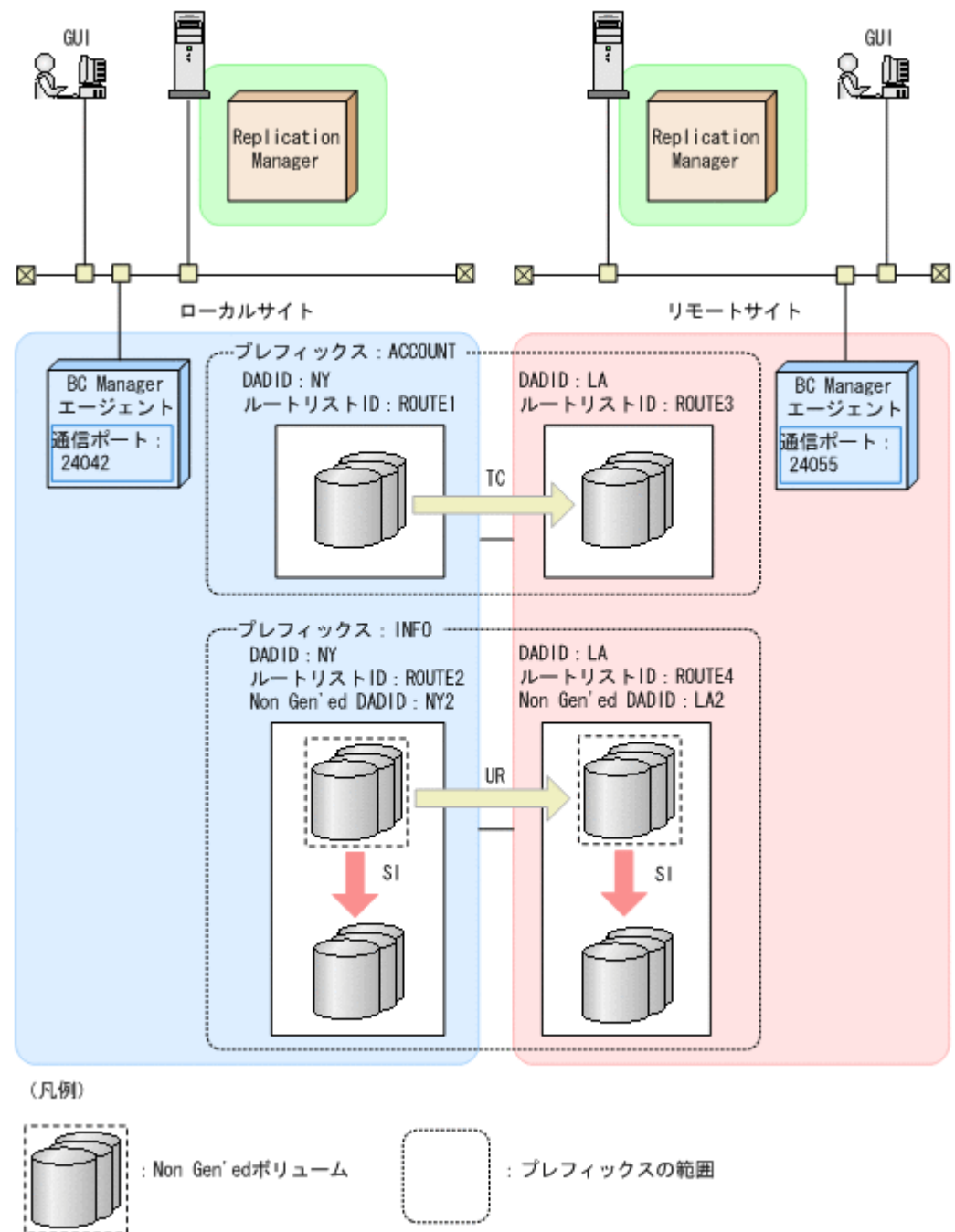
図 3-9 BC Manager エージェントがローカルサイトとリモートサイトにある場合の構成例
