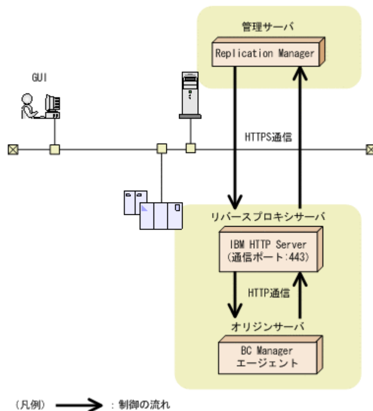
図 3-6 Replication Manager と IBM HTTP Server が HTTPS 通信する場合の構成例
