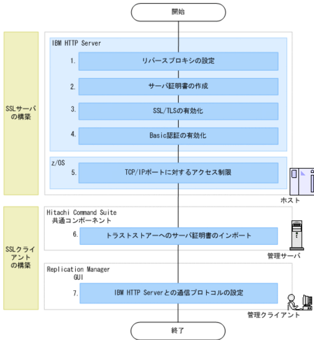
図 3-7 HTTPS 通信するために必要な設定の流れ
