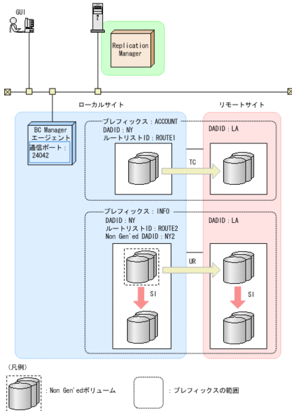
図 3-8 BC Manager エージェントがローカルサイトだけにある場合の構成例
