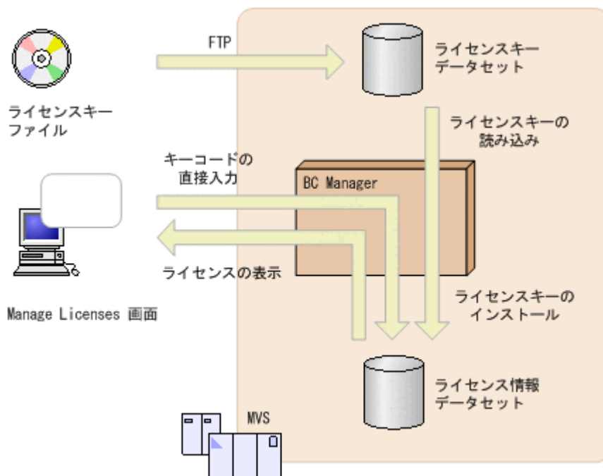
図 2-2 ライセンス登録の概要
