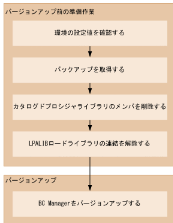
図 2-3 BC Manager のバージョンアップの流れ
