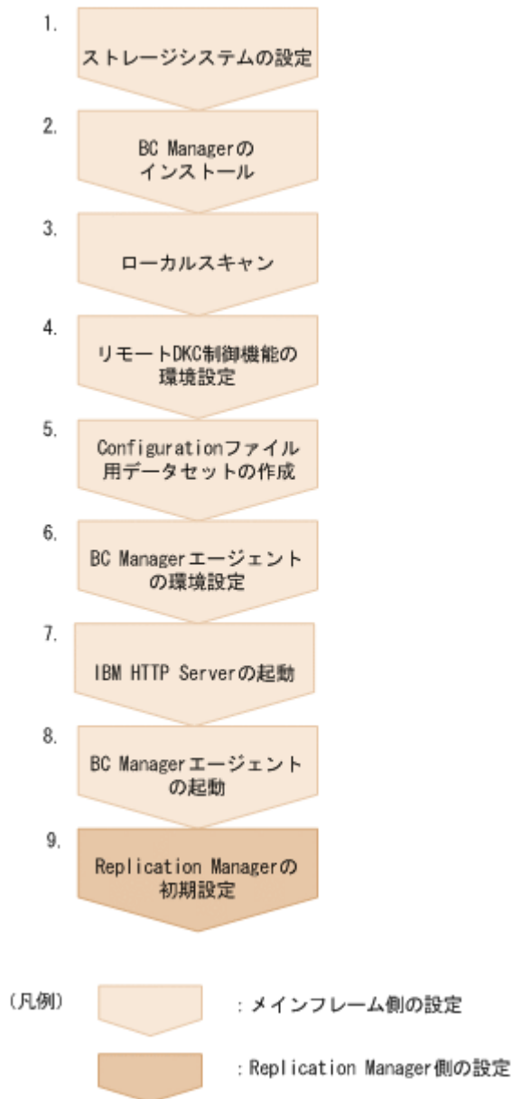
図 3-2 BC Manager のインストール前で、リモート DKC 制御機能を使用する場合の環境設定
