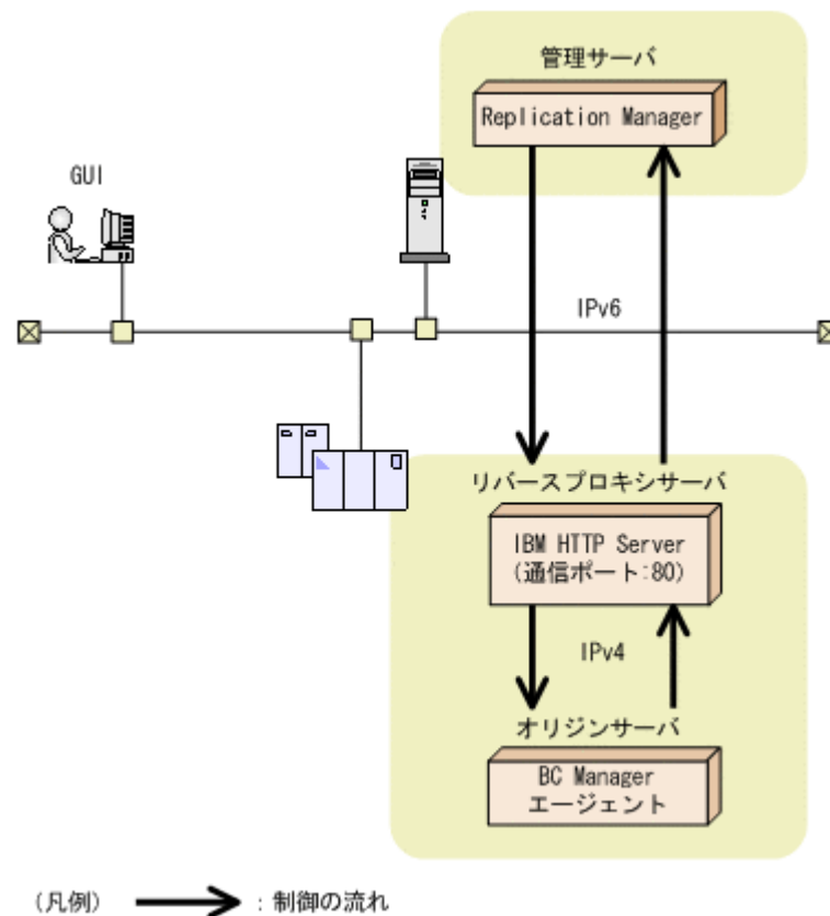
図 3-5 Replication Manager と BC Manager エージェントが IPv6 接続する場合の構成例
