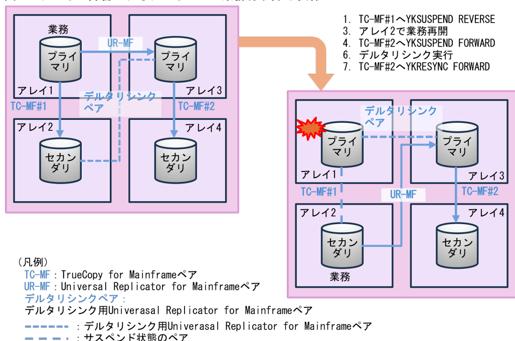
図 45 アレイ 1 障害によるアレイ 2 への業務切り替え手順
