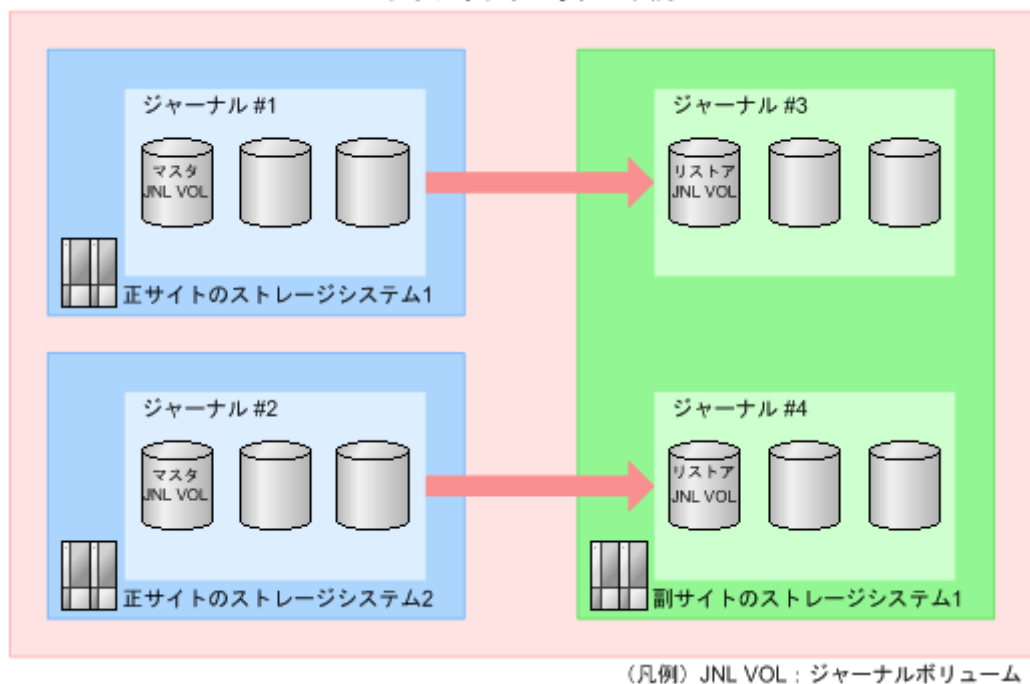
図 12 複数のジャーナルを伴う RAID Manager のコンシステンシーグループの構成例 (2) コンシステンシーグループ#0
