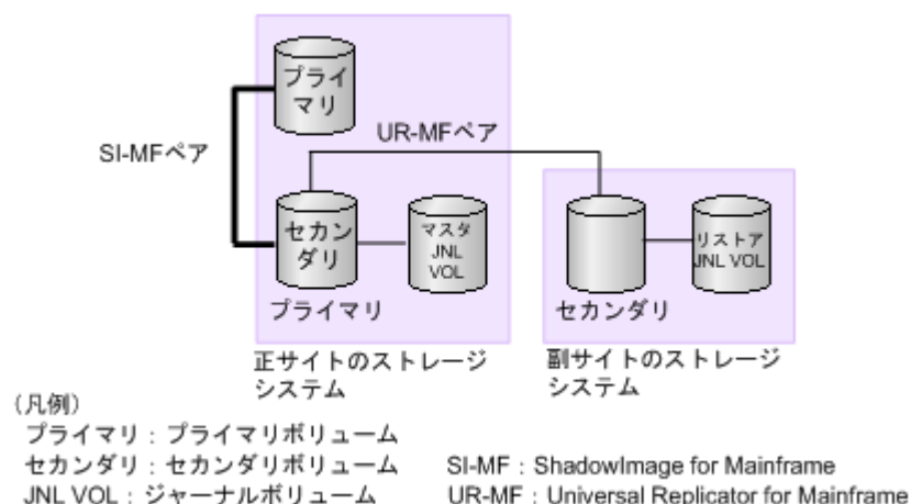
図 62 Universal Replicator for Mainframe ペアのプライマリボリュームと ShadowImage for Mainframe ペアのセカンダリボリュームを共有する構成
