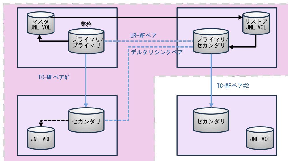
図 58 4DC 構成内のデルタリシンク処理の実行条件が適用される構成
