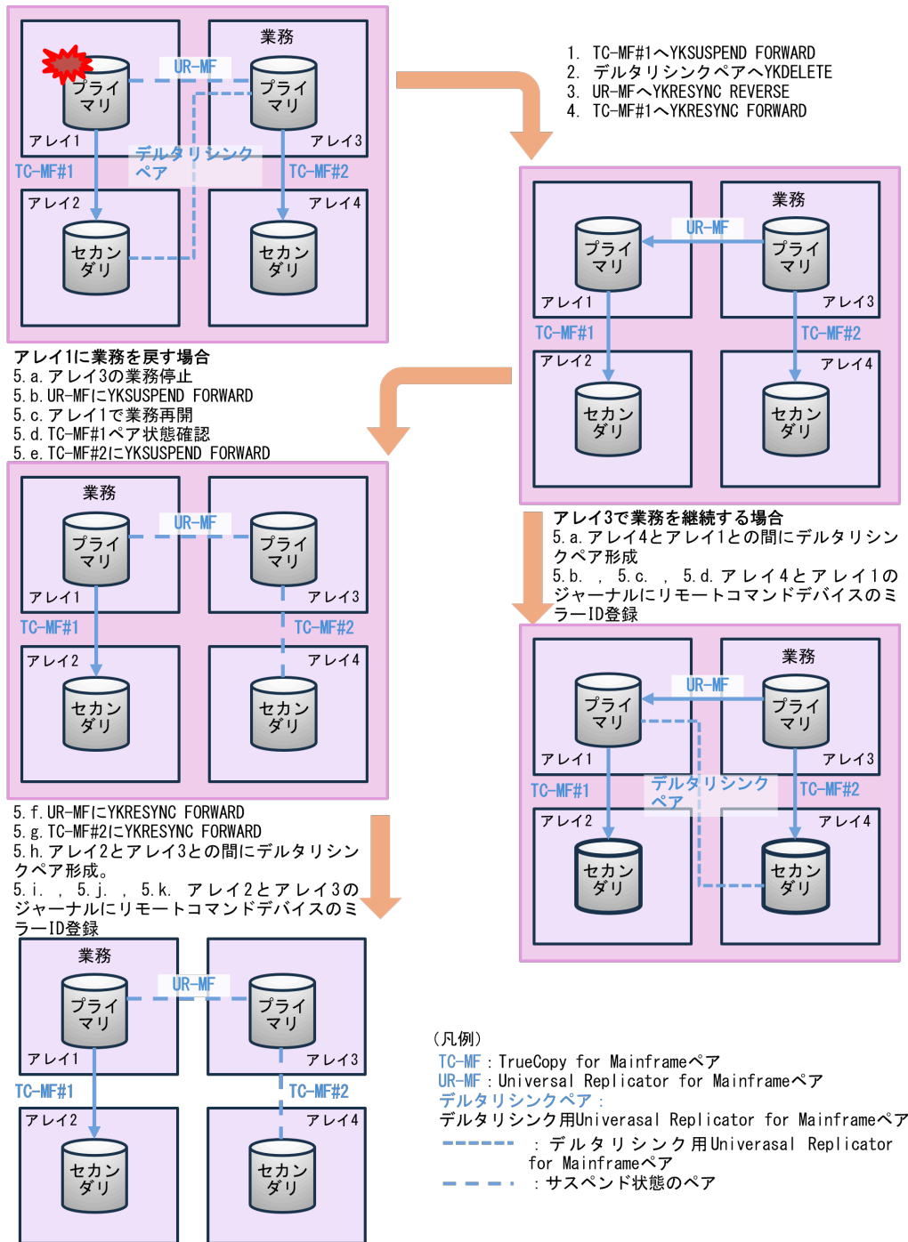
図 48 アレイ 3 に移動した業務をアレイ 1 に戻すまたはアレイ 3 で業務を継続する手順
