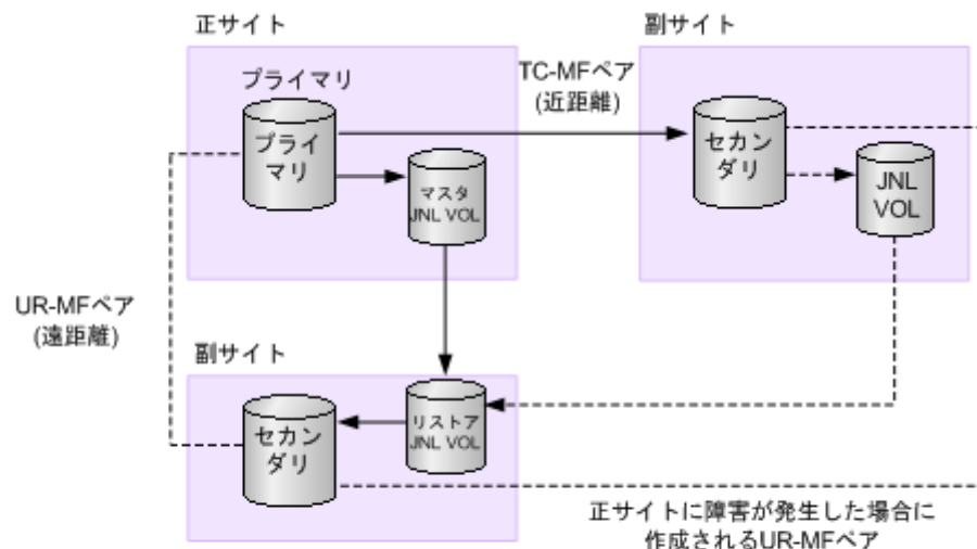
図 52 3DC マルチターゲット
