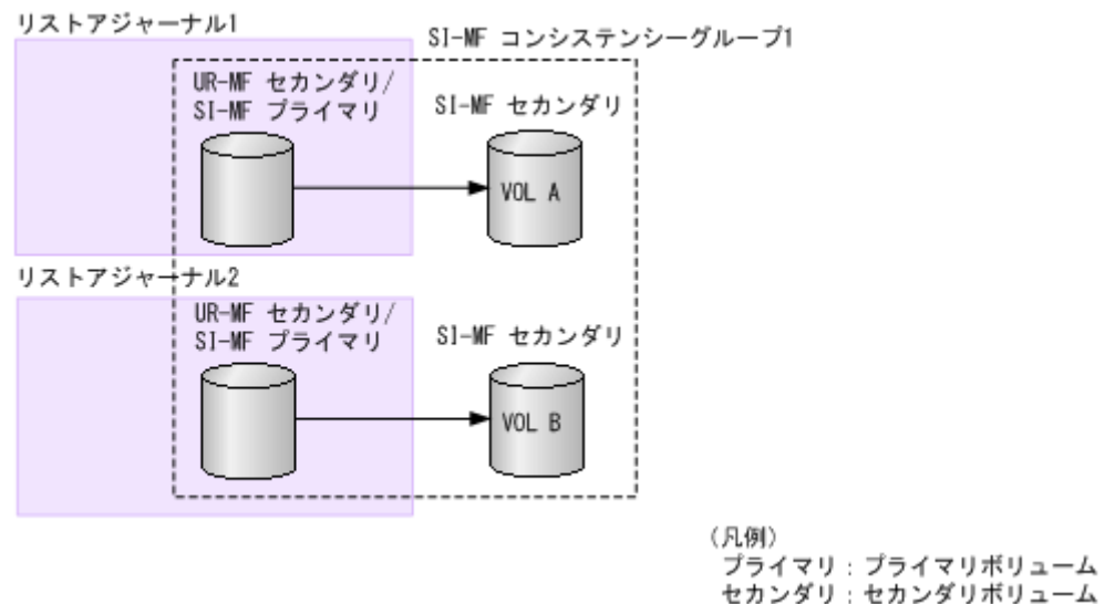
図 64 複数のジャーナルが 1 つの ShadowImage for Mainframe のコンシステンシーグループに登録されている構成
