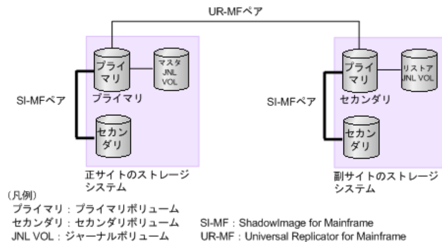
図 61 Universal Replicator for Mainframe ペアのプライマリボリュームと ShadowImage for Mainframe ペアのプライマリボリュームを共有し、さらに Universal Replicator for Mainframe ペアのセカンダリボリュームと ShadowImage for Mainframe ペアのプライマリボリュームを共有する構成
