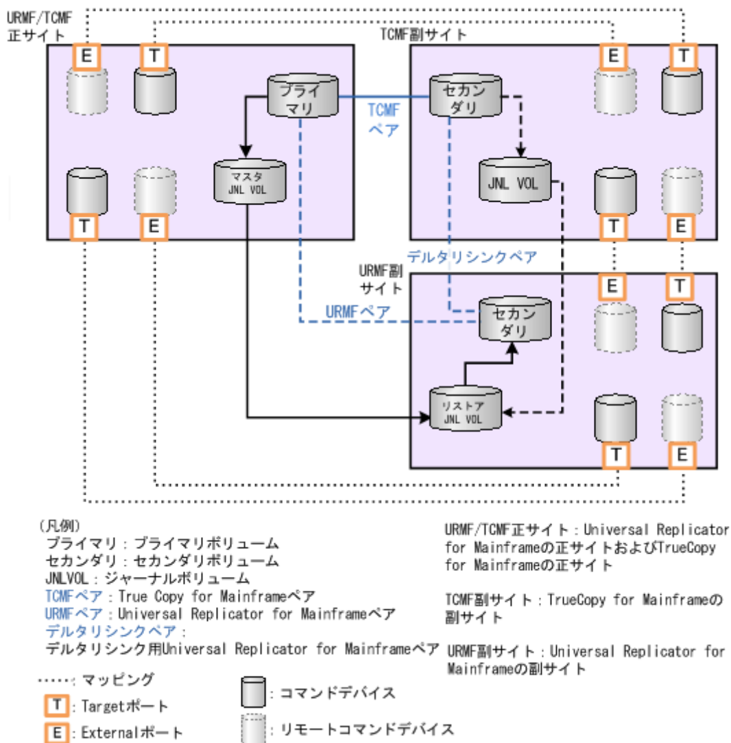
図 53 デルタリシンクに対応した 3DC マルチターゲット構成
