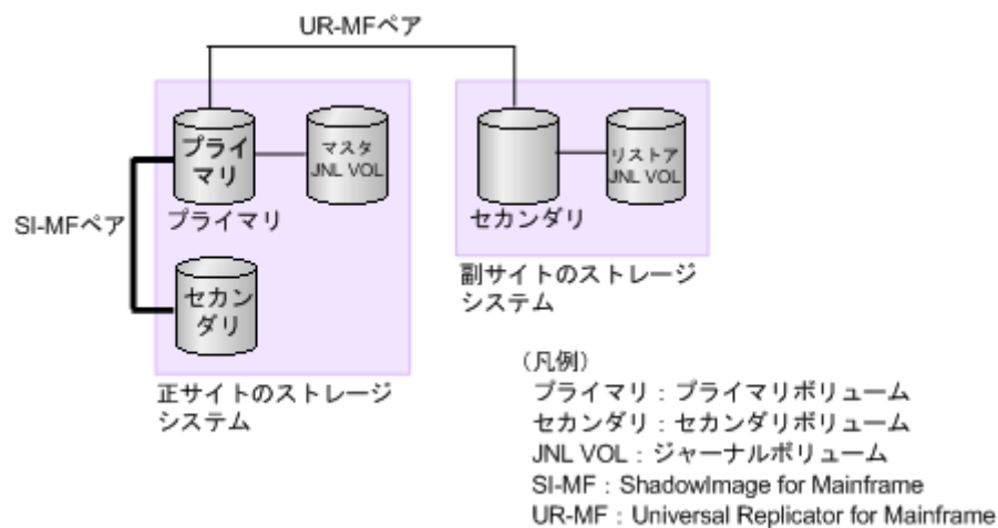
図 59 Universal Replicator for Mainframe ペアと ShadowImage for Mainframe ペアの プライマリボリュームを共有する構成
