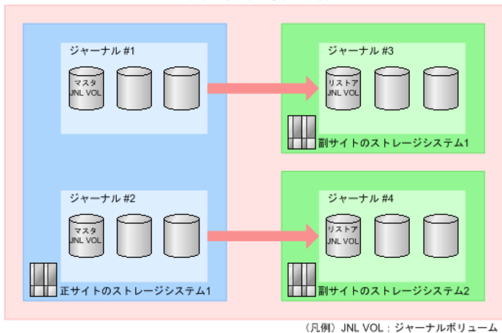
図 11 複数のジャーナルを伴う RAID Manager のコンシステンシーグループの構成例 (1) コンシステンシーグループ#0
