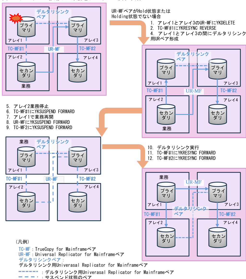
図 46 アレイ 2 に移動した業務をアレイ 1 に戻す手順
