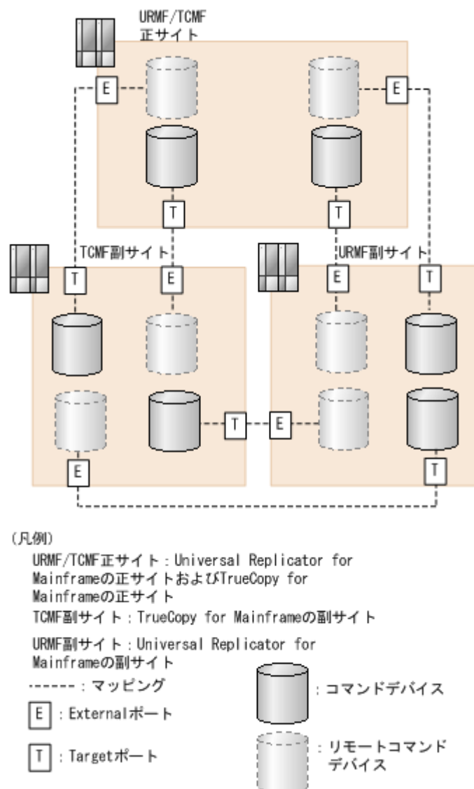
図 55 デルタリシンク用リモートコマンドデバイス構成
