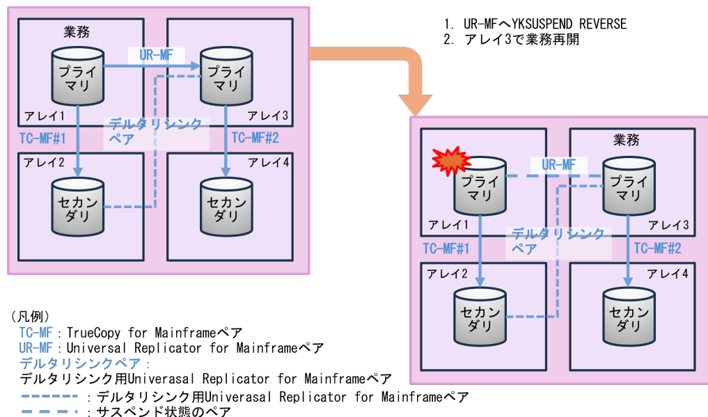
図 47 アレイ 1 障害によるアレイ 3 への業務切り替え
