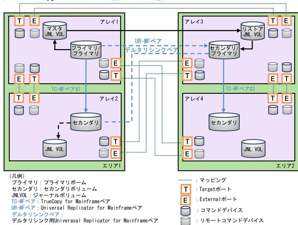
図 56 TrueCopy for Mainframe と併用した 4DC 構成
