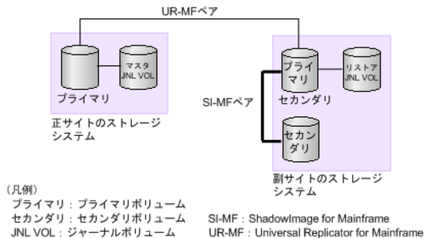
図 60 Universal Replicator for Mainframe ペアの セカンダリボリュームと ShadowImage for Mainframe ペアのプライマリボリュームを共有する構成
