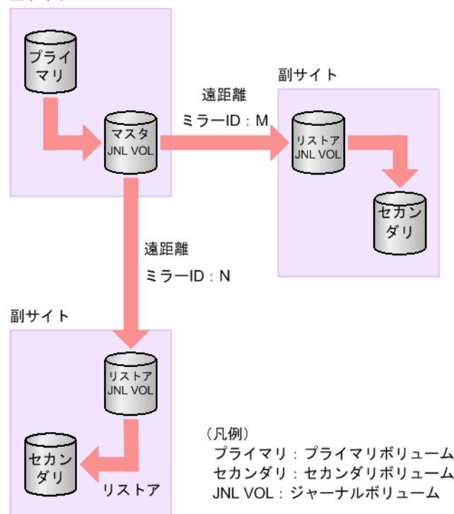
図 4 3つの Universal Replicator for Mainframe サイトによる 3DC マルチターゲット構成
