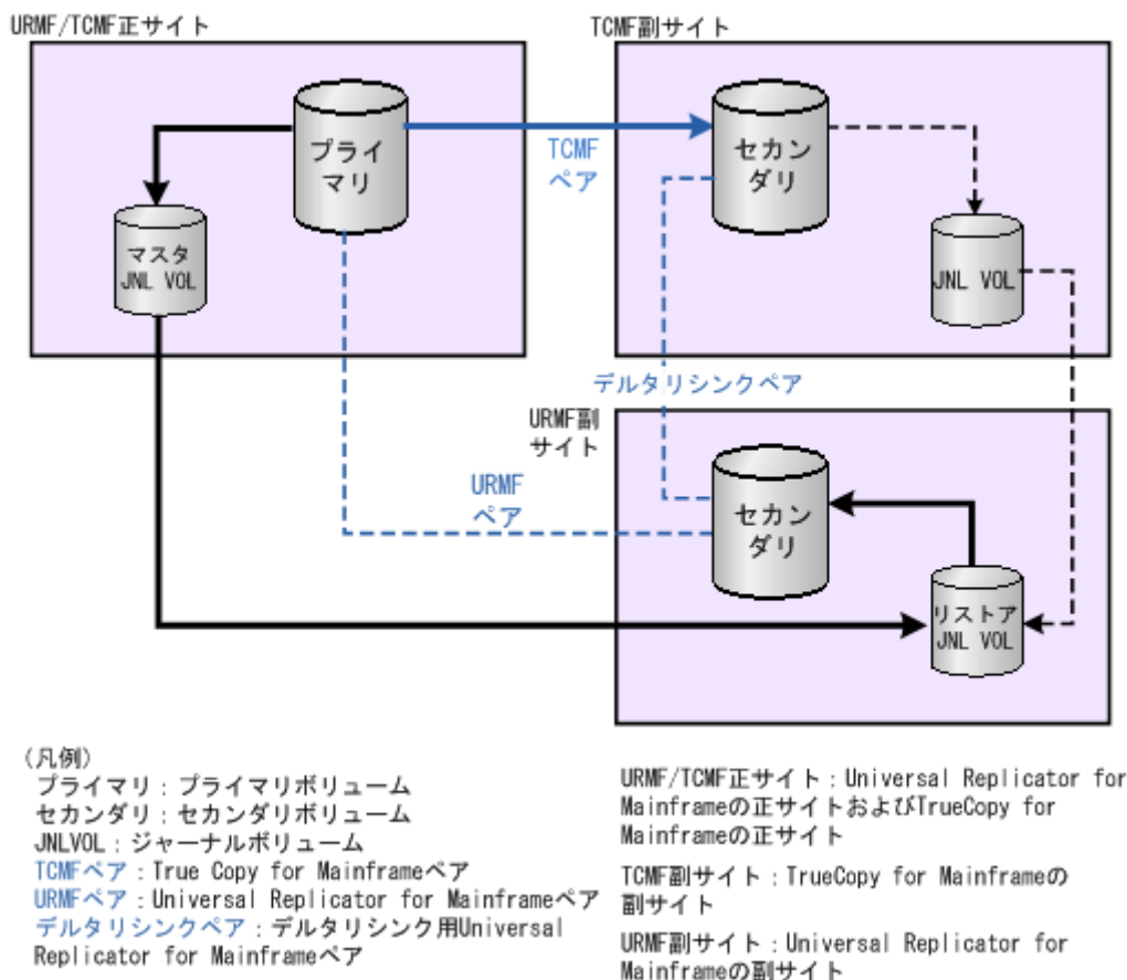
図 39 デルタリシンク用 3DC マルチターゲット構成
