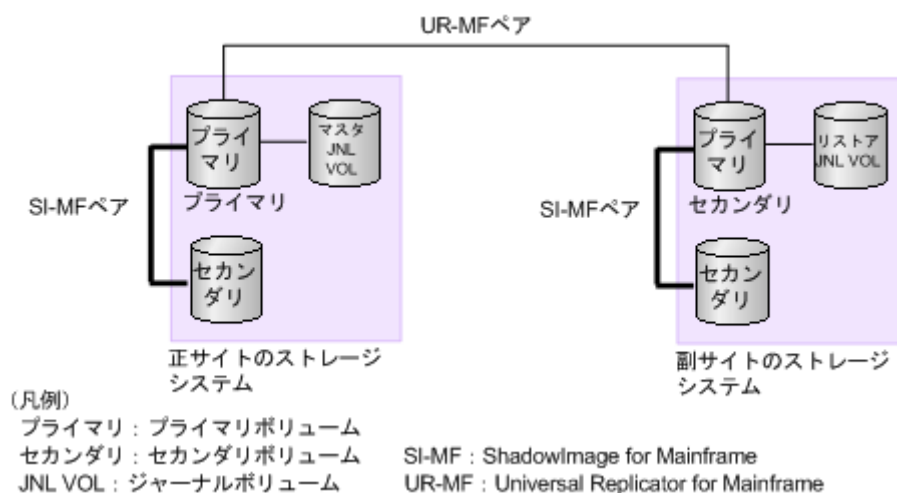
図 43 Universal Replicator for Mainframe ペアのプライマリボリュームと ShadowImage for Mainframe ペアのプライマリボリュームを共有し、さらに Universal Replicator for Mainframe ペアのセカンダリボリュームと ShadowImage for Mainframe ペアのプライマリボリュームを共有する構成
