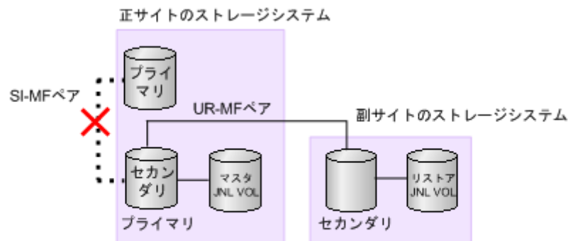
図 25 ShadowImage for Mainframe プライマリボリュームの復旧手順 (1)
