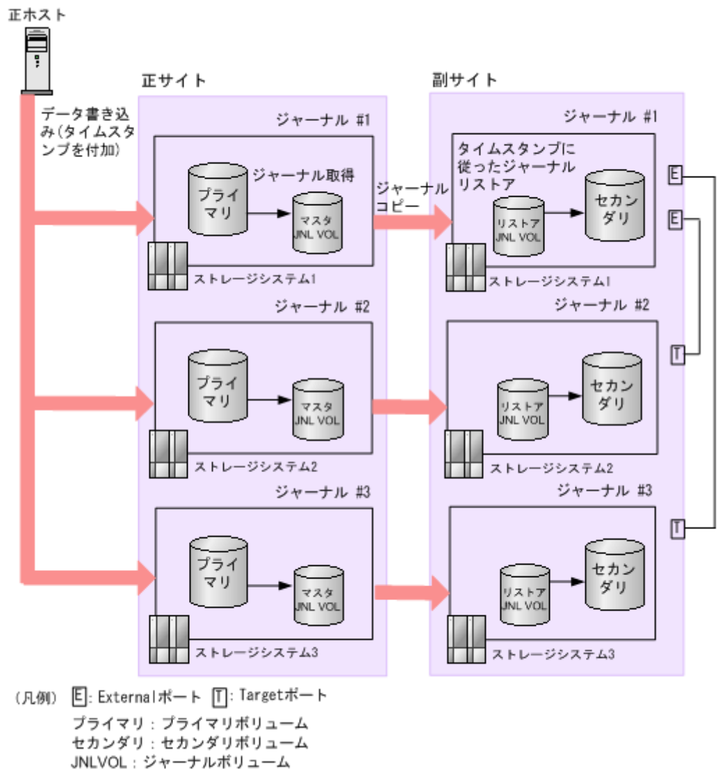
図 4 複数のストレージシステムを組み合わせた構成例
