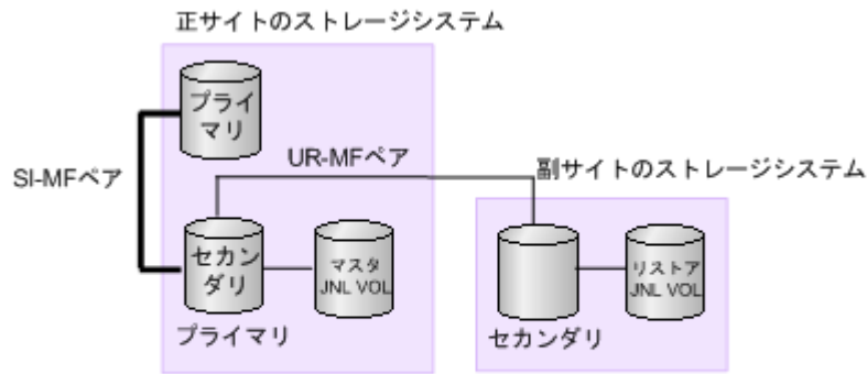
図 24 Universal Replicator for Mainframe のプライマリボリュームと ShadowImage for Mainframe のセカンダリボリューム (Split/SUSPOP 状態) を共有
