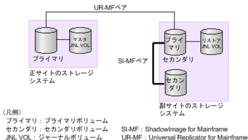
図 42 Universal Replicator for Mainframe ペアの セカンダリボリュームと ShadowImage for Mainframe ペアのプライマリボリュームを共有する構成
