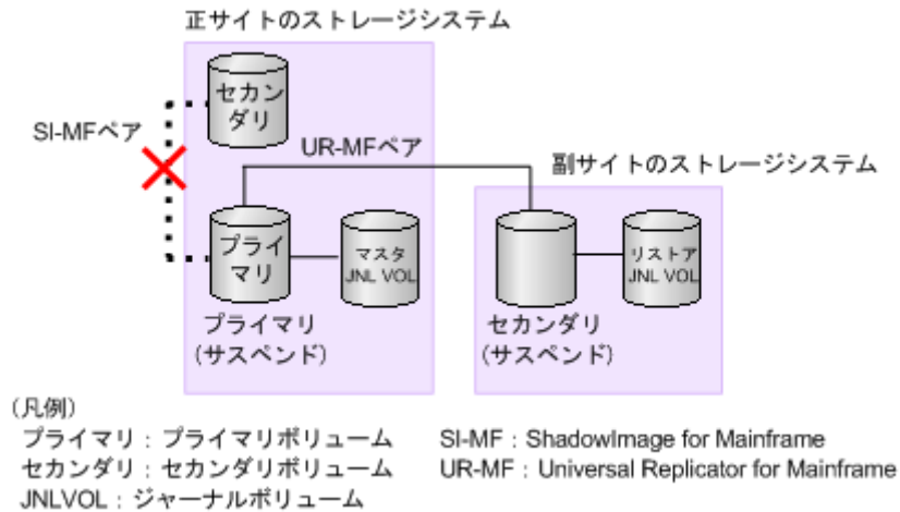
図 30 ShadowImage for Mainframe プライマリボリュームの復旧手順 (6)
