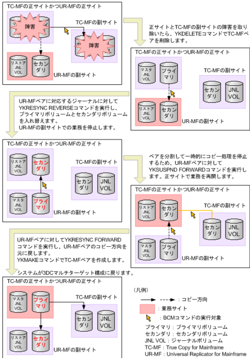
図 23 Universal Replicator for Mainframe の副サイトから正サイトに業務を戻す
