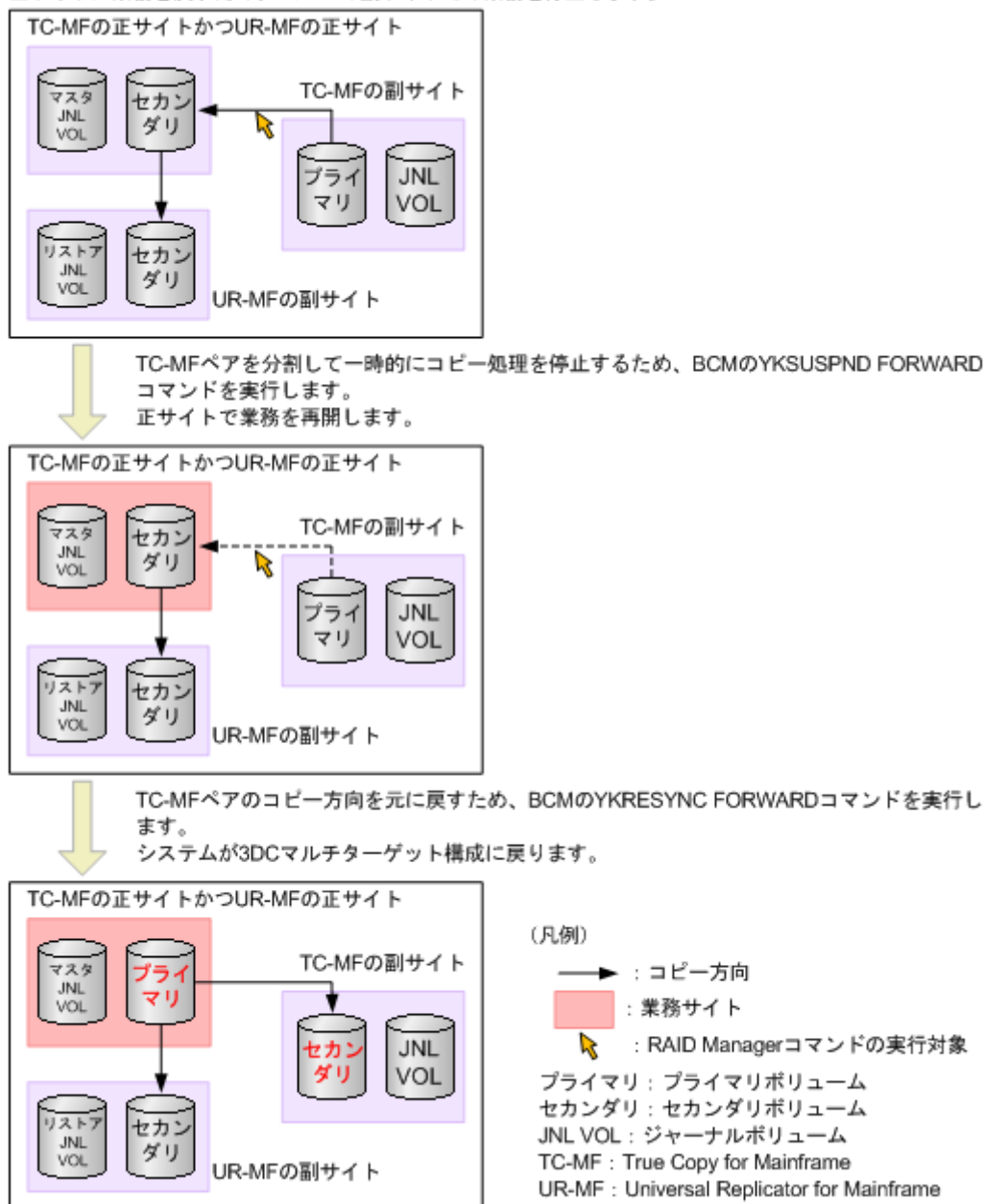
図 18 TrueCopy for Mainframe の副サイトから正サイトに業務を戻す(3DC カスケード構成から) 正サイトに業務を戻すため、TC-MFの副サイトでの業務を停止します。
