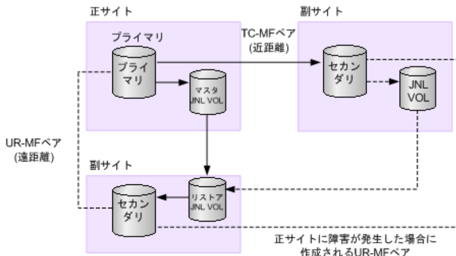
図 37 3DC マルチターゲット
