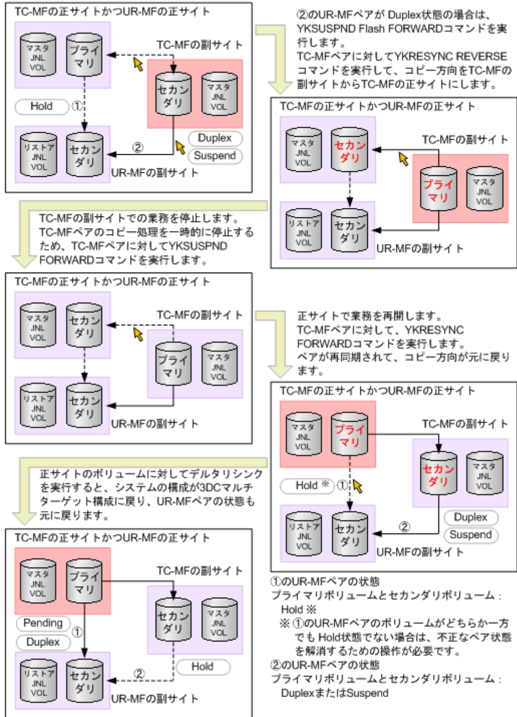
図 21 TrueCopy for Mainframe の副サイトから正サイトに業務を戻す (3DC マルチターゲット構成、デルタリシンク処理を実行した場合)
