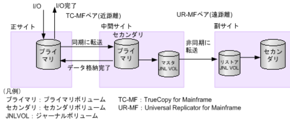
図 36 3DC カスケード構成
