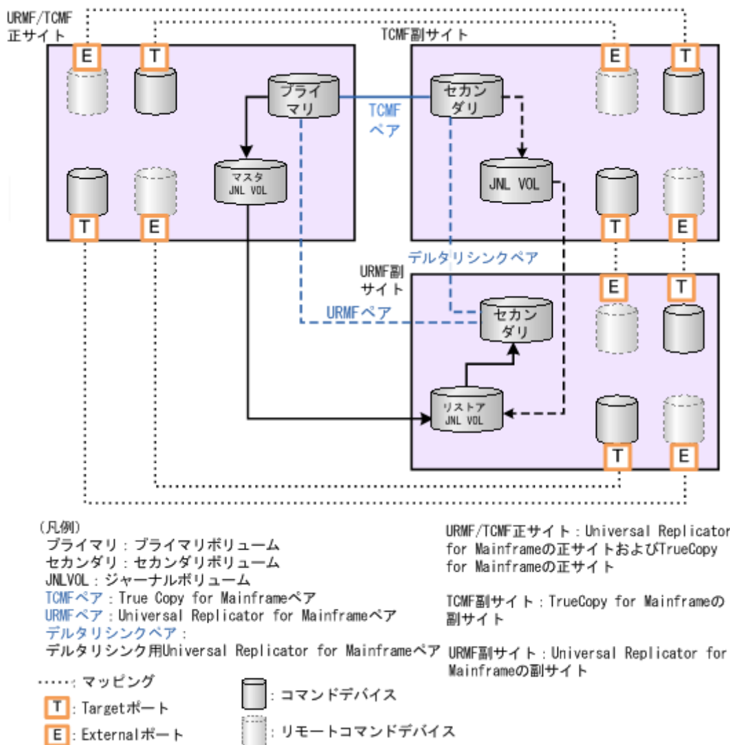
図 38 デルタリシンクに対応した 3DC マルチターゲット構成
