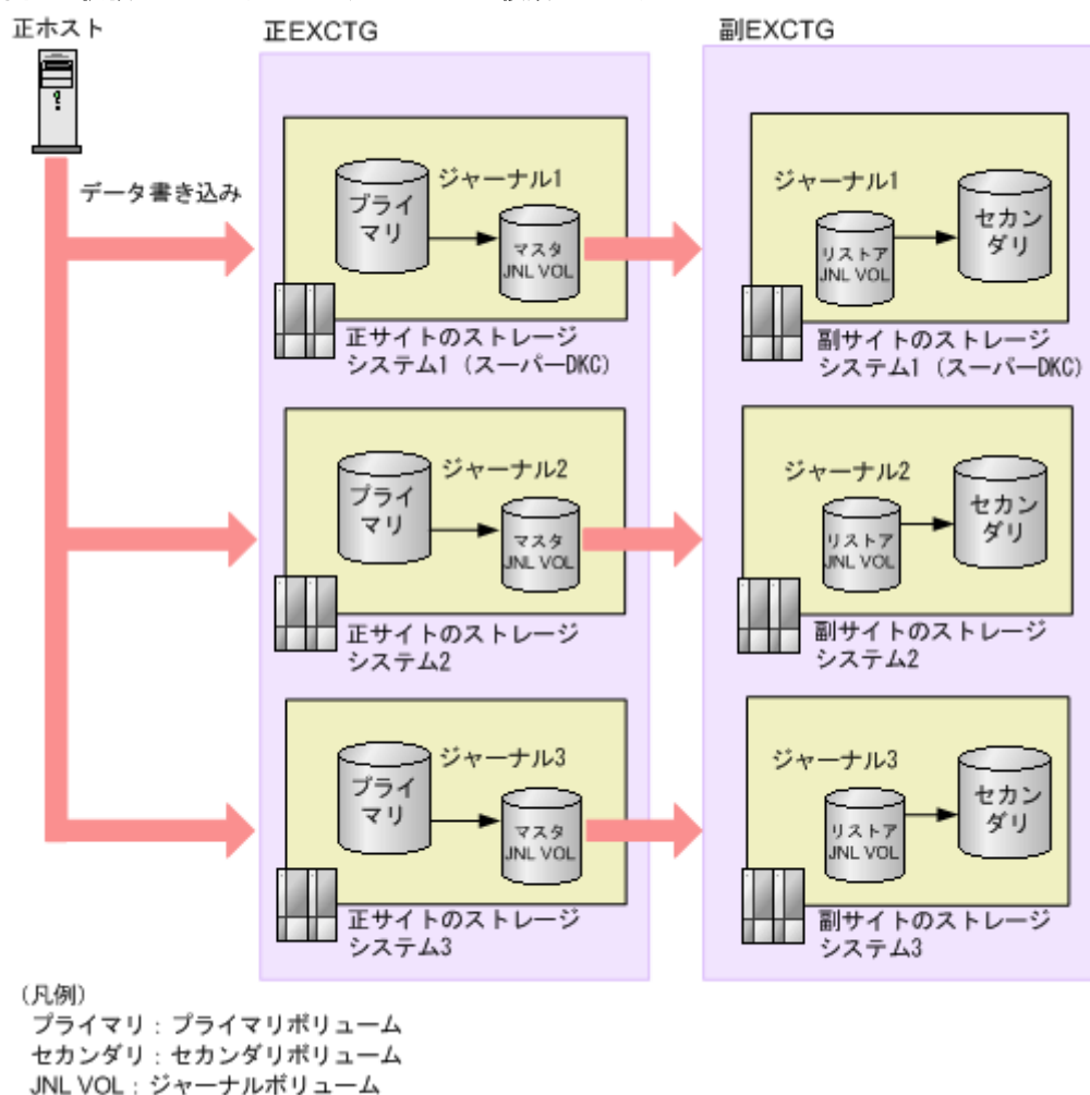
図 14 拡張コンシステンシーグループ内の複数のシステム
