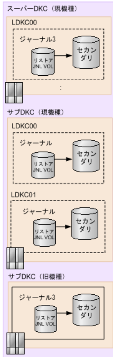
図 15 VSP G1000, VSP G1500, VSP F1500 または VSP を副サイトのストレージシステムのサブDKC に設定できる構成例
