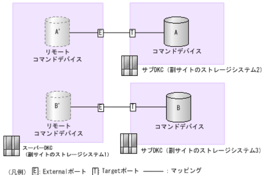
図 5 複数の副サイトのストレージシステムを組み合わせた構成例
