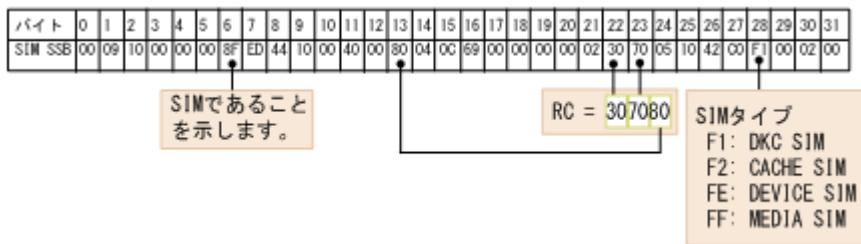
図 34 代表的な SIM と参照コードおよび SIM タイプ
