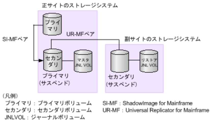
図 31 ShadowImage for Mainframe プライマリボリュームの復旧手順 (7)
