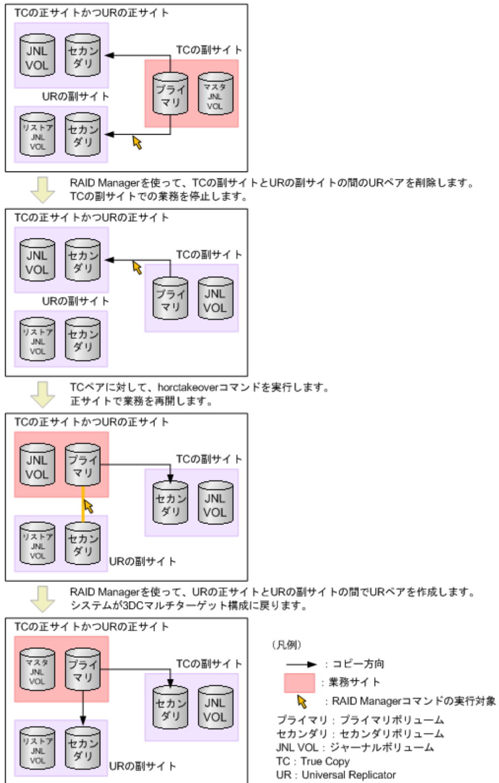
図 23 TrueCopy の副サイトから正サイトに業務を戻す (3DC マルチターゲット構成から) 暫定的に、TCの副サイトを業務サイトにした3DCマルチターゲット構成になっています。
