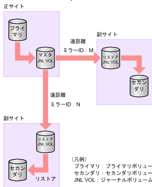
図 4 3つの Universal Replicator サイトによる 3DC マルチターゲット構成
