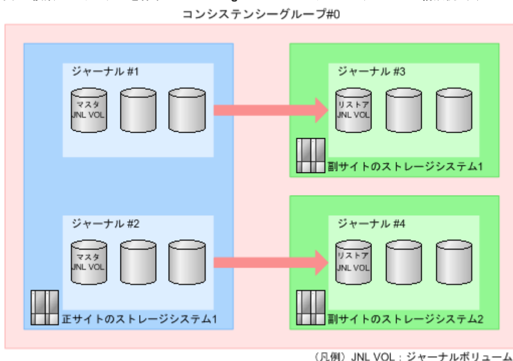
図 9 複数のジャーナルを伴う RAID Manager のコンシステンシーグループの構成例 (1)
