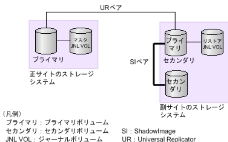
図 50 Universal Replicator ペアの セカンダリボリュームと ShadowImage ペアのプライマリボリュームを共有する構成
