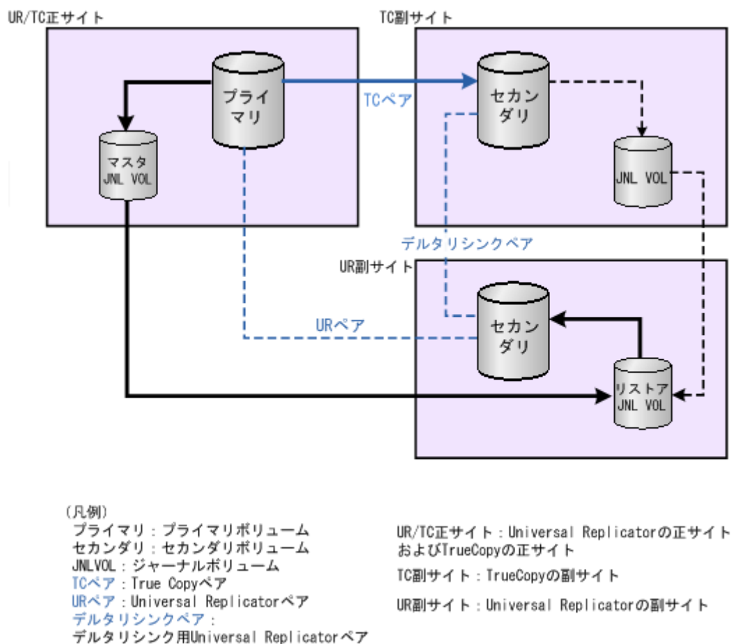
図 47 デルタリシンク用 3DC マルチターゲット構成
