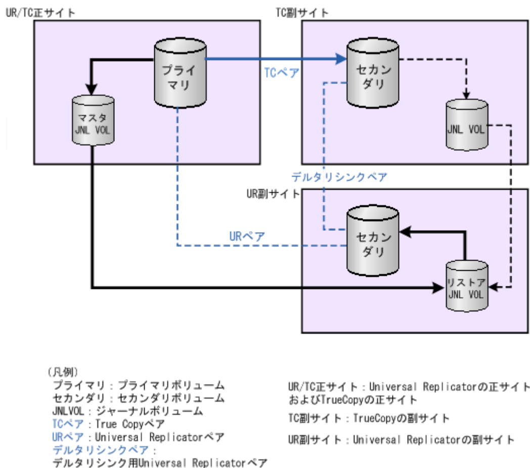
図 47 デルタリシンク用 3DC マルチターゲット構成
