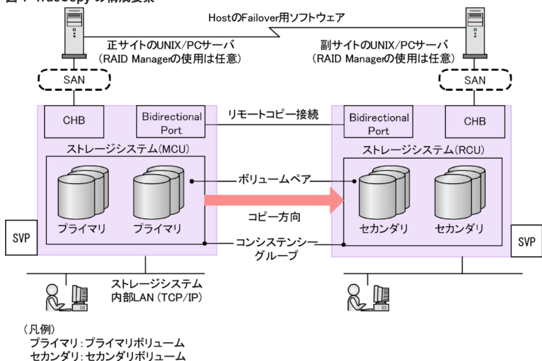
図 1 TrueCopy の構成要素
